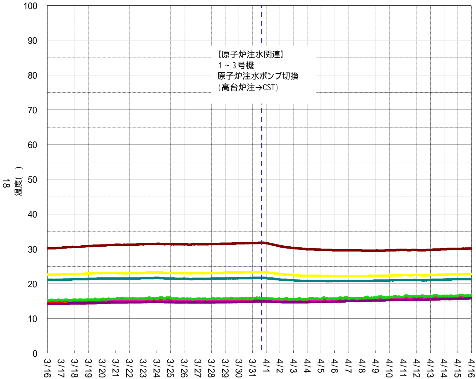
1号機 実施計画関連温度計(PCV)
