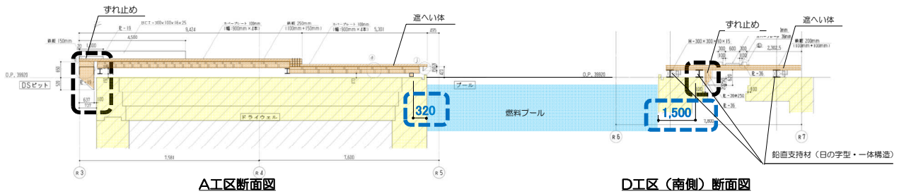
(b) プール周りの南北断面
