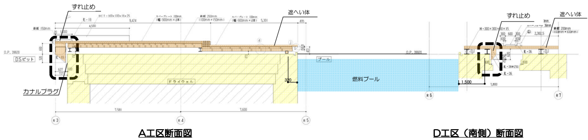
(b) プール周りの南北断面
