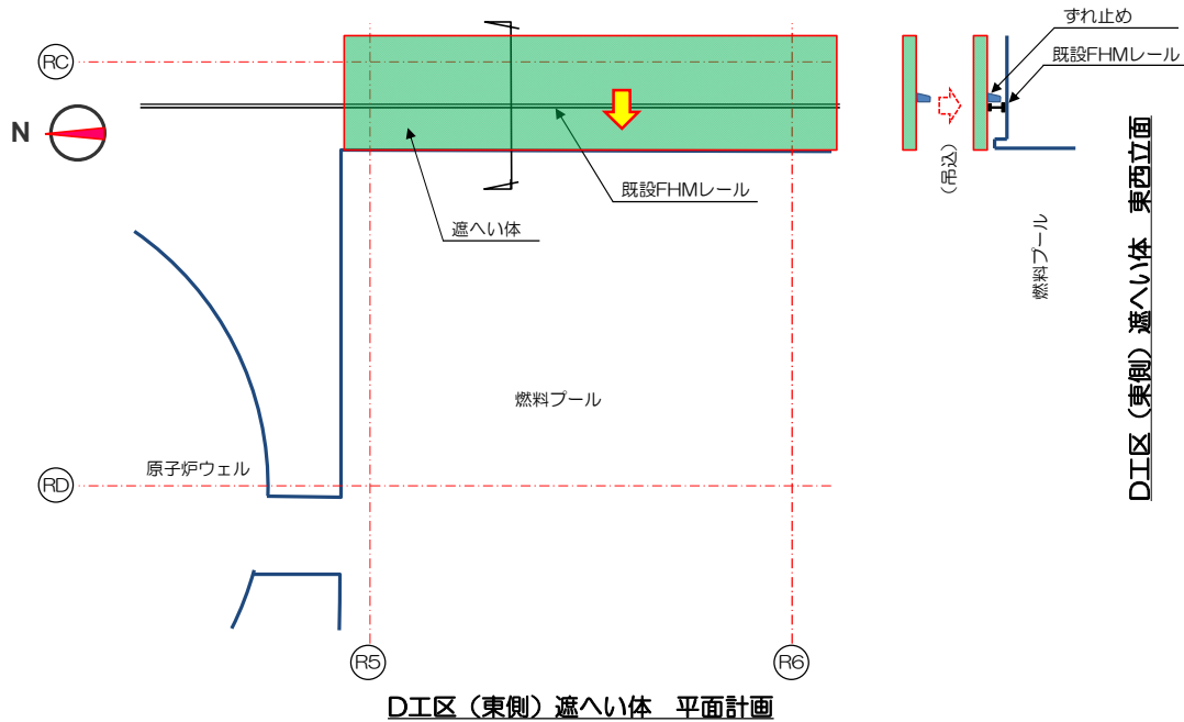
(c) プール際D工区 (東側) 遮へい体
