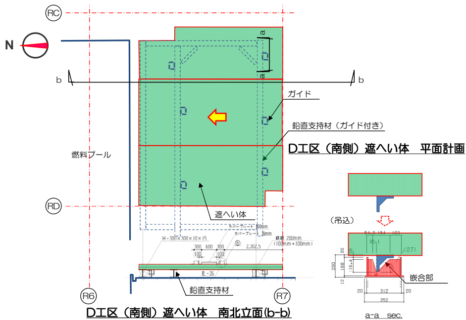
(d) プール際D工区 (南側) 遮へい体
