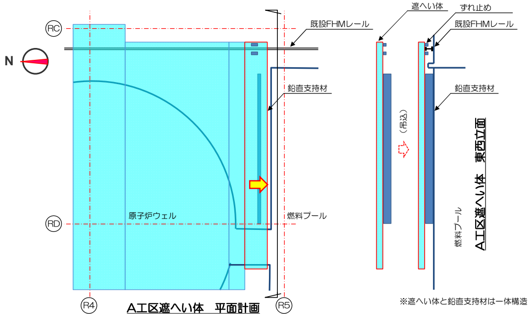
(a) プール際 A 工区遮へい体
