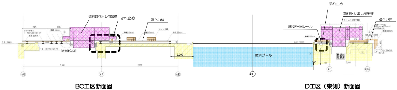
(c) プール周りの東西断面
