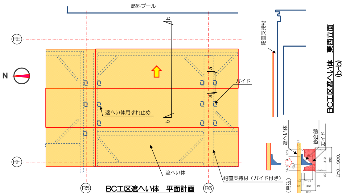
(b) プール際 BC 工区遮へい体
