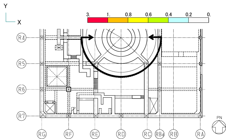
図-3.5.8 面外せん断力の検定比（シェル壁部）
