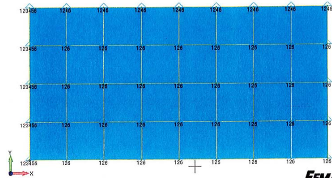
図 5.2.2-2 片持ち平板の解析モデル
