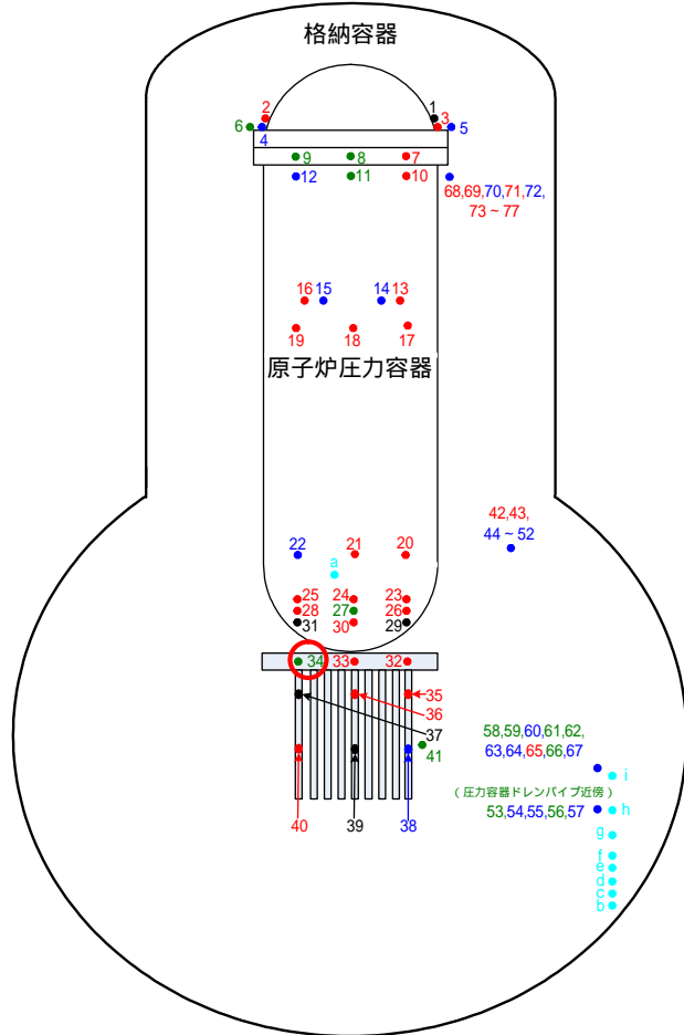
<平面図>
