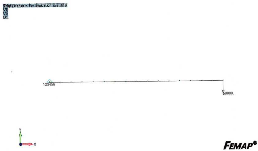
図 5.2.2-3 片持ち梁の解析モデル
