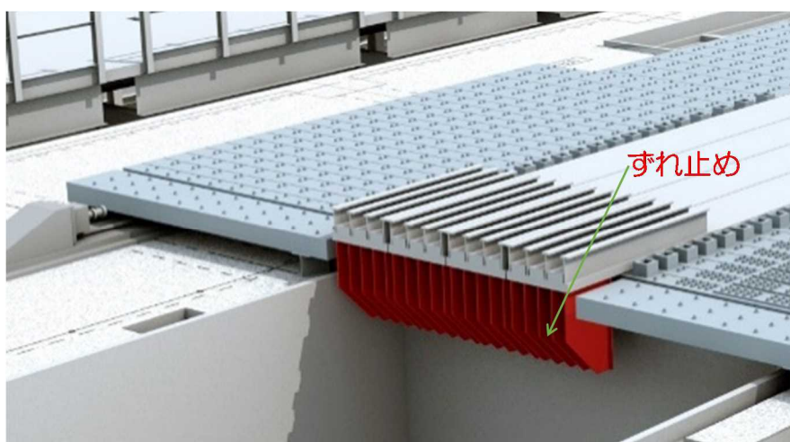
図 2.1-1 ずれ止めの概要 (A 工区)
