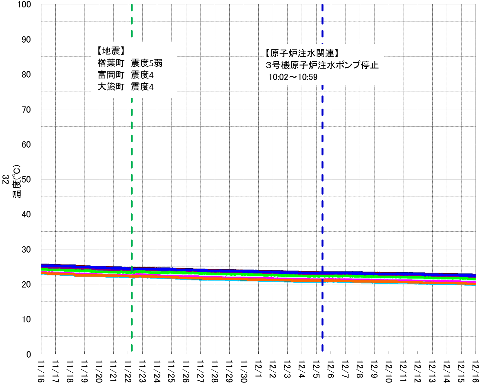
3号機 RPV周辺温度計(下部)
