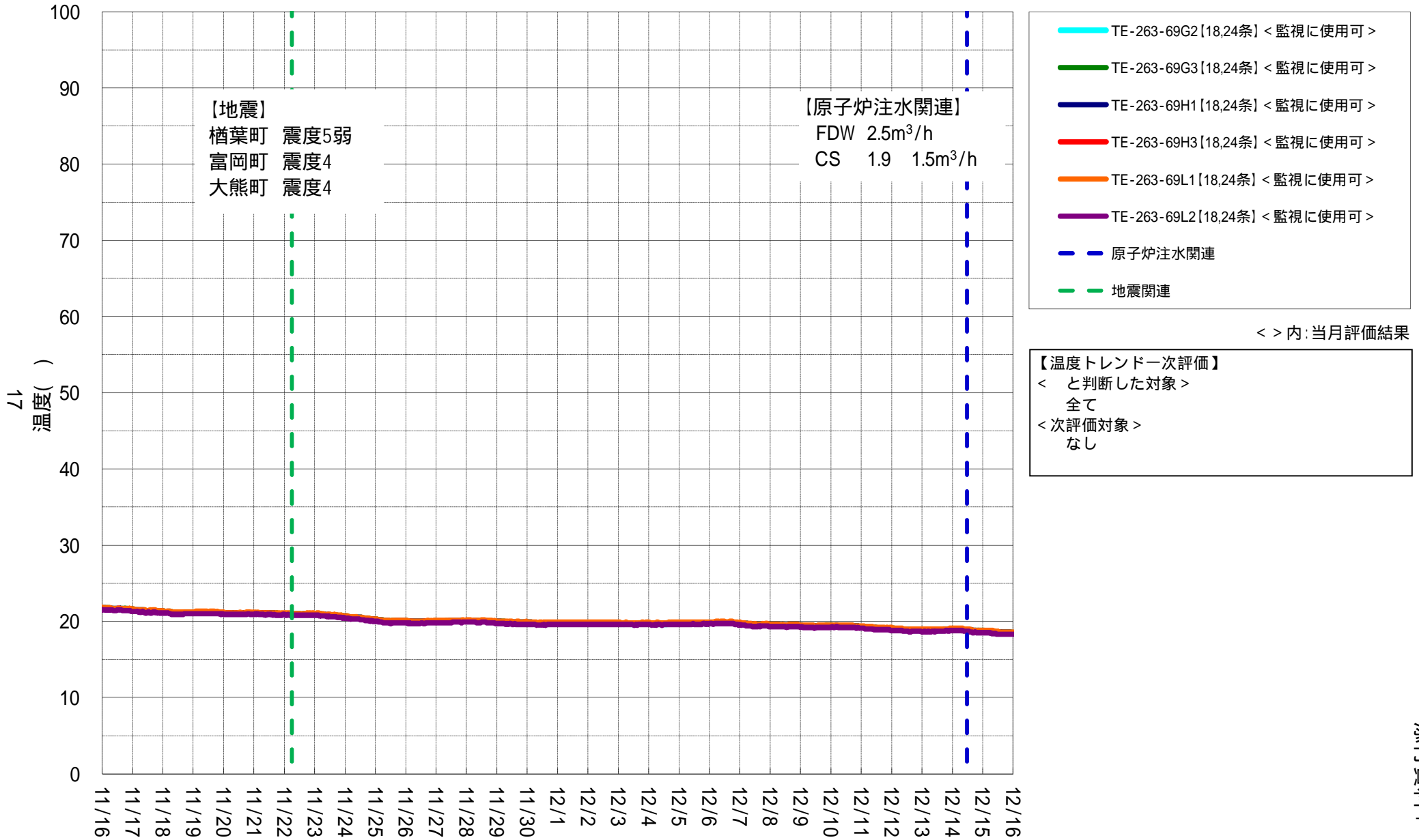
1号機 実施計画関連温度計 (RPV)
