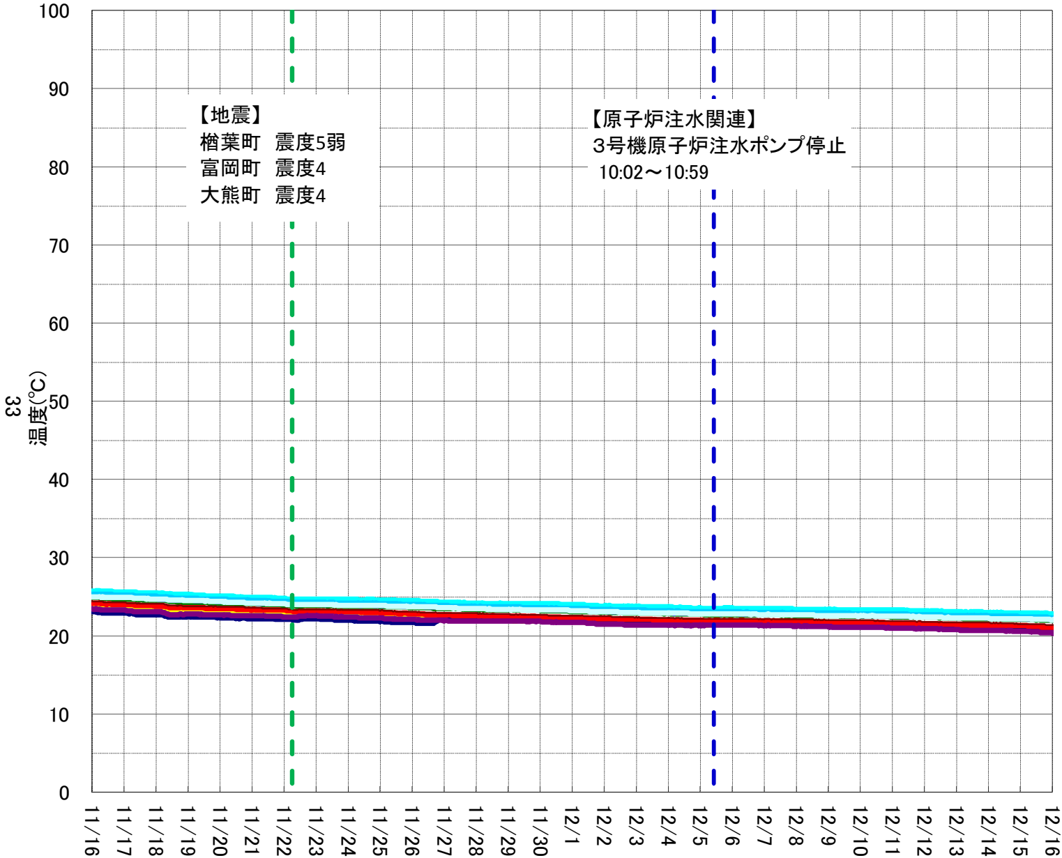
3号機 PCV内温度計①
