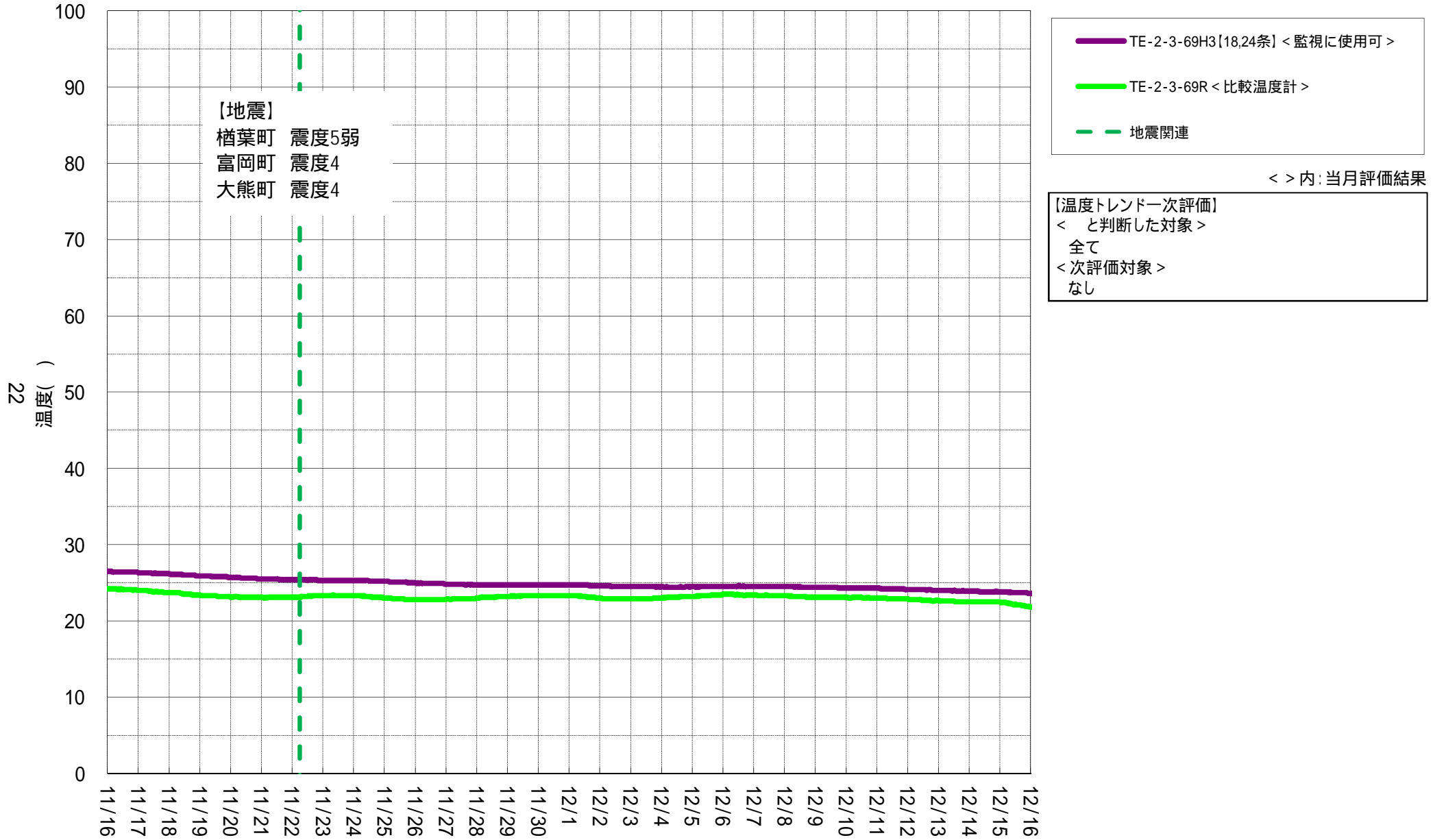
2号機 実施計画関連温度計(RPV)
