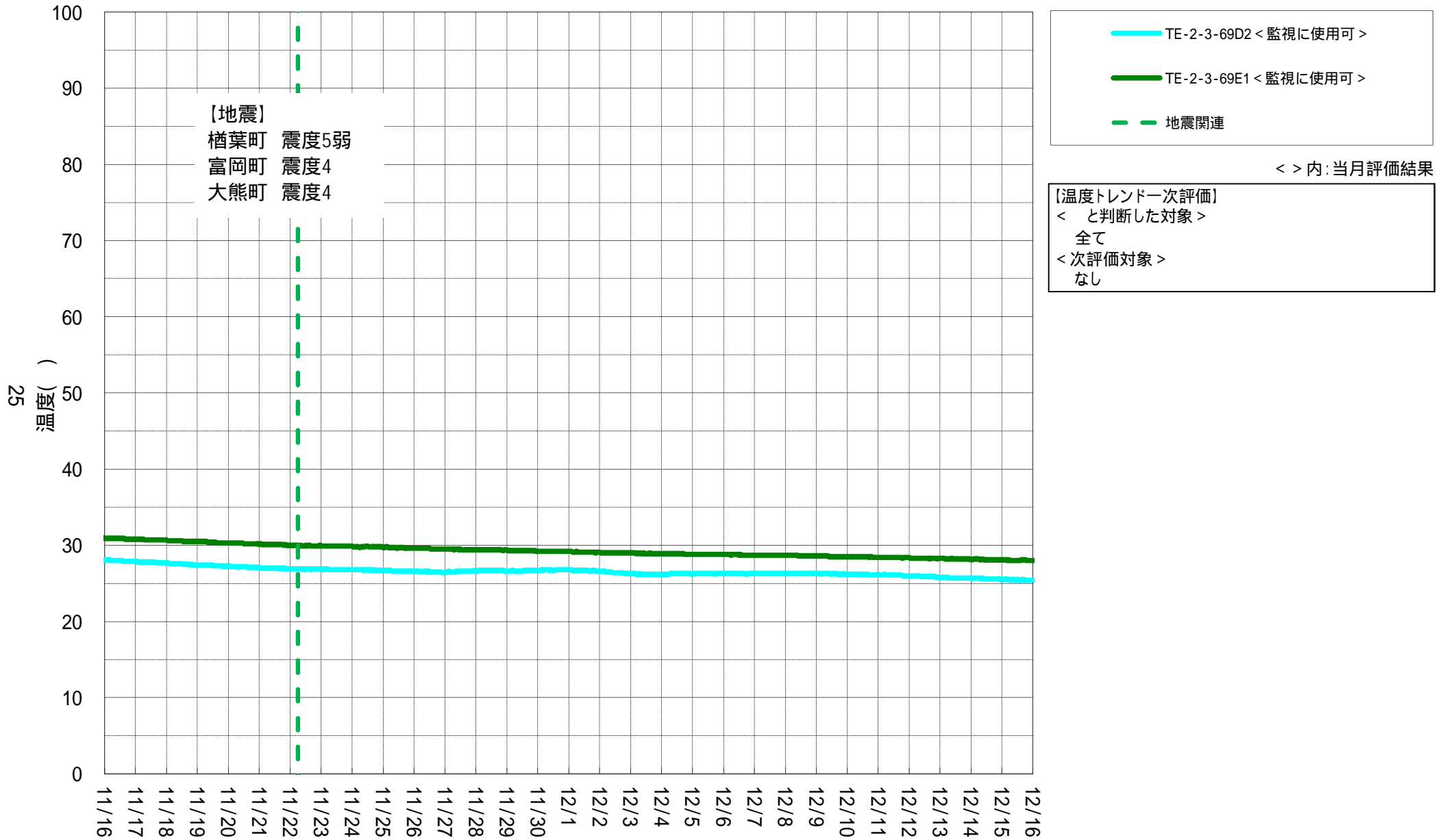
2号機 RPV周辺温度計(上部)
