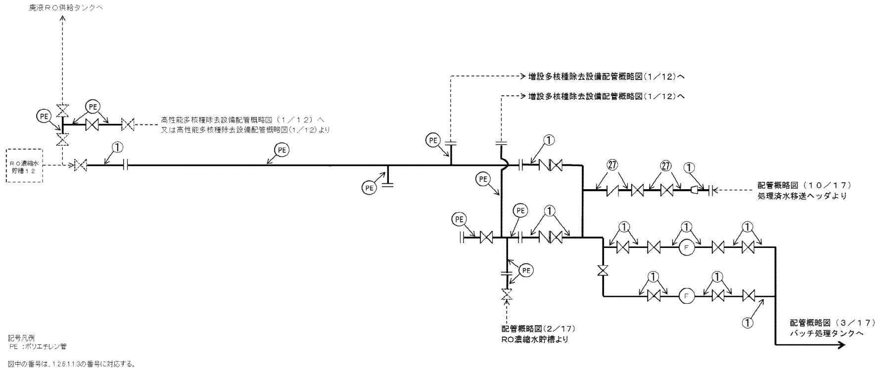
図一 配管概略図 (1 / 17)
