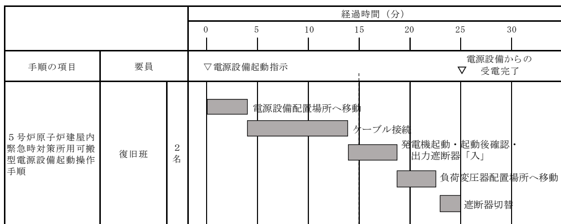
図 3.2-8 5号炉原子炉建屋内緊急時対策所用可搬型電源設備立ち上げのタイムチャート
