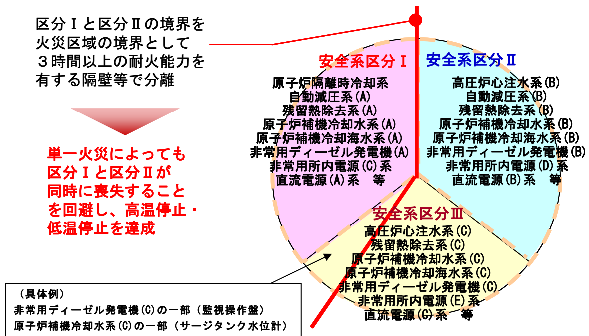
図7-1：3時間耐火能力を有する隔壁等による系統分離の概要
