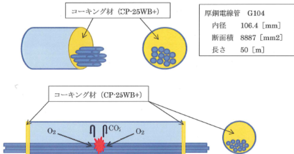
図 2 : 電線管外部からの酸素供給防止を目的としたシール処理
