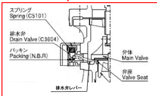
図 1-25：不凍式消火栓の構造の概要
