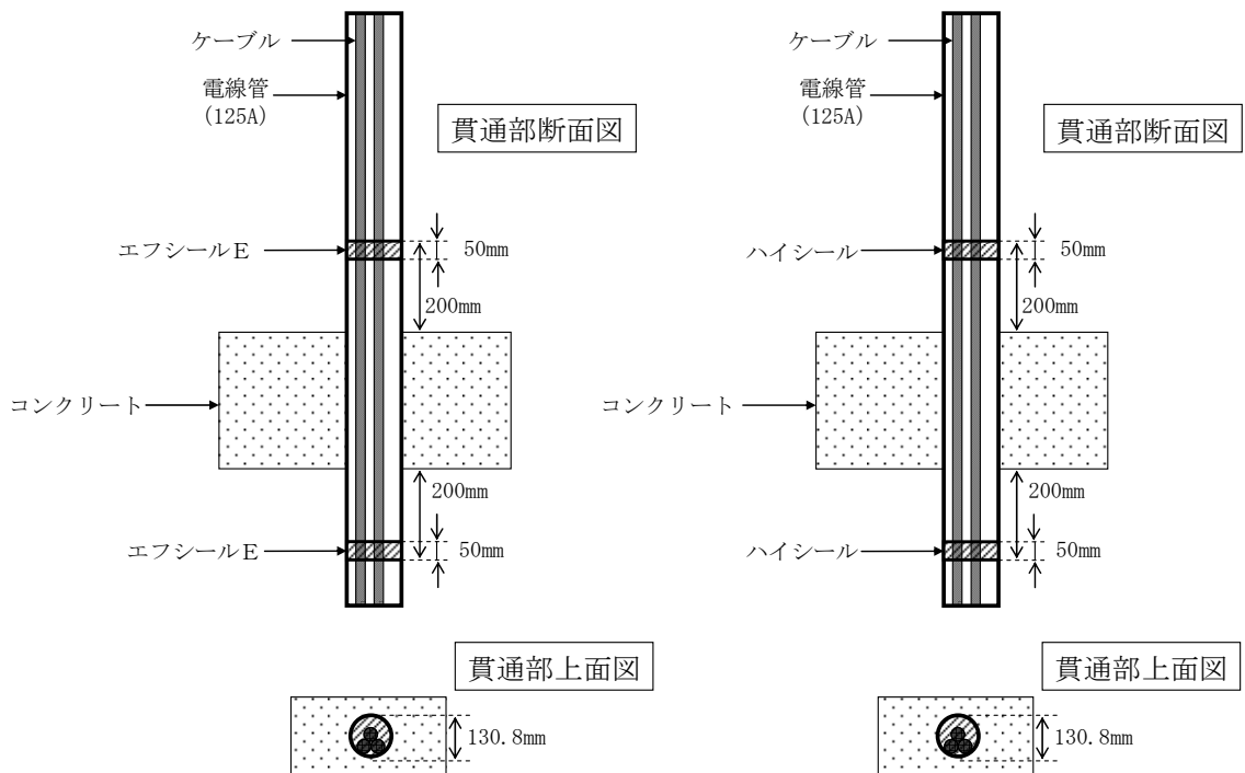
(c) 6号炉電線管貫通部
