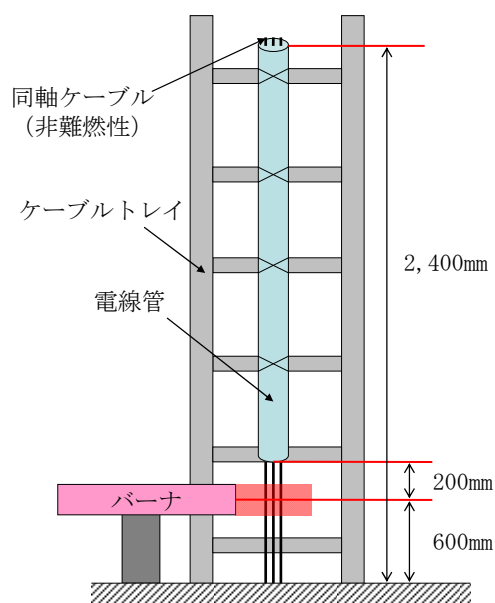
図1：電線管収納状態での IEEE 383 std 1974 垂直トレイ燃焼試験の概要
