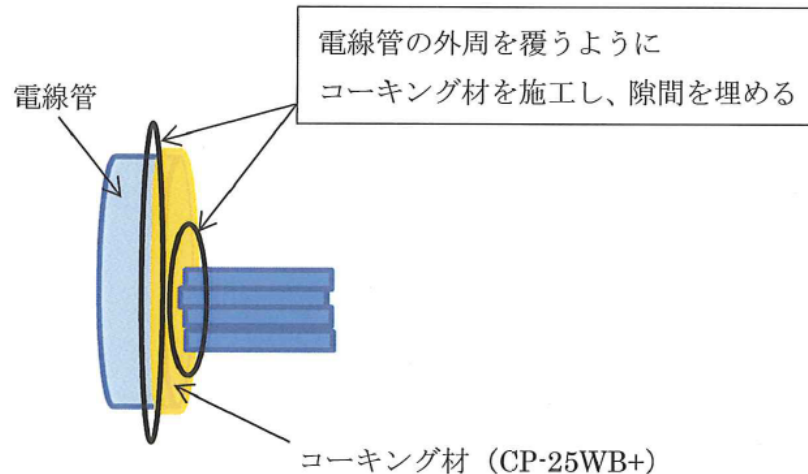
図4. コーキング材（CP-25WB+）の施工方法
