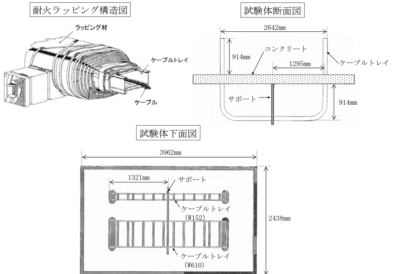
図 6 耐火ラッピング試験体の構造
