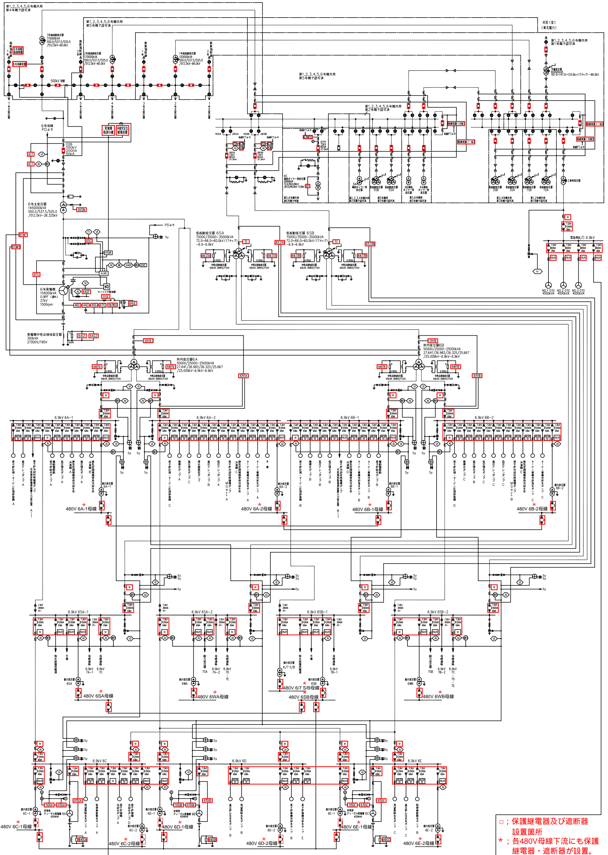
図1-7：6号炉 電気系統保護継電器及び遮断器の設置箇所
