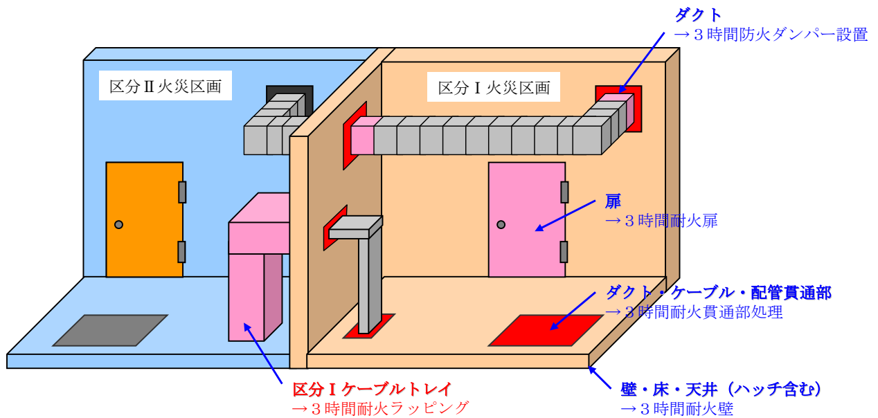
図2：火災の影響軽減対策とケーブルラッピング
