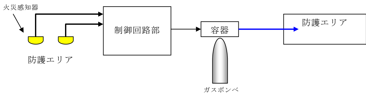
図5：全域ガス消火設備起動ロジック
