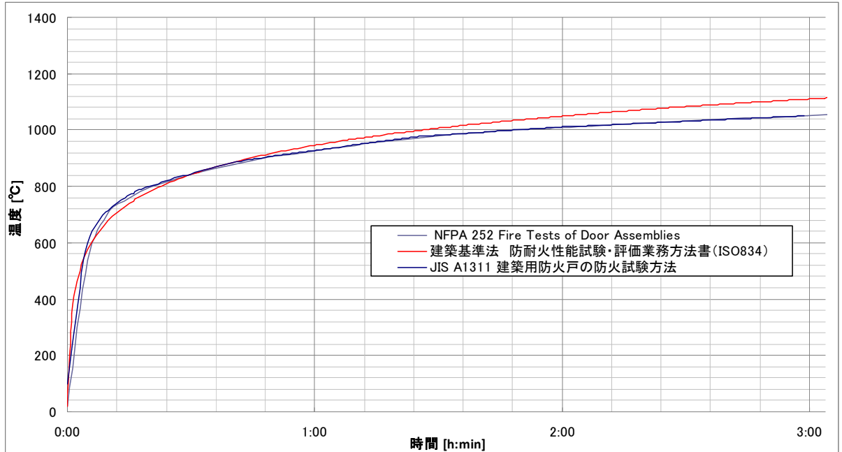
図2 加熱曲線の比較
