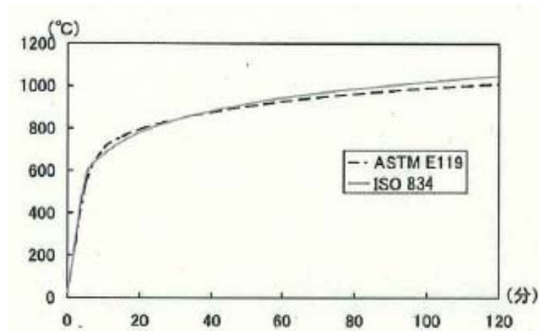
図 5 加熱曲線の比較 (出典：加熱炉特性の試験所間比較試験報告 (2009))
