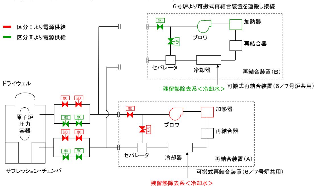
※本図は7号炉に再結合装置(A)を接続している場合の例を示す
