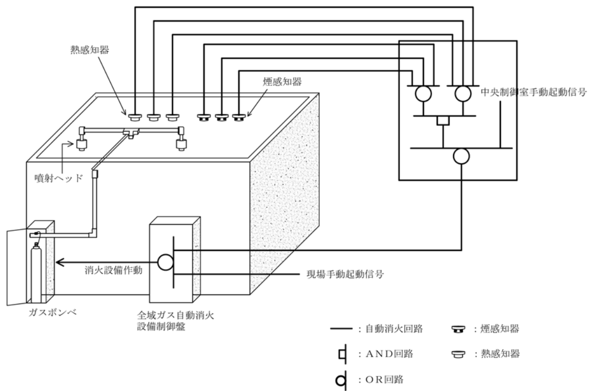
図 1-14 : 全城ガス消火設備の概要
