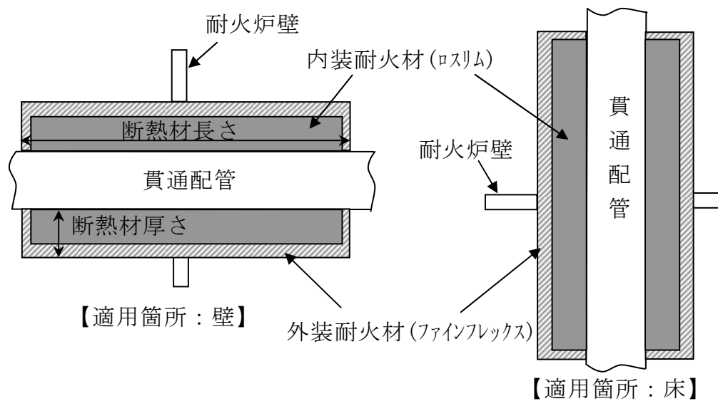
図3 耐火材取付部の耐火試験体
