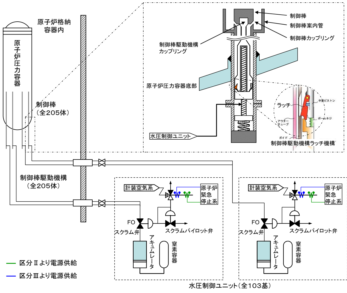
図 2-2 : 制御棒及び制御棒駆動系 (水圧制御ユニット) の系統概略図
