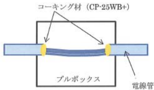
図 3 : プルボックスの火災発生防止処理
