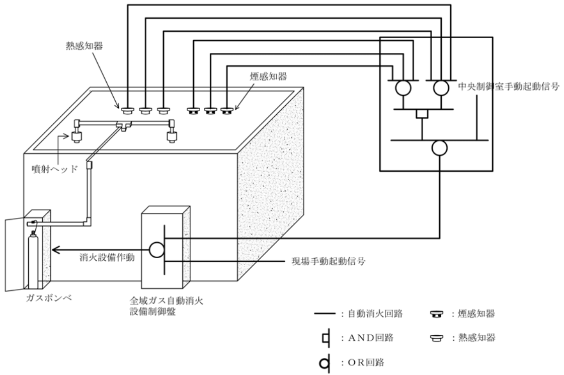
図 1 : 全域ガス消火設備の動作概要図
