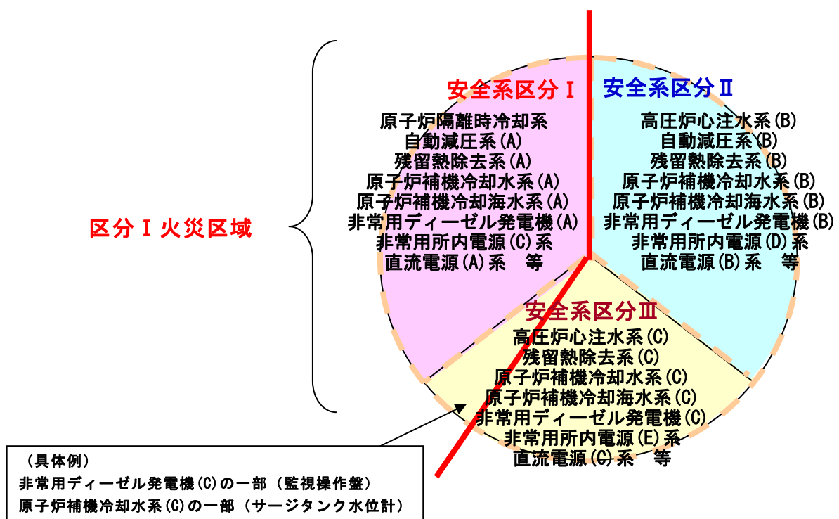
図1：系統分離の概要
