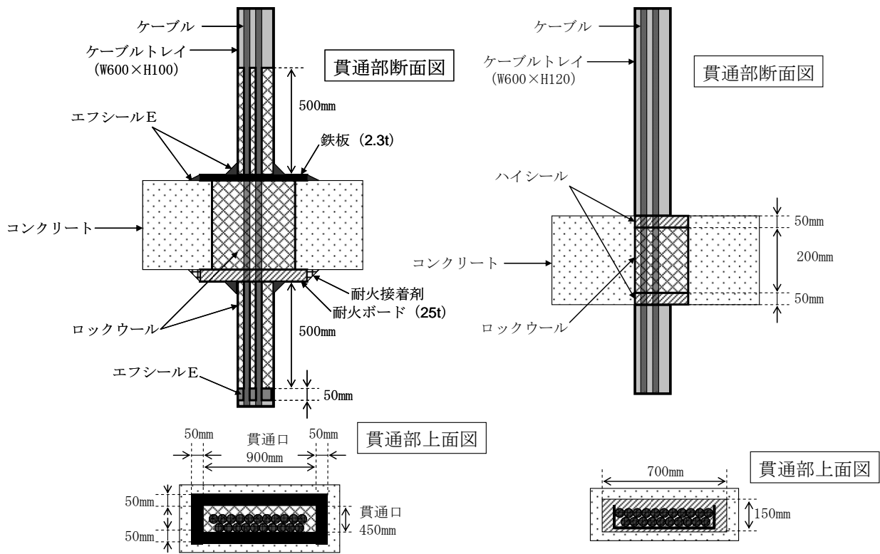
(a) 6号炉ケーブルトレイ貫通部
