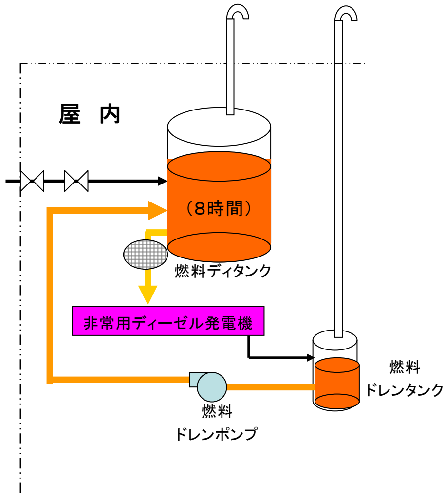
図 1-29 : 油タンクのベント管設置の概要
