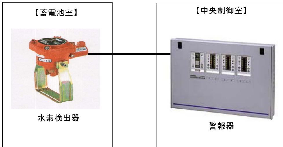
図 1-4 : 蓄電池室水素検出器の概要
