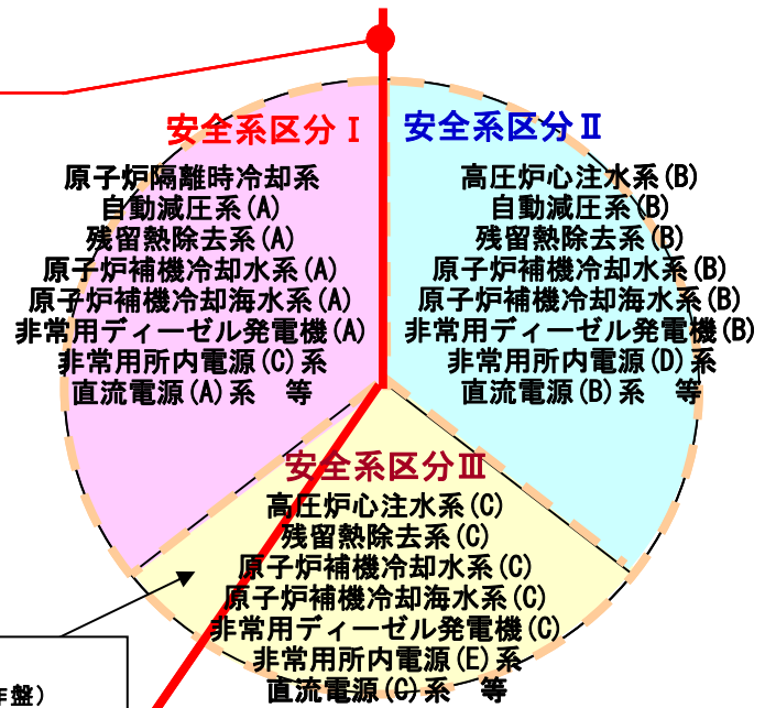
図 1-28 : 3 時間耐火能力を有する隔壁等による系統分離の概要
