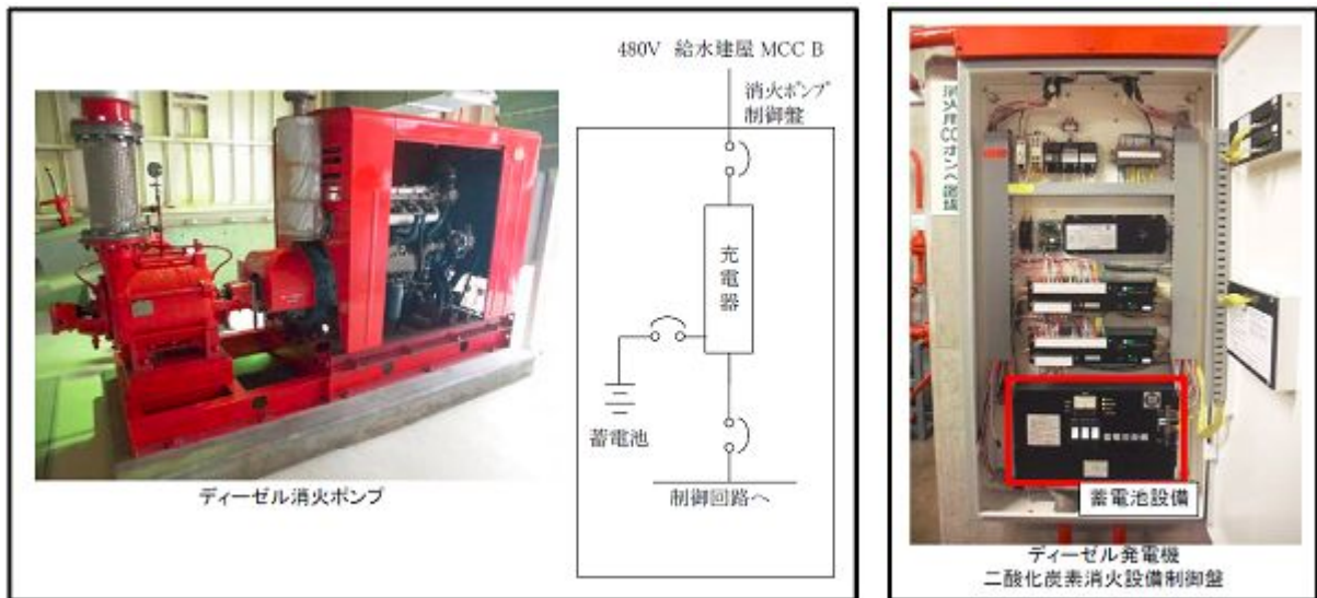
図 1-19：消火設備の電源確保の概要
