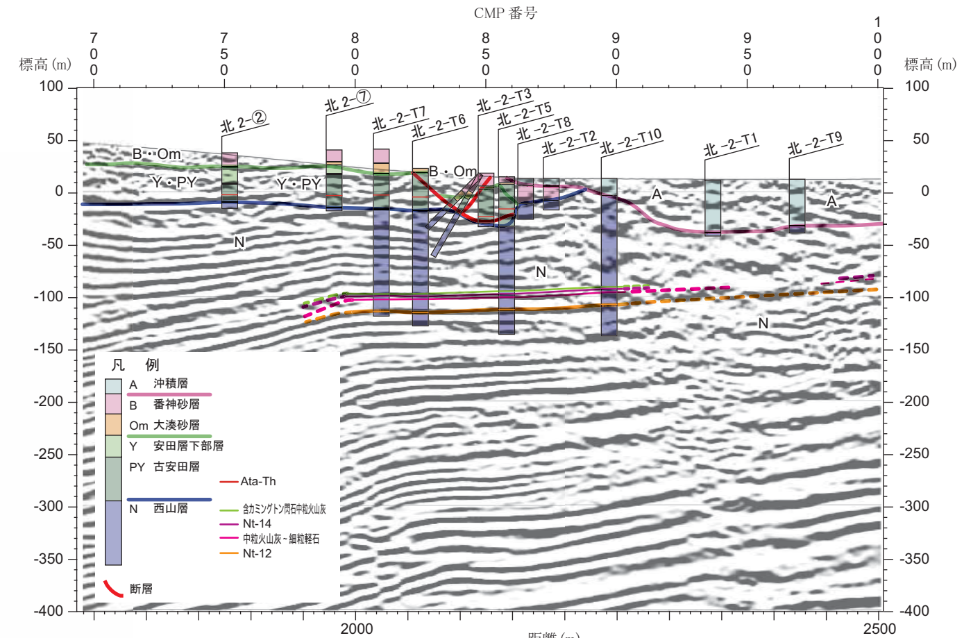
西元寺周辺の北-2測線深度断面図及び解釈図
