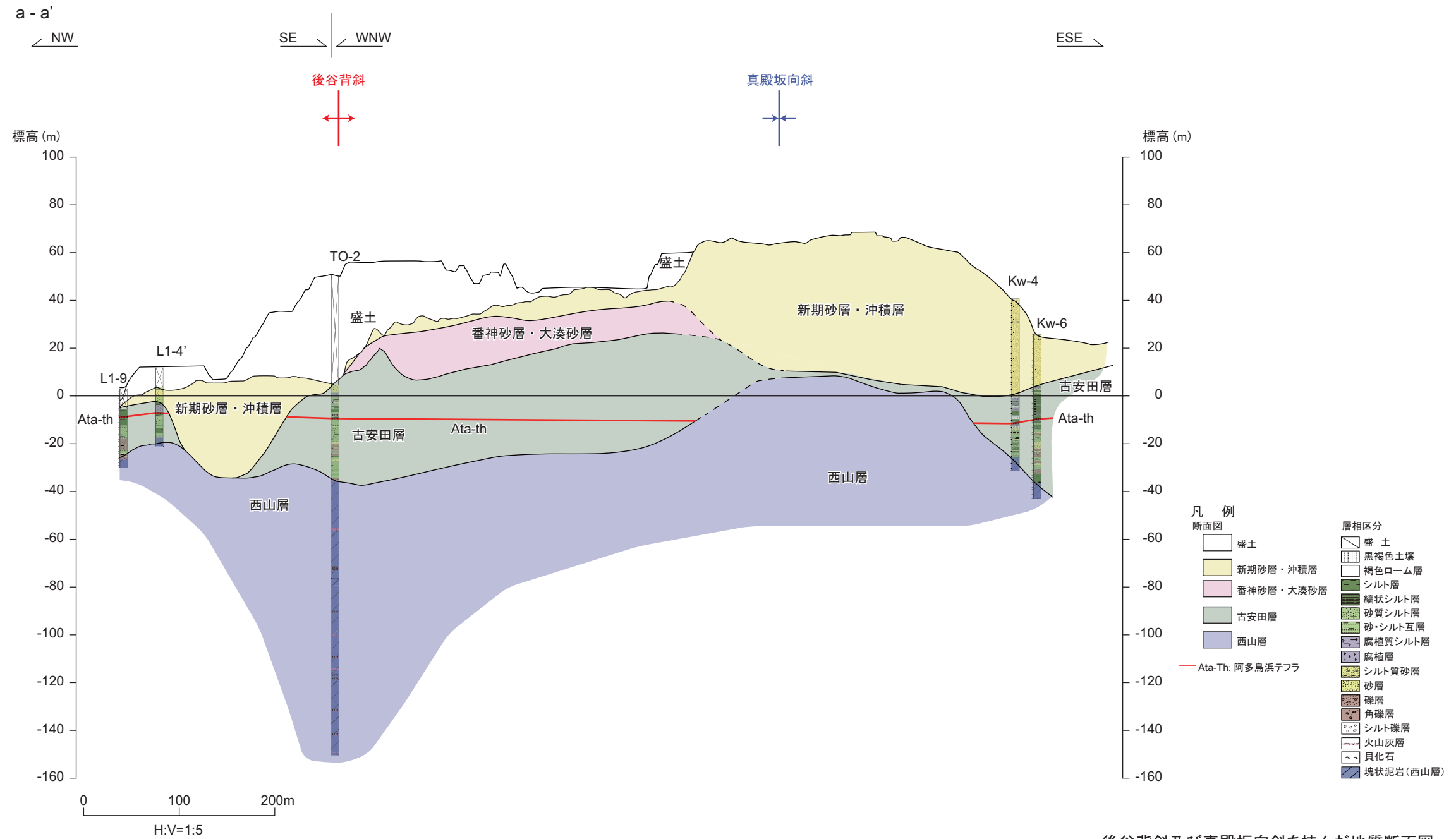
後谷背斜及び真殿坂向斜を挟んだ地質断面図
