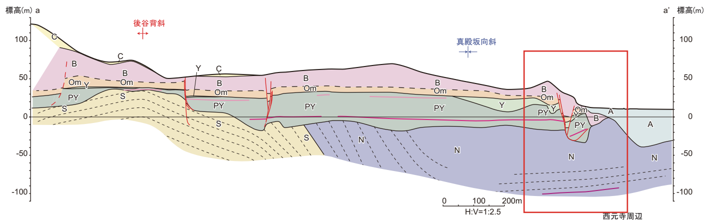
西元寺周辺の地質断面図
