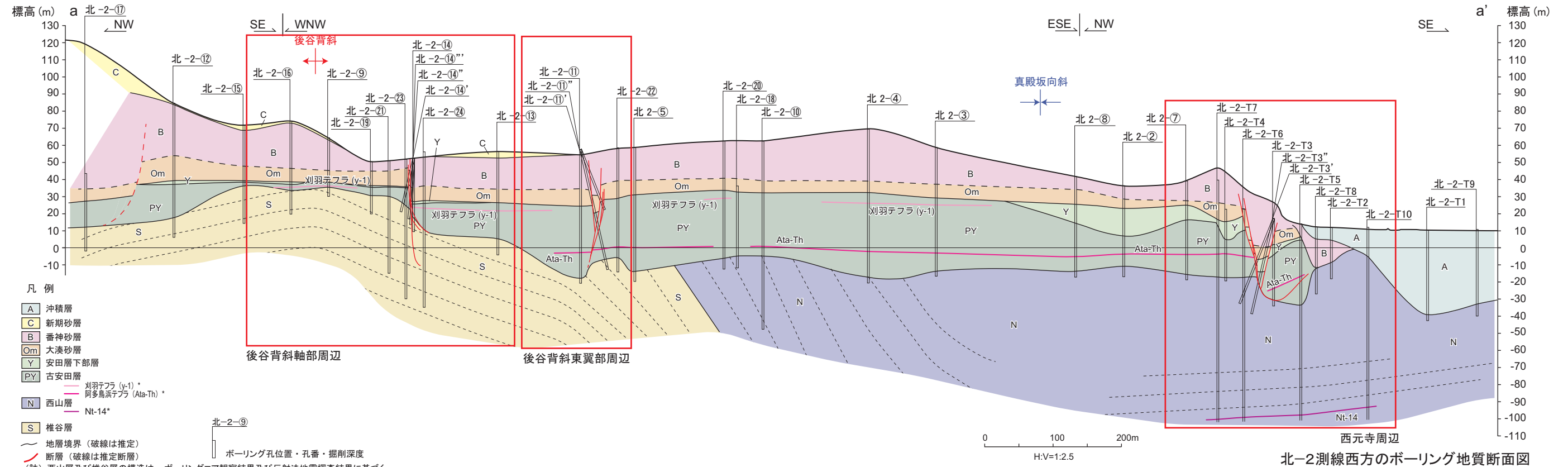
北-2測線西方のボーリング地質断面図
