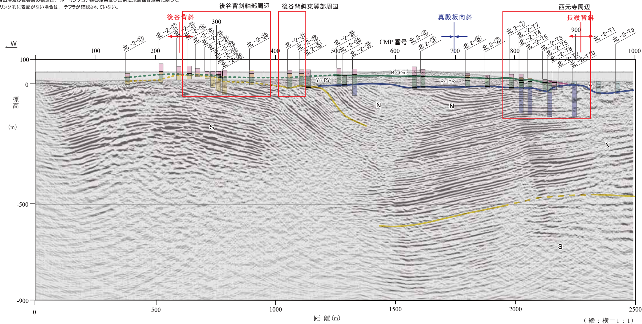
北-2測線の深度断面図・解釈図
