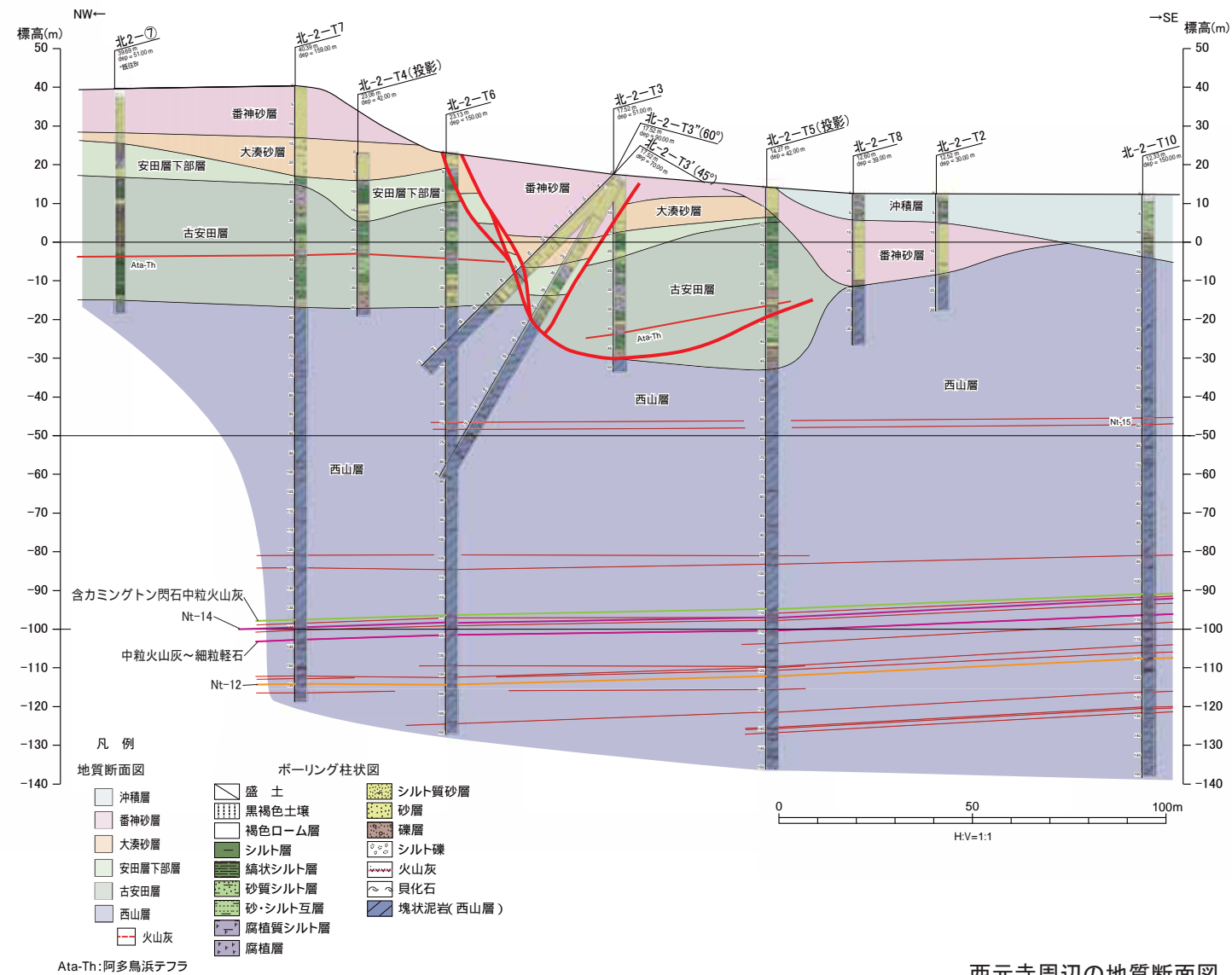
西元寺周辺の地質断面図
