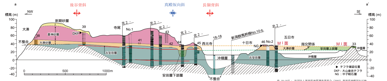
後谷背斜~長嶺背斜周辺のボーリング調査結果
