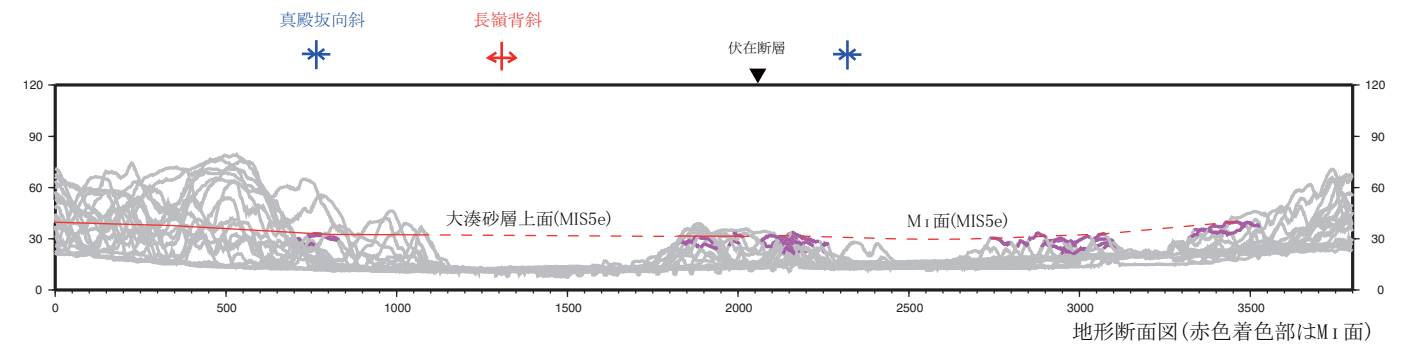
柏崎平野北部における下末吉離水面の標高分布
