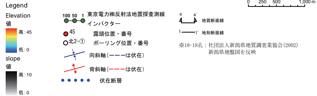
柏崎平野北部の標高段彩陰影図
