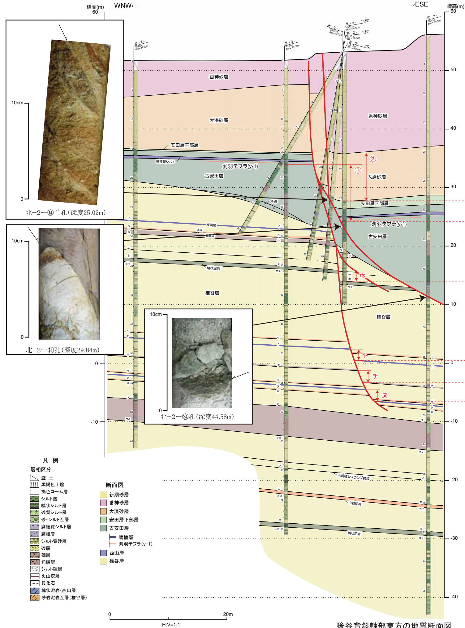
後谷背斜軸部東方の地質断面図
