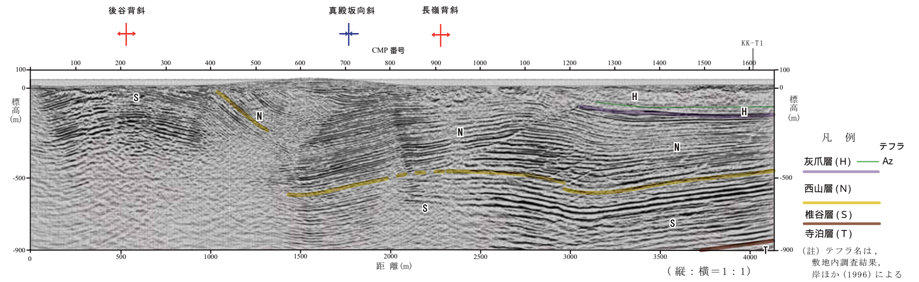
北-2測線の深度断面図及び解釈図
