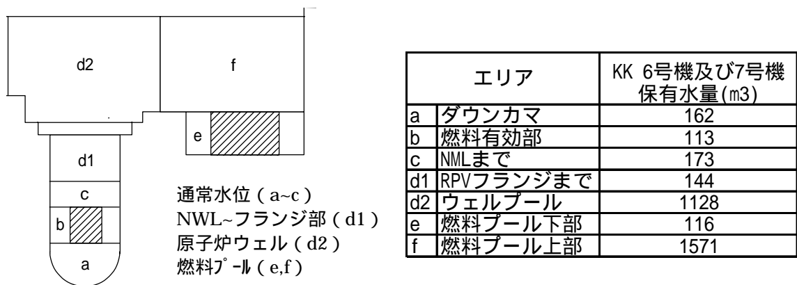
図 3.1.2.c-3 保有水のエリア分割図と保有水量
