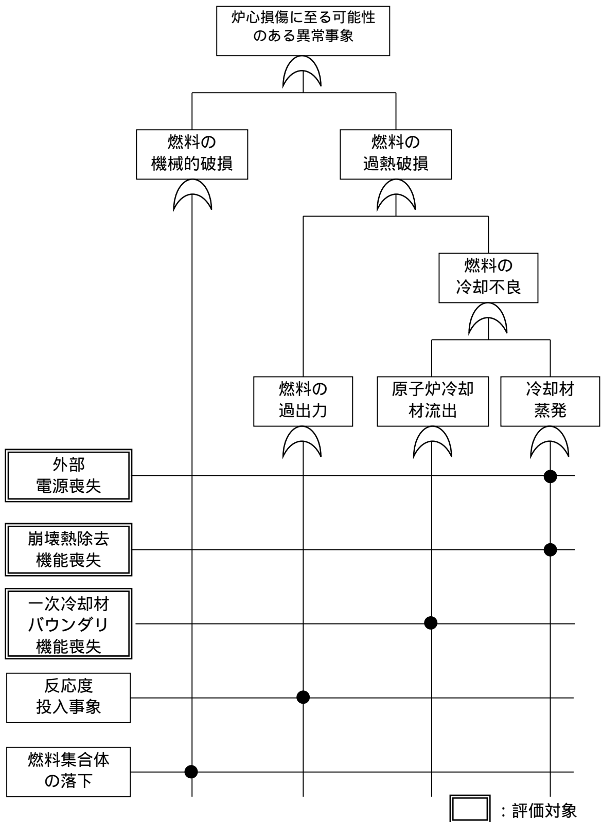
図3.1.2.b-1 炉心損傷に至る可能性のある異常事象マスターロジックダイヤグラム
