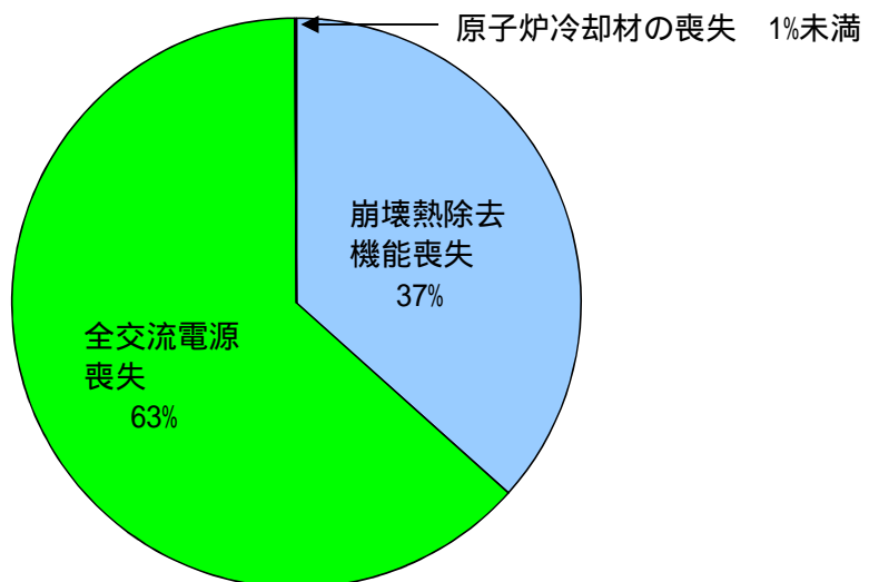
図 3.1.2.h-9 事故シーケンスグループ別の炉心損傷頻度の割合(感度解析)
