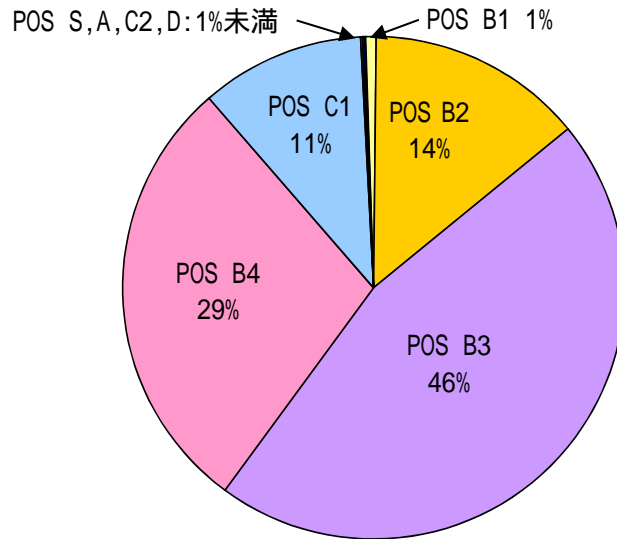
図 3.1.2.h-7 POS 別の炉心損傷頻度の割合(感度解析)
