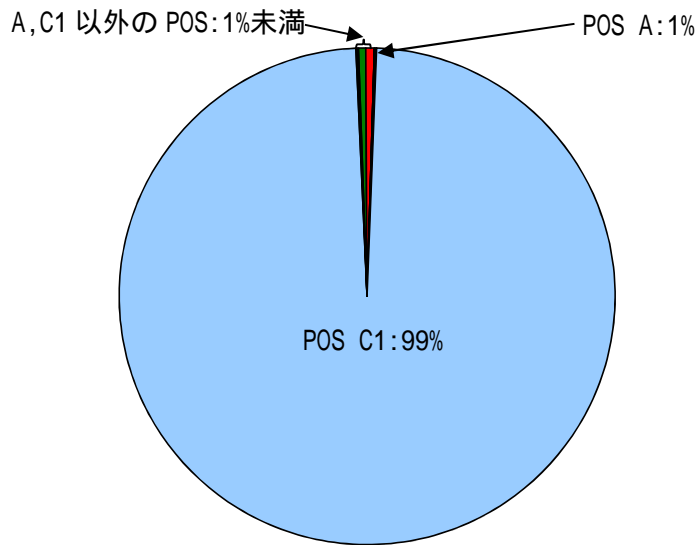
図 3.1.2.h-1 POS 別の炉心損傷頻度の割合
