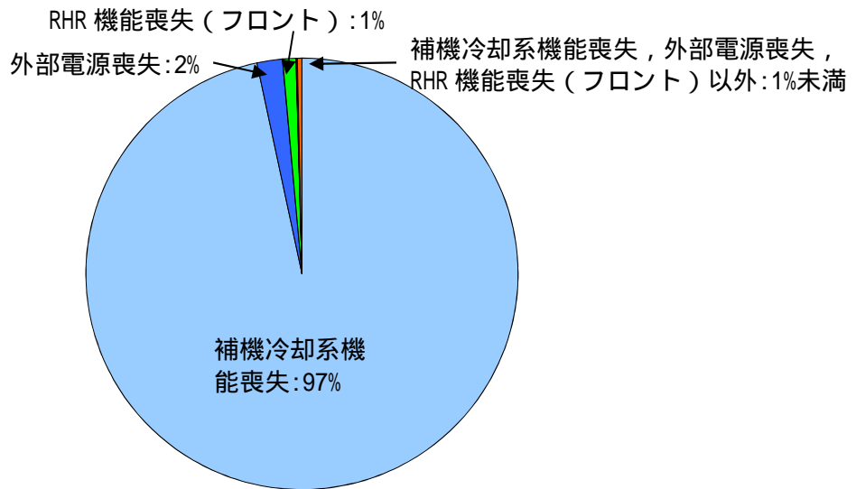
図 3.1.2.h-2 起因事象別の炉心損傷頻度の割合
