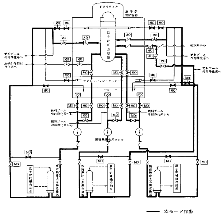
図3.1.2.a-1 残留熱除去系停止時冷却モード(SHC)の概要図
