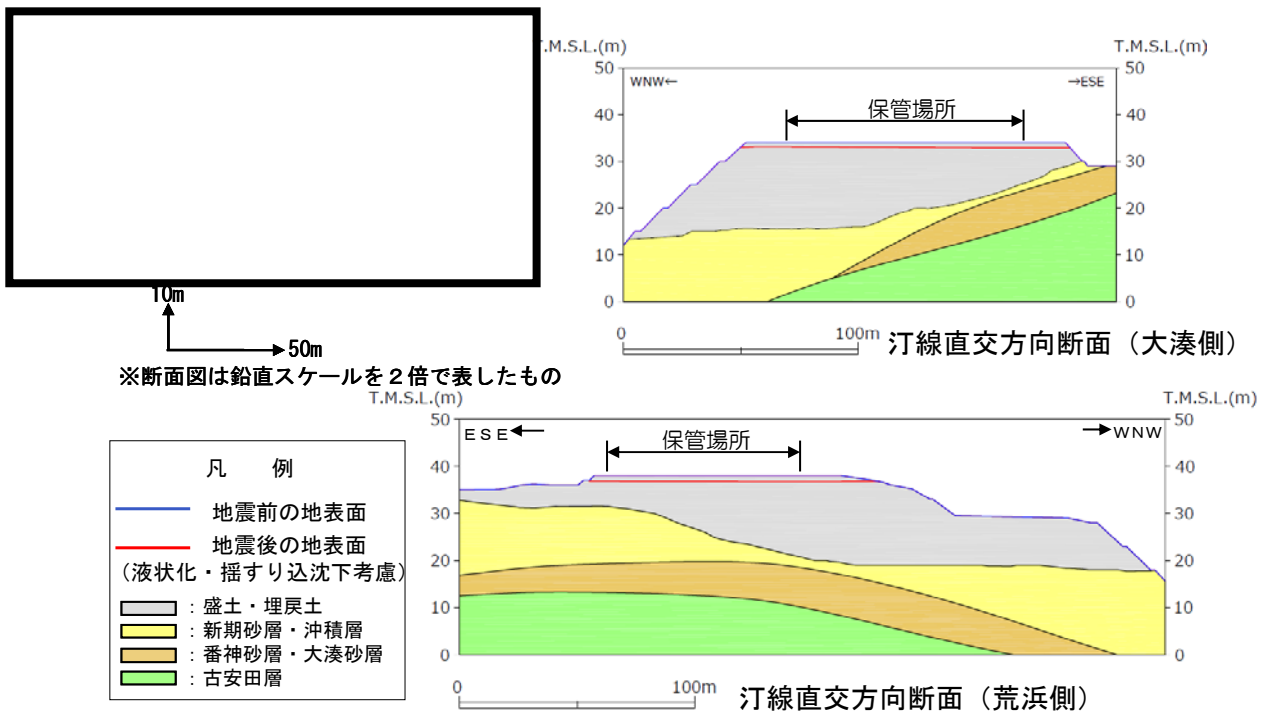
図 8-6 不等沈下評価結果
