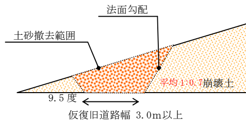
図 10 復旧法面のイメージ
