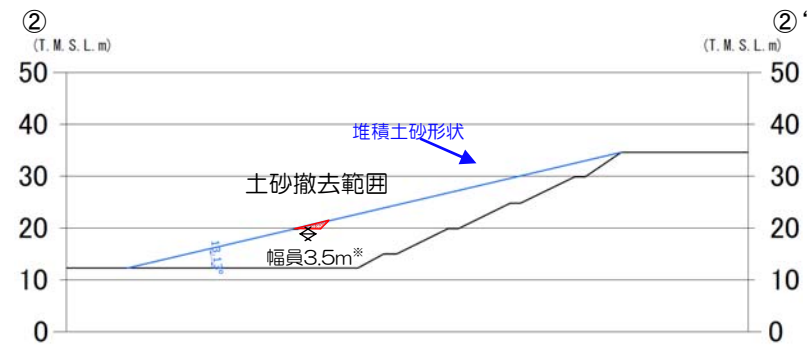
②-②'断面図
