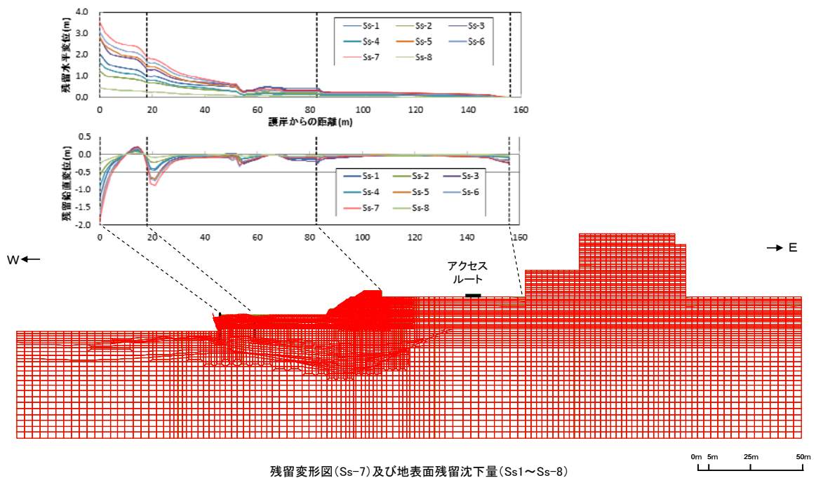
図 24-3 側方流動による地表面残留変形量評価結果
