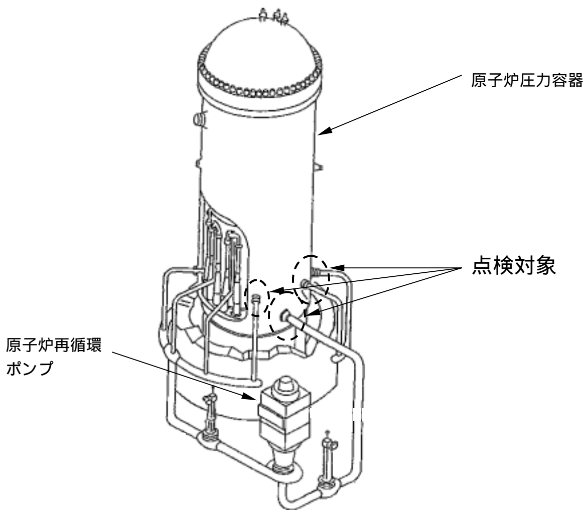
原子炉压力容器及び原子炉再循環系 概略図
