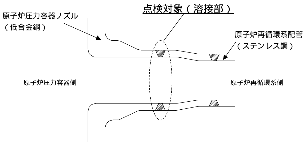
原子炉压力容器と原子炉再循環系配管の接続部の概略図
