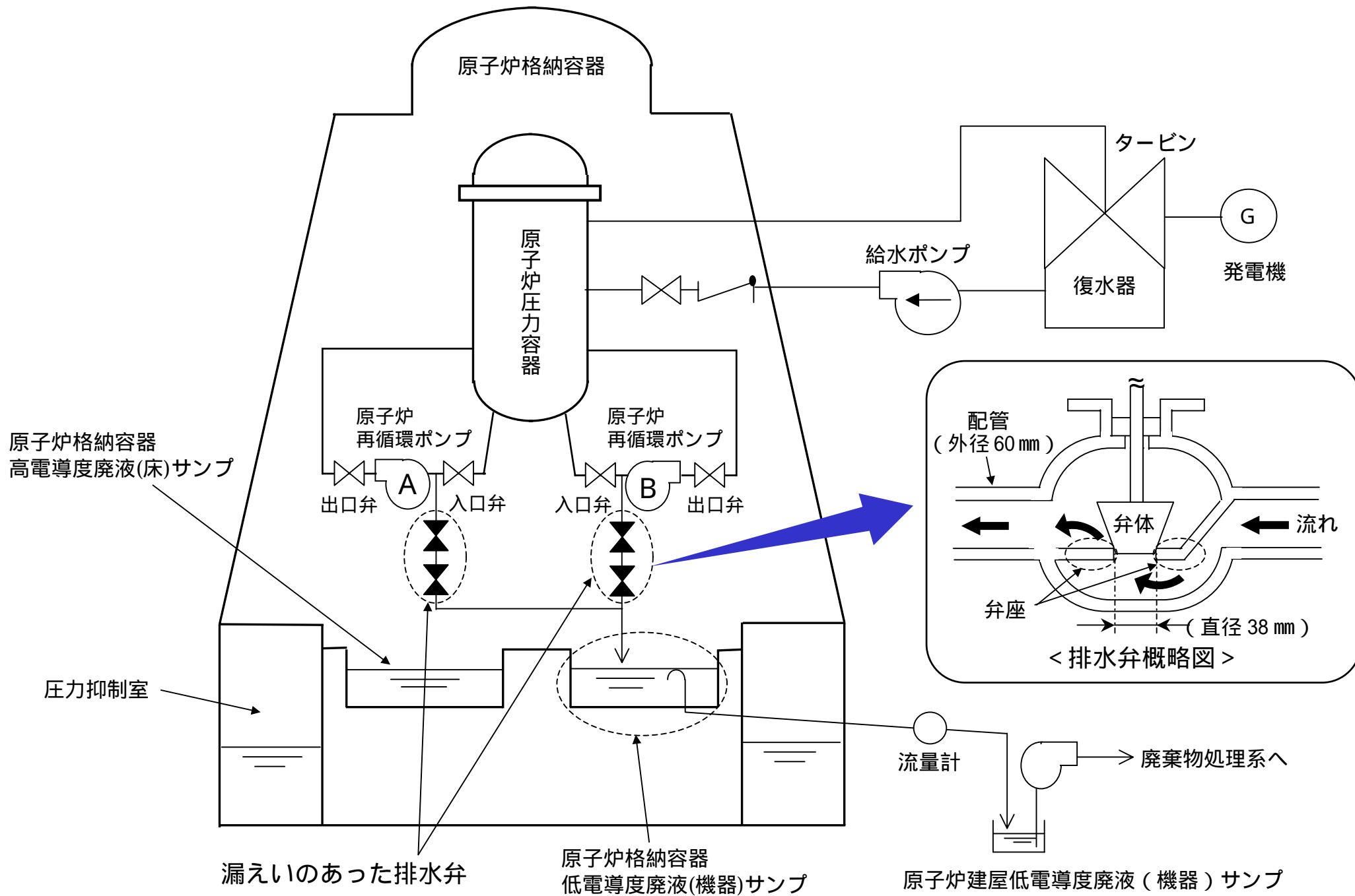
6号機原子炉格納容器低電導度廃液サンブ流入量増加の概略図
