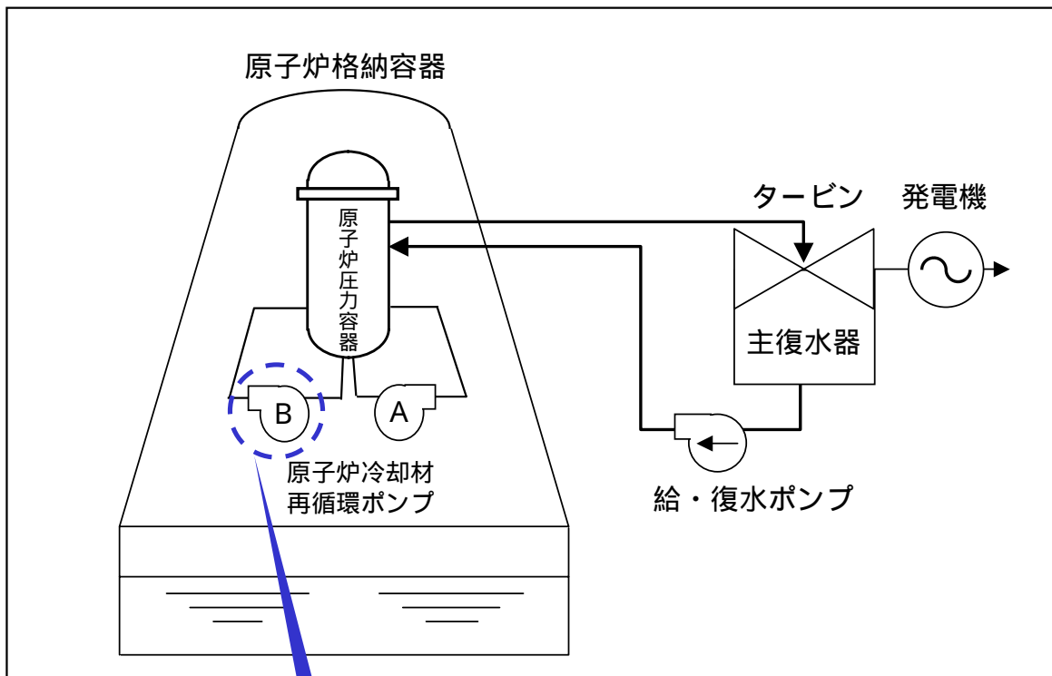
系統概略図
