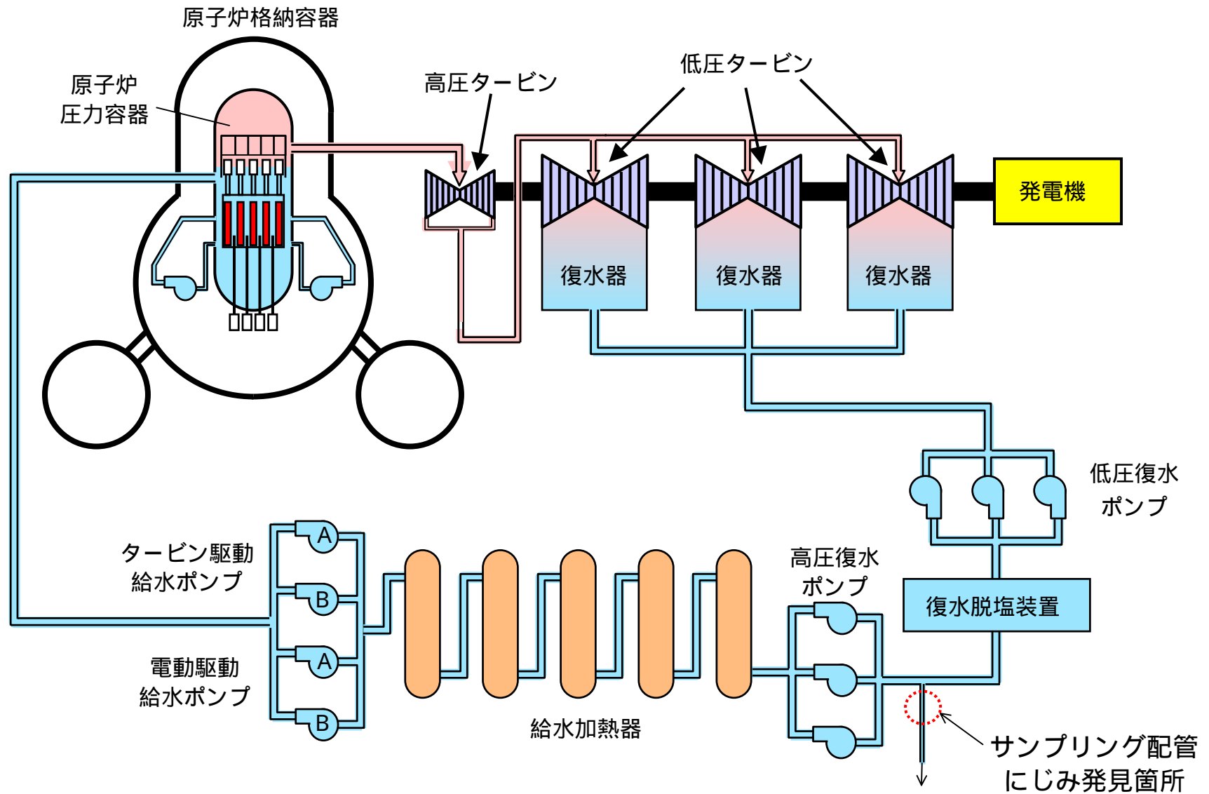
4号機系統概要図
