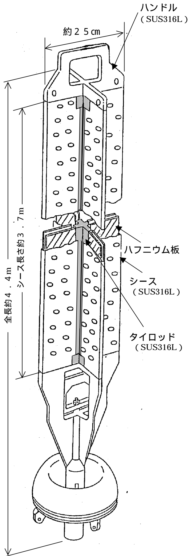
6号機制御棒（ハフニウム板型）概略図
