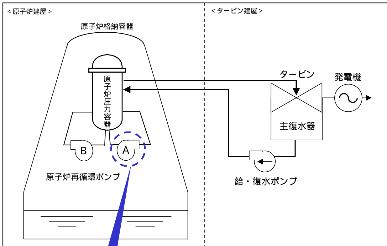
系 統 概 略 図
