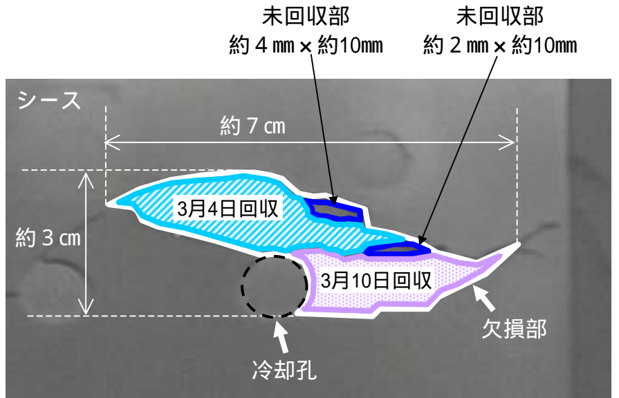
制御棒のシース部で確認された ひびおよび欠損部の状況
