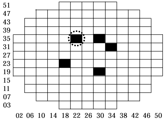
ひび等が確認された制御棒の炉内での位置
