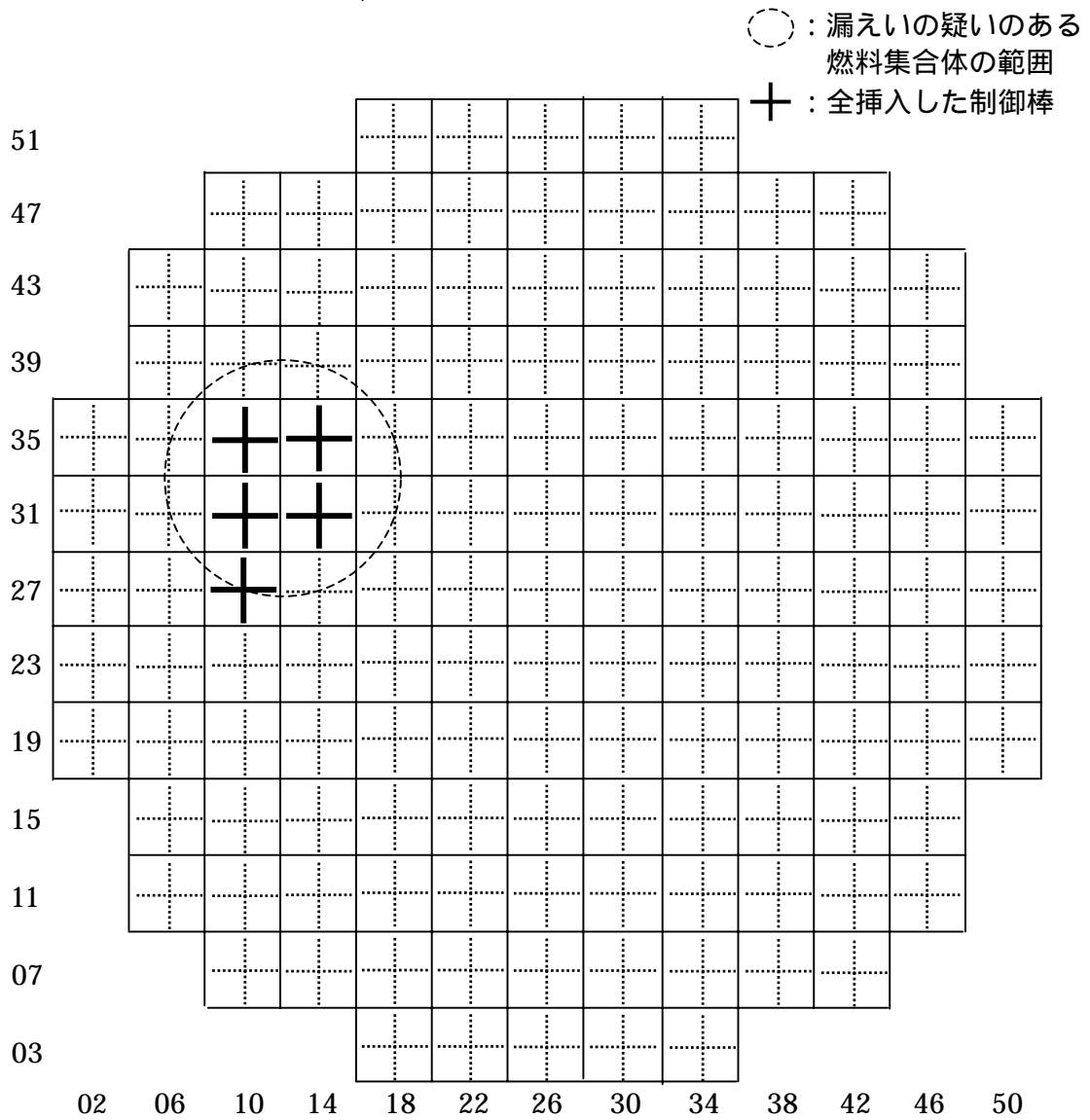
4号機における漏えいの疑いのある燃料集合体の範囲
