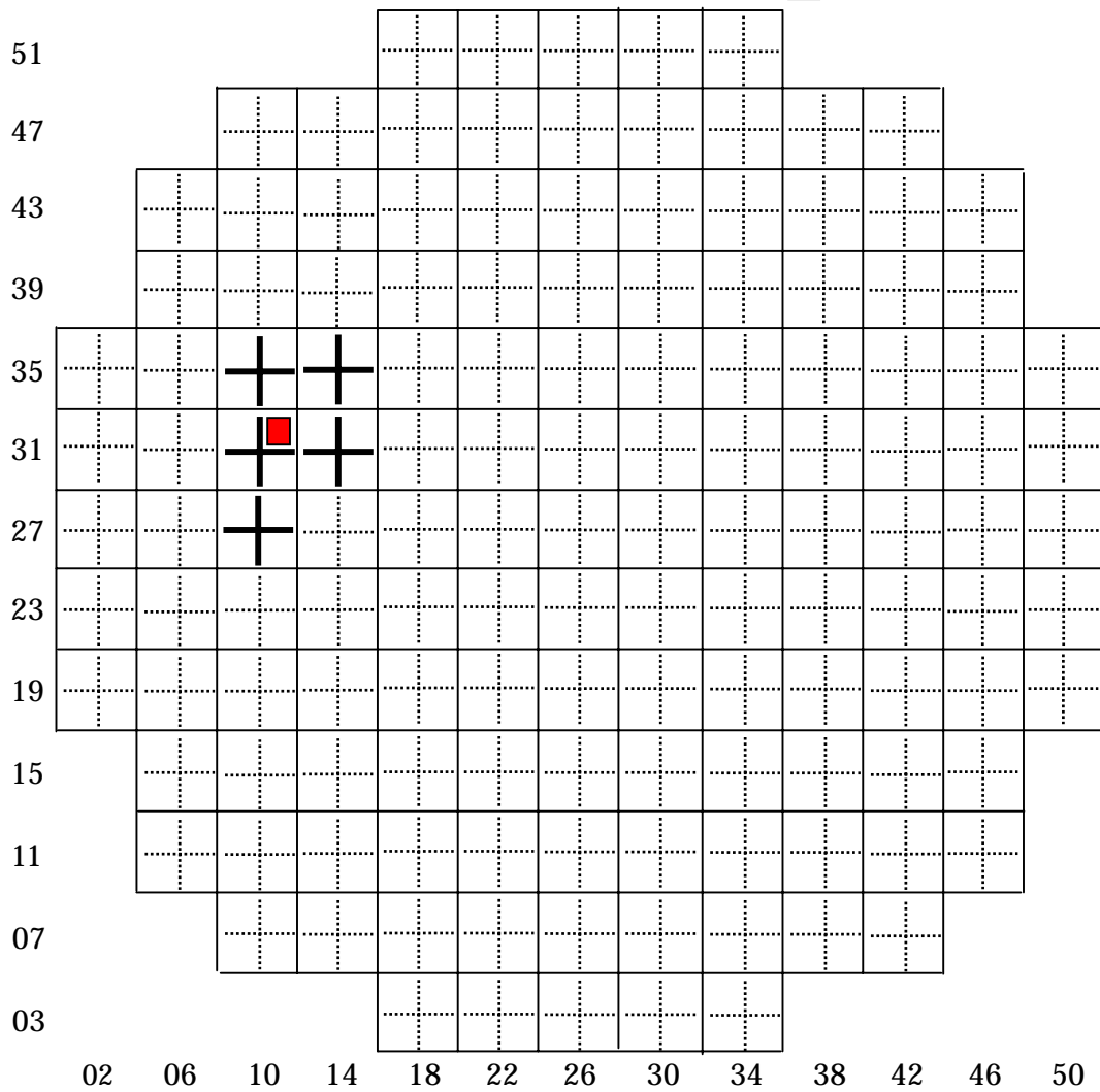
4号機漏えい燃料集合体の装荷位置
