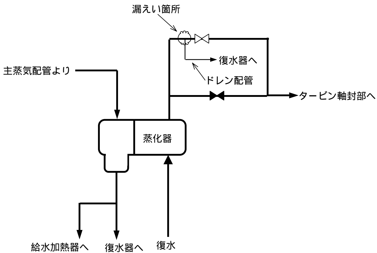
タービングランドシール蒸化系 系統概略図
