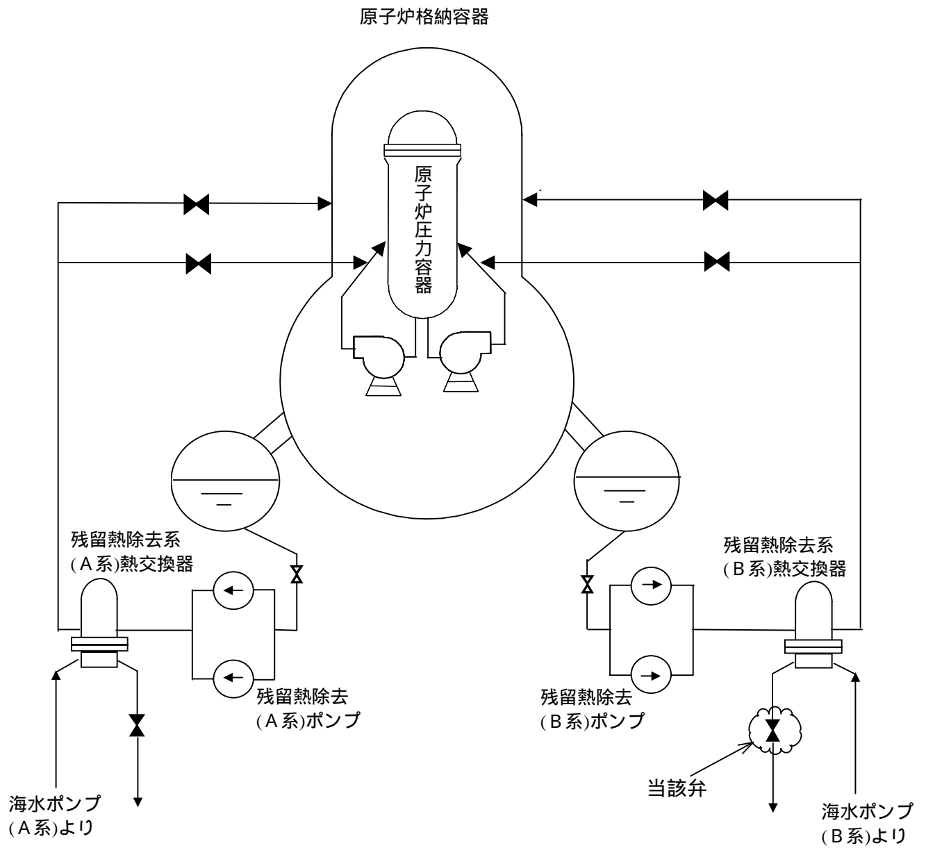
2号機残留熱除去系 系統概略図
