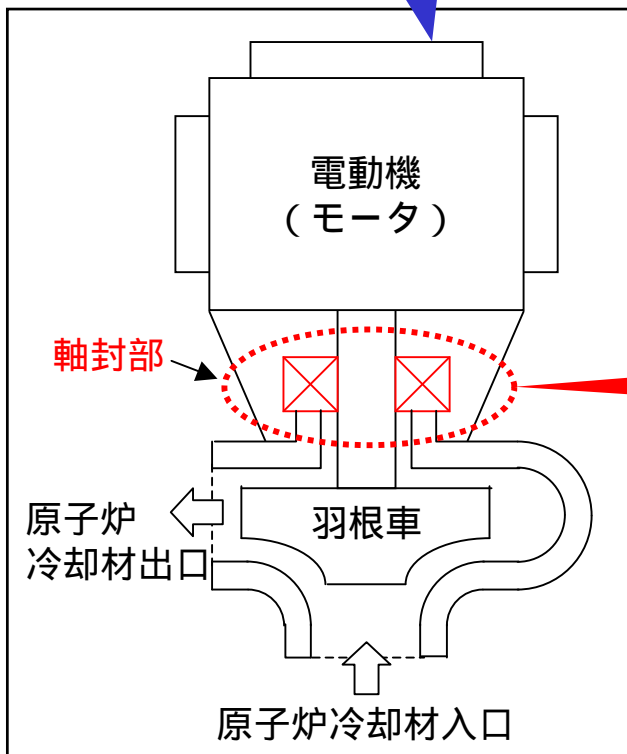
原子炉再循環ポンプ概略図
