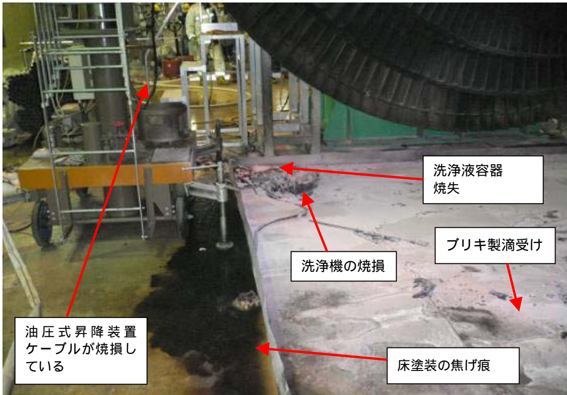
低圧タービン（A）ロータ下部の状況
