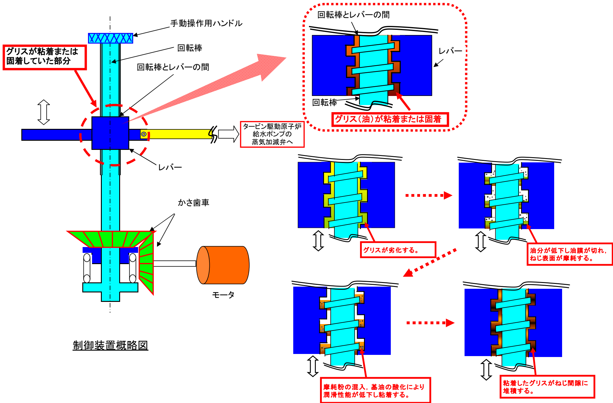
グリス劣化の推定メカニズム
