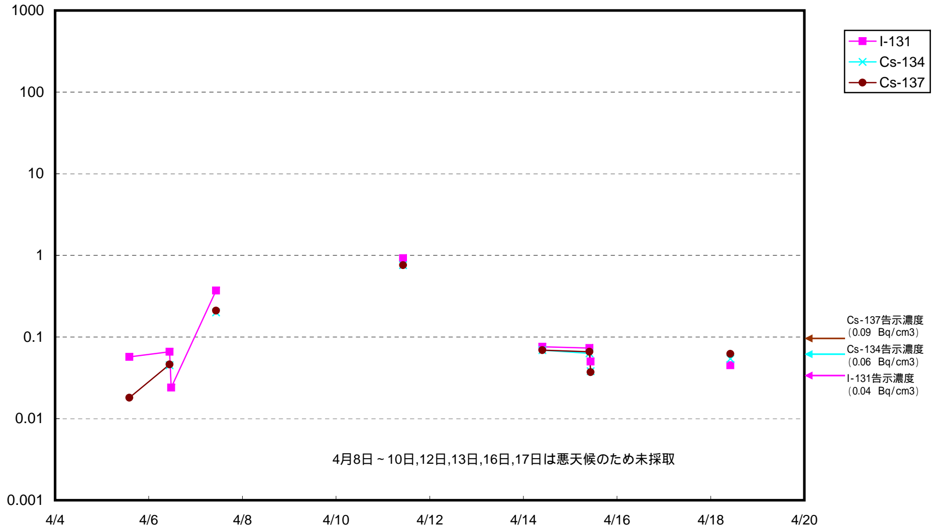
南相馬市沖合約15km付近 海水放射能濃度 (Bq / cm 3 )
