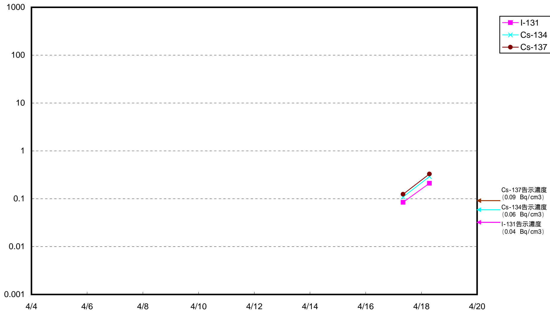
いわき市北部沖合3km付近 海水放射能濃度 (Bq / cm 3 )
