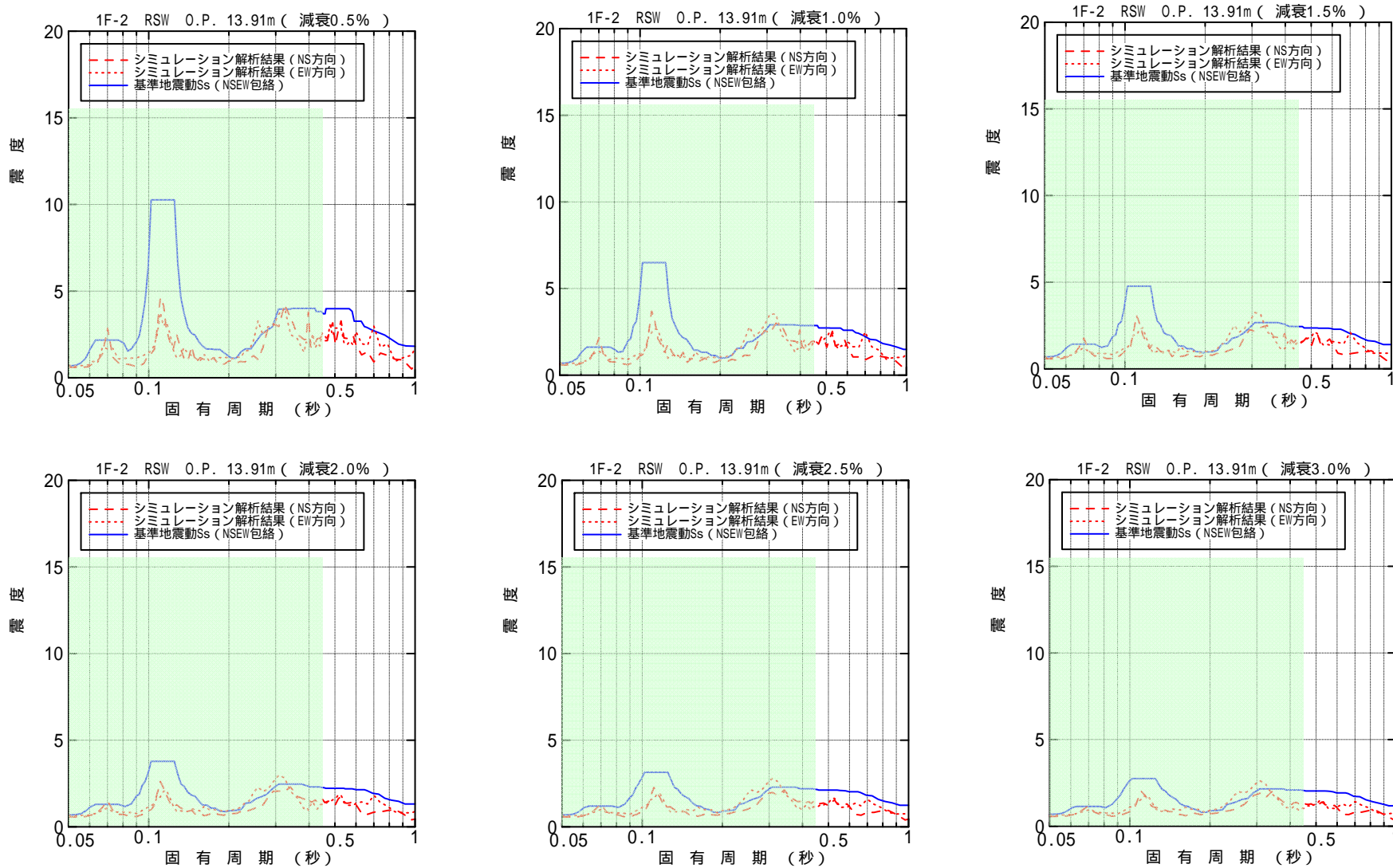
図-4.4.3.9 原子炉遮へい壁 O.P. 13.91m 床応答スペクトル (水平方向)
