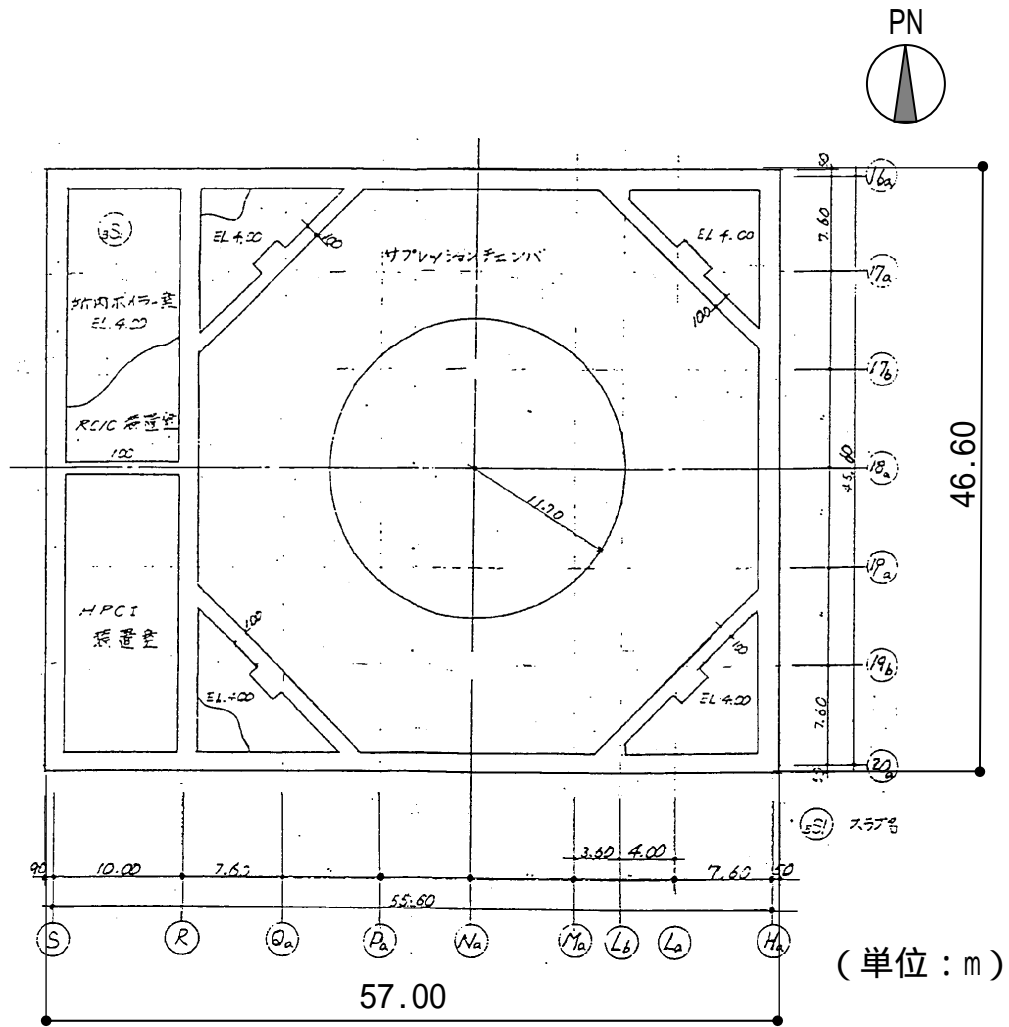
図-3.1.1 原子炉建屋の概略平面図
