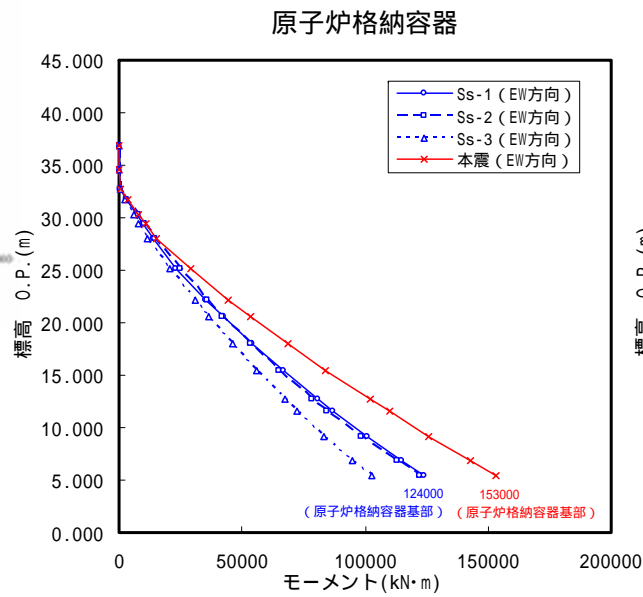
図-4.4.2.2.2 最大応答モーメント (NS,EW 方向) (原子炉格納容器, 原子炉压力容器 及び原子炉本体基礎)
