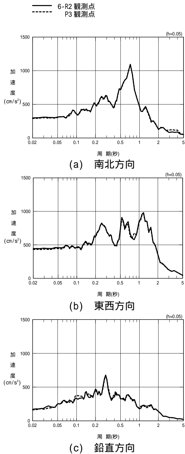
参図-1.3 近接する観測点における加速度応答スペクトルの比較 (h=0.05) ( 6号機原子炉建屋基礎版上 )
