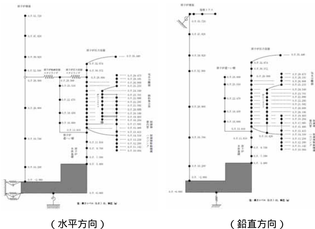
図-4.4.2.1.2 原子炉建屋 - 炉内構造物連成系モデル (福島第一2号機)
