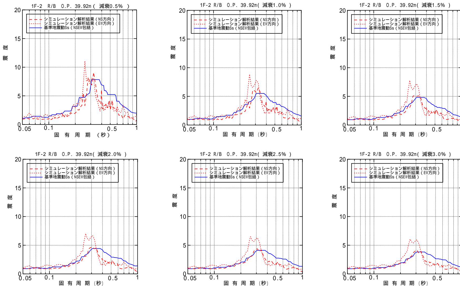
図-4.4.3.1 原子炉建屋 0.P. 39.92m 床応答スペクトル (水平方向)
