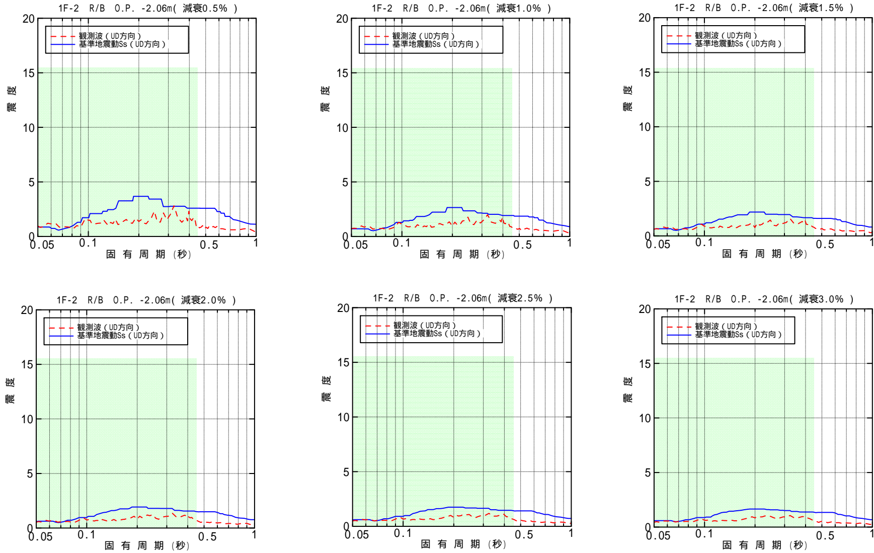
図-4.4.3.6 原子炉建屋 O.P. -2.06m 床応答スペクトル (鉛直方向)
