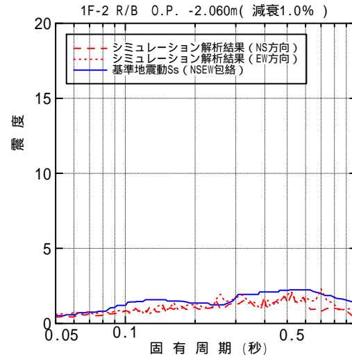
床応答スペクトル（水平）
