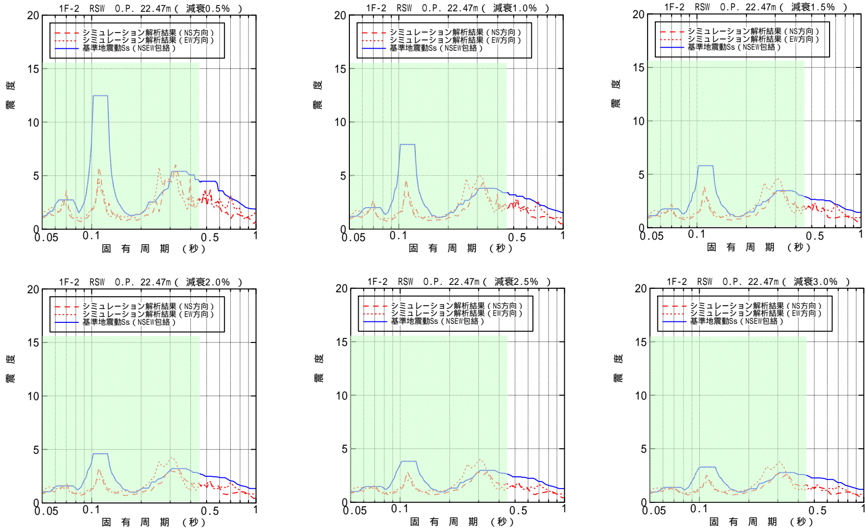
図-4.4.3.8 原子炉遮へい壁 O.P. 22.47m 床応答スペクトル(水平方向)
