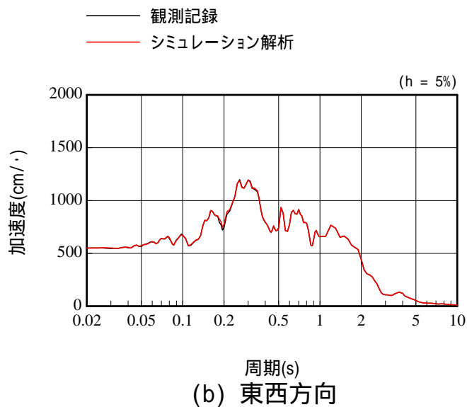
参図-2.2 2号機原子炉建屋基礎版上の加速度応答スペクトルの比較 観測記録(2-R2)とシミュレーション解析結果に基づく応答波
