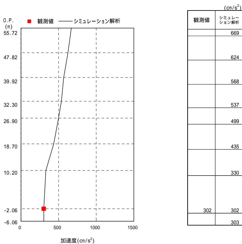
図-3.5.1(3) 最大応答加速度 (鉛直方向)
