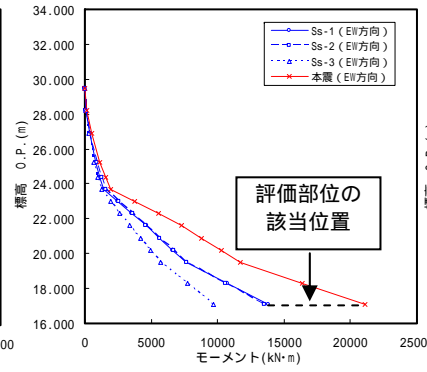
シュラウドサポートに作用する地震荷重
