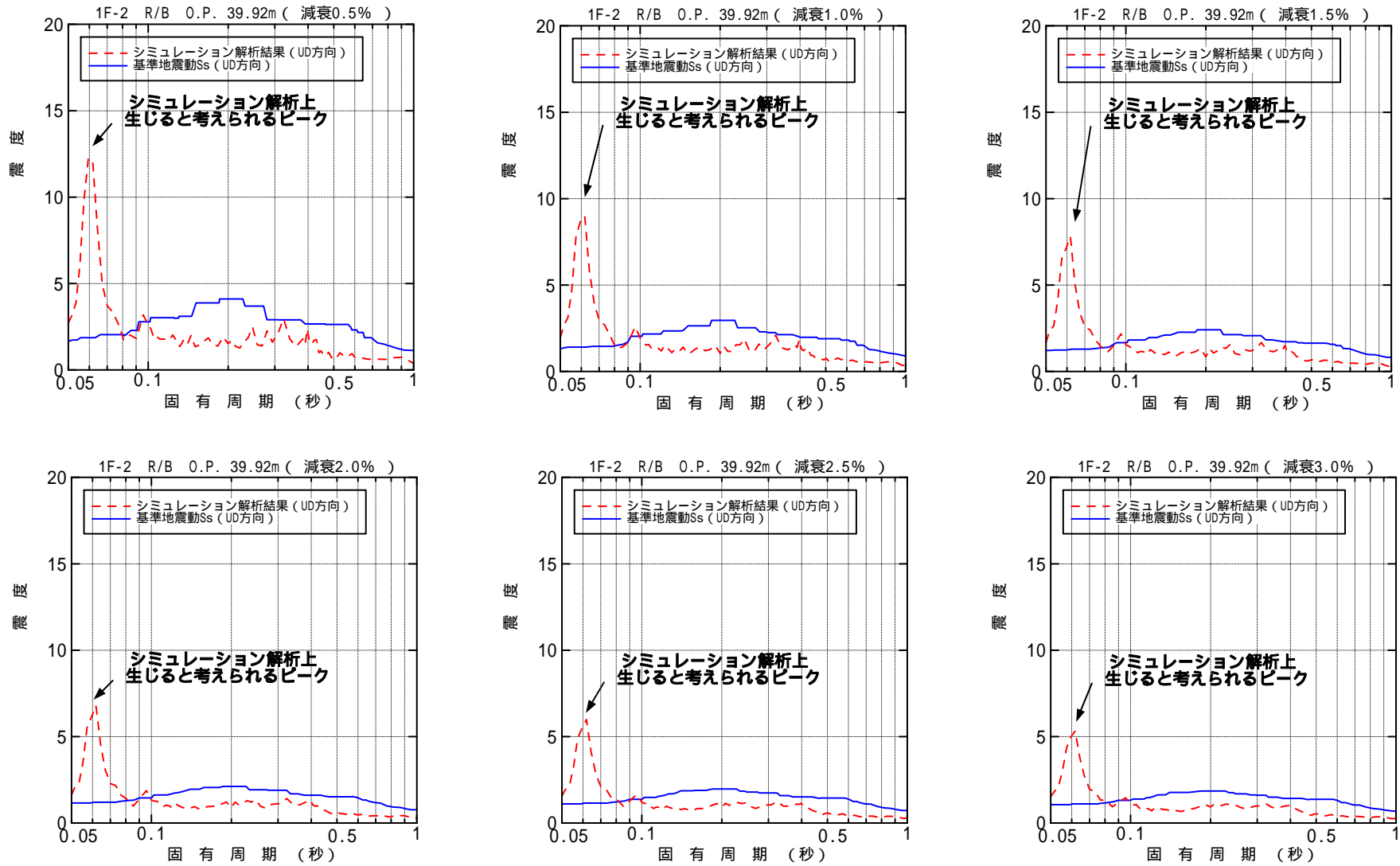
図-4.4.3.4 原子炉建屋 0.P. 39.92m 床応答スペクトル (鉛直方向)
