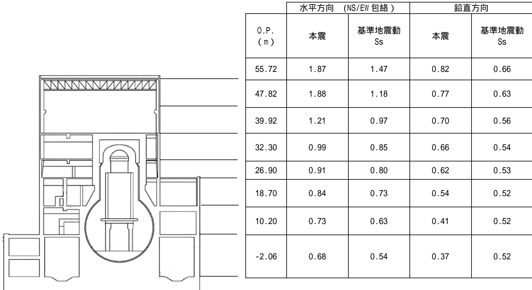
図-4.4.1.1 原子炉建屋の評価用震度
