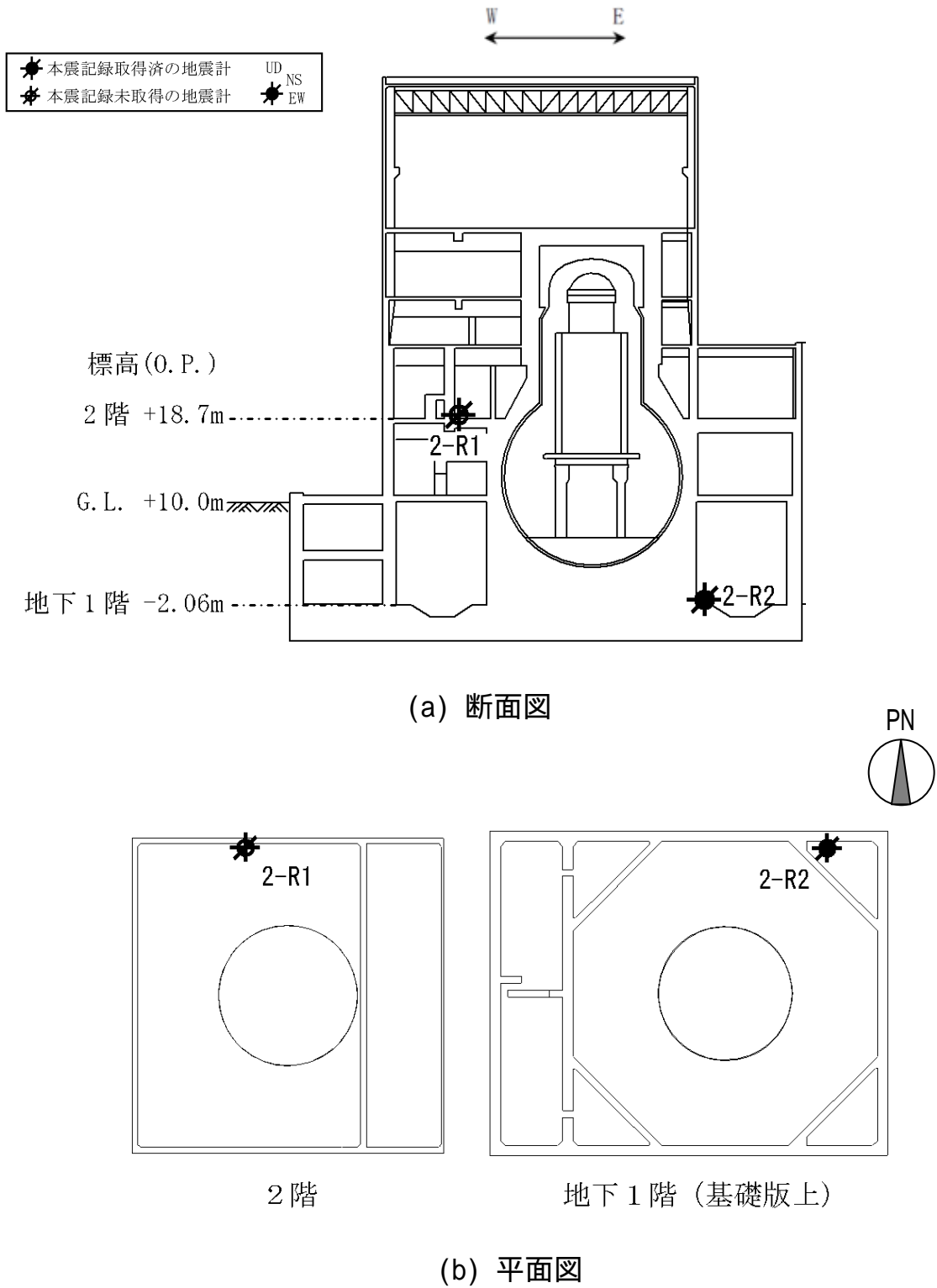
図-3.2.1 原子炉建屋内の地震観測位置
