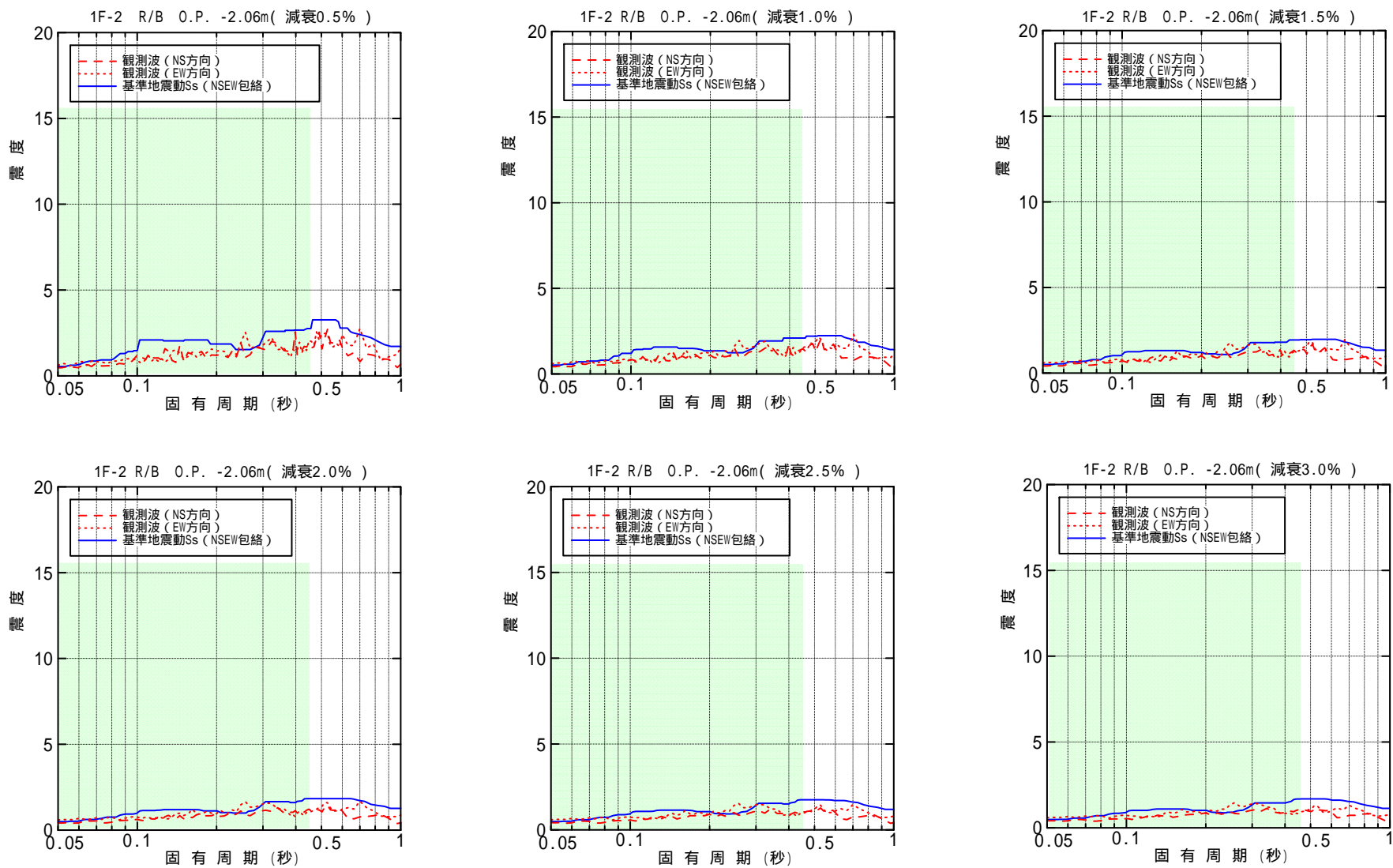
図-4.4.3.3 原子炉建屋 0.P. -2.06m 床応答スペクトル (水平方向)
