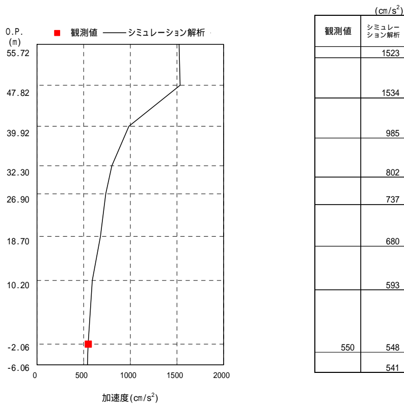
図-3.5.1(2) 最大応答加速度（東西方向）
