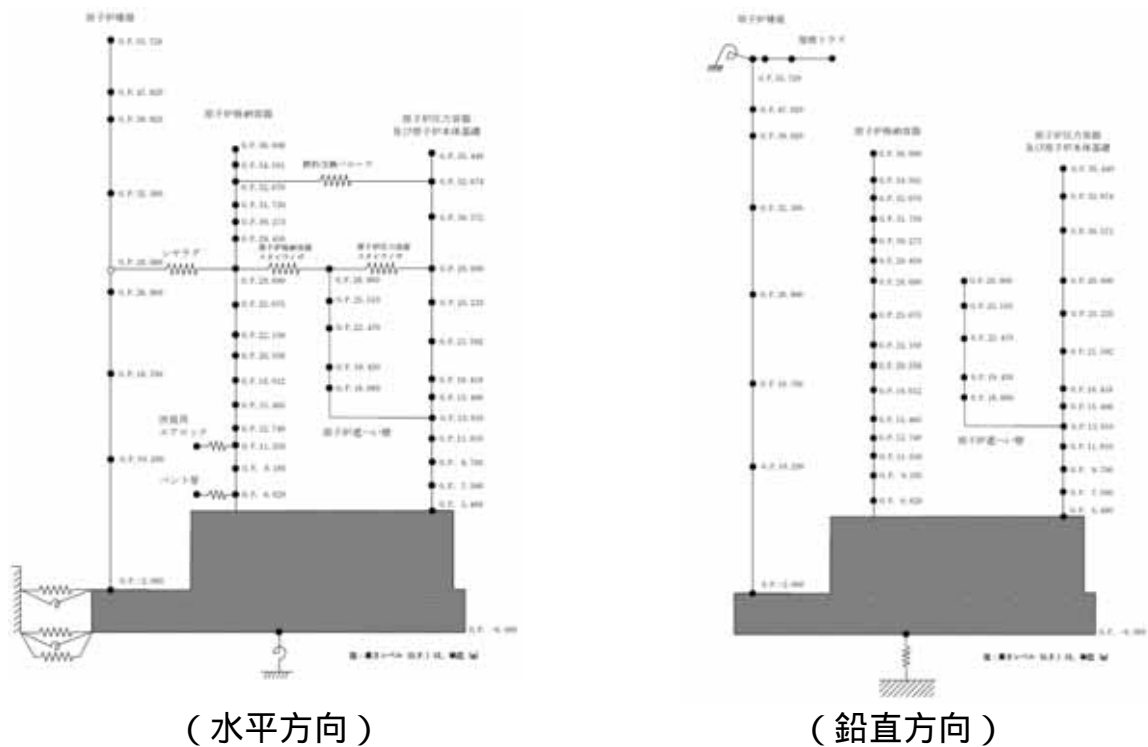
図-4.4.2.1.1 原子炉建屋 - 原子炉格納容器 - 原子炉压力容器連成系モデル (福島第一2号機)
