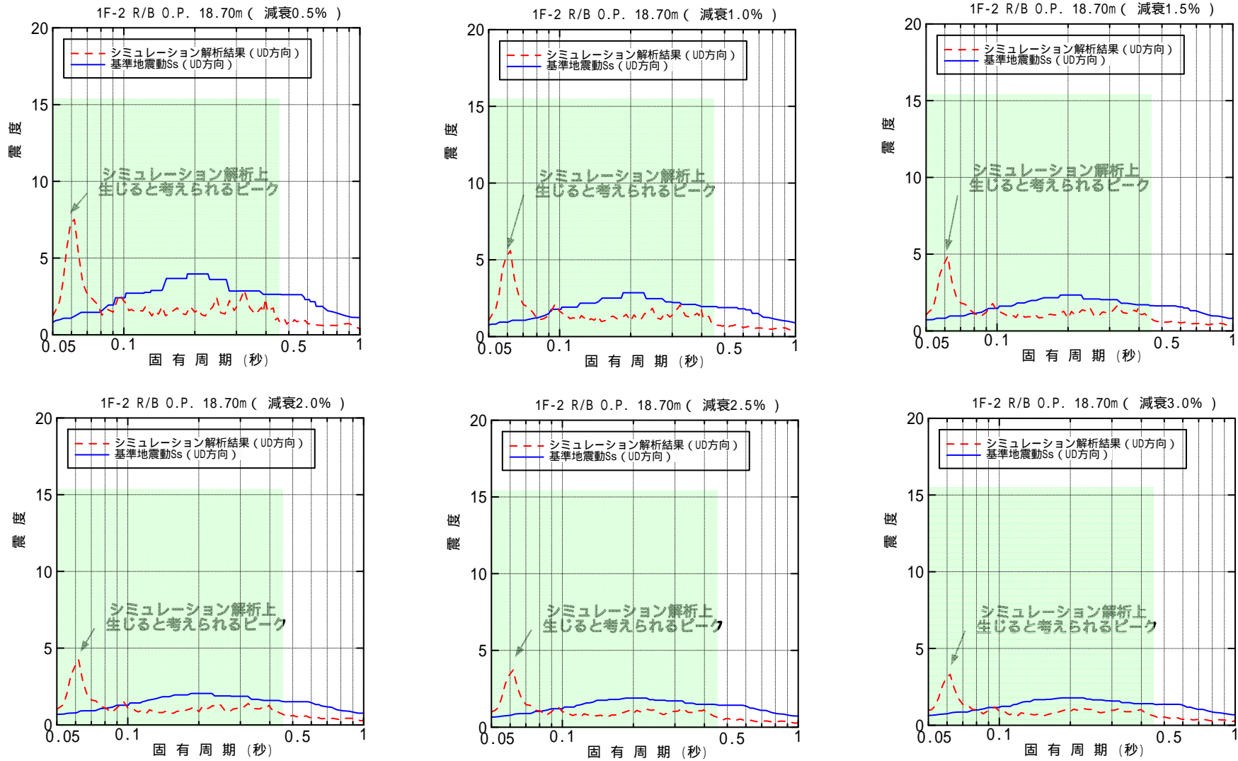
図-4.4.3.5 原子炉建屋 O.P. 18.70m 床応答スペクトル(鉛直方向)
