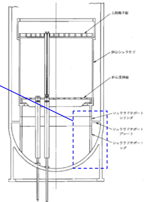
炉内構造物模式図
