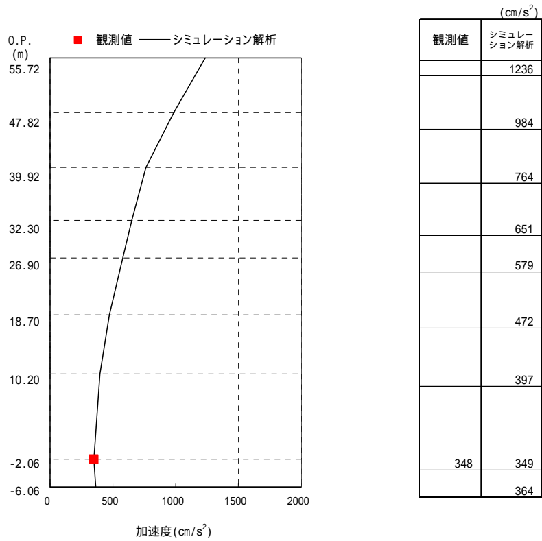
図-3.5.1(1) 最大応答加速度（南北方向）
