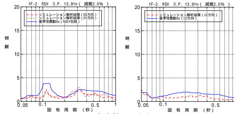
床応答スペクトル
