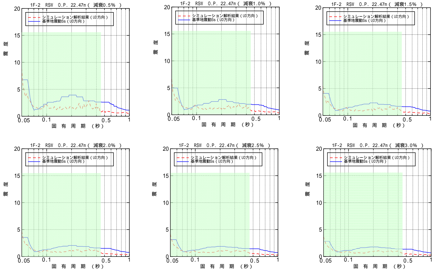
図-4.4.3.11 原子炉遮へい壁 O.P. 22.47m 床応答スペクトル (鉛直方向)
