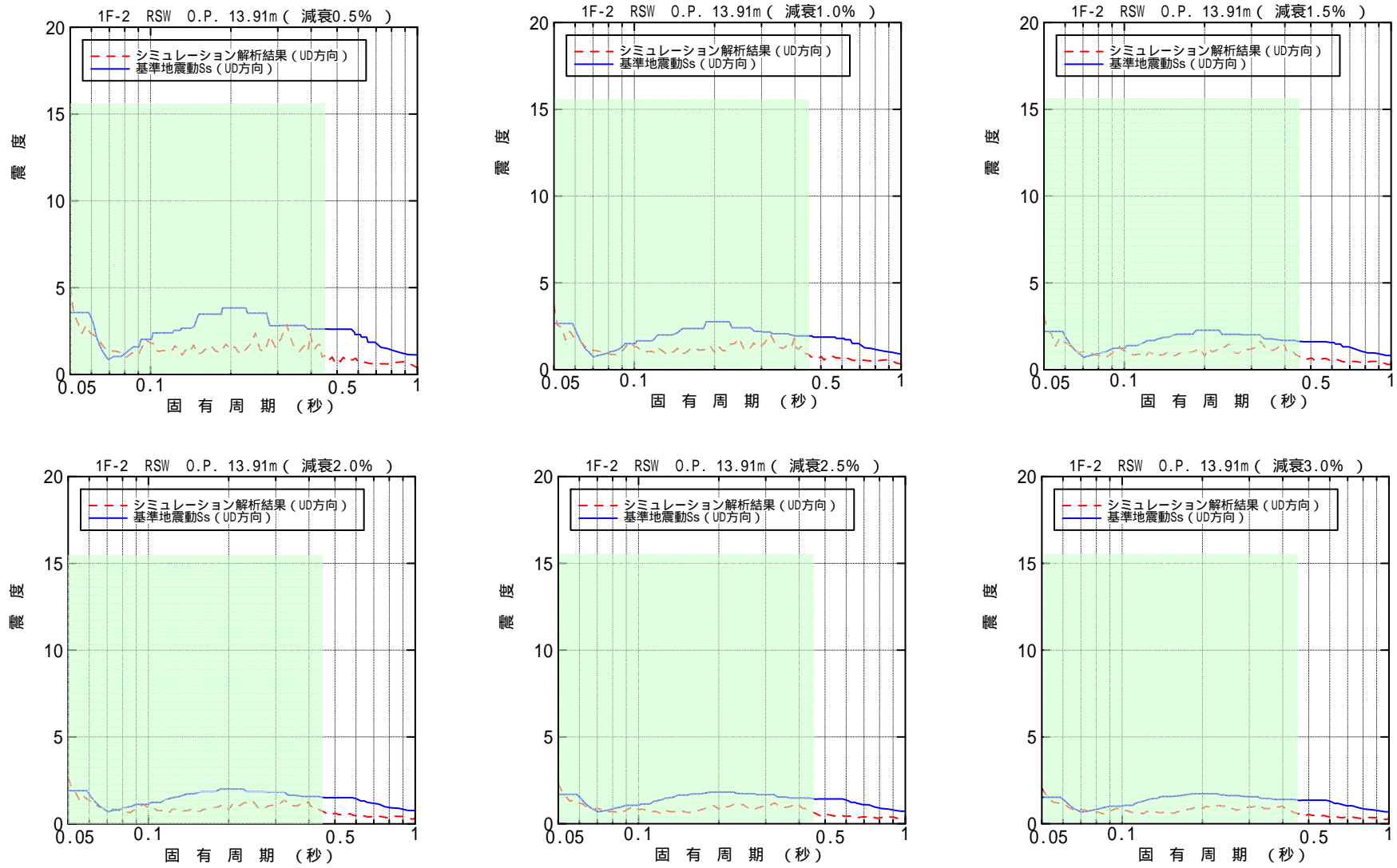
図-4.4.3.12 原子炉遮へい壁 O.P. 13.91m 床応答スペクトル (鉛直方向)
