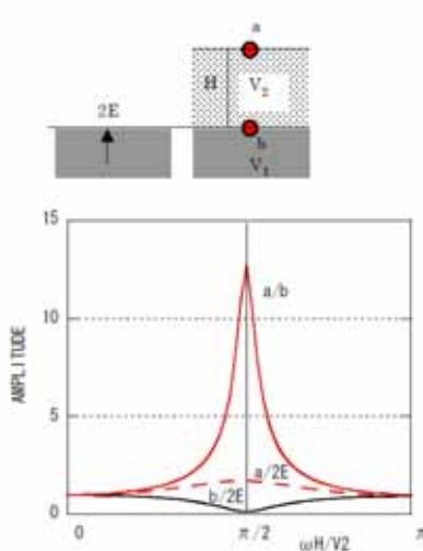
2層地盤の周波数伝達関数 q=0.5 : \alpha = (\nu_1 - \nu_2) / \nu_1 比
