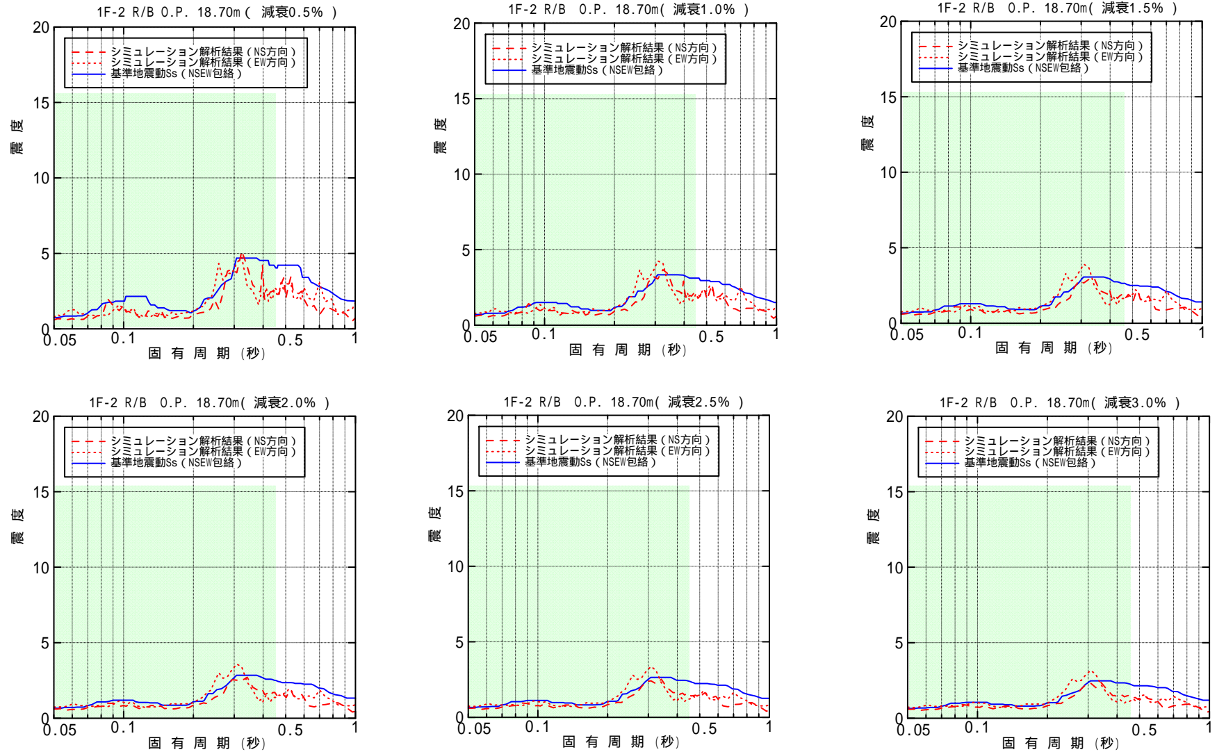
図-4.4.3.2 原子炉建屋 0.P. 18.70m 床応答スペクトル (水平方向)
