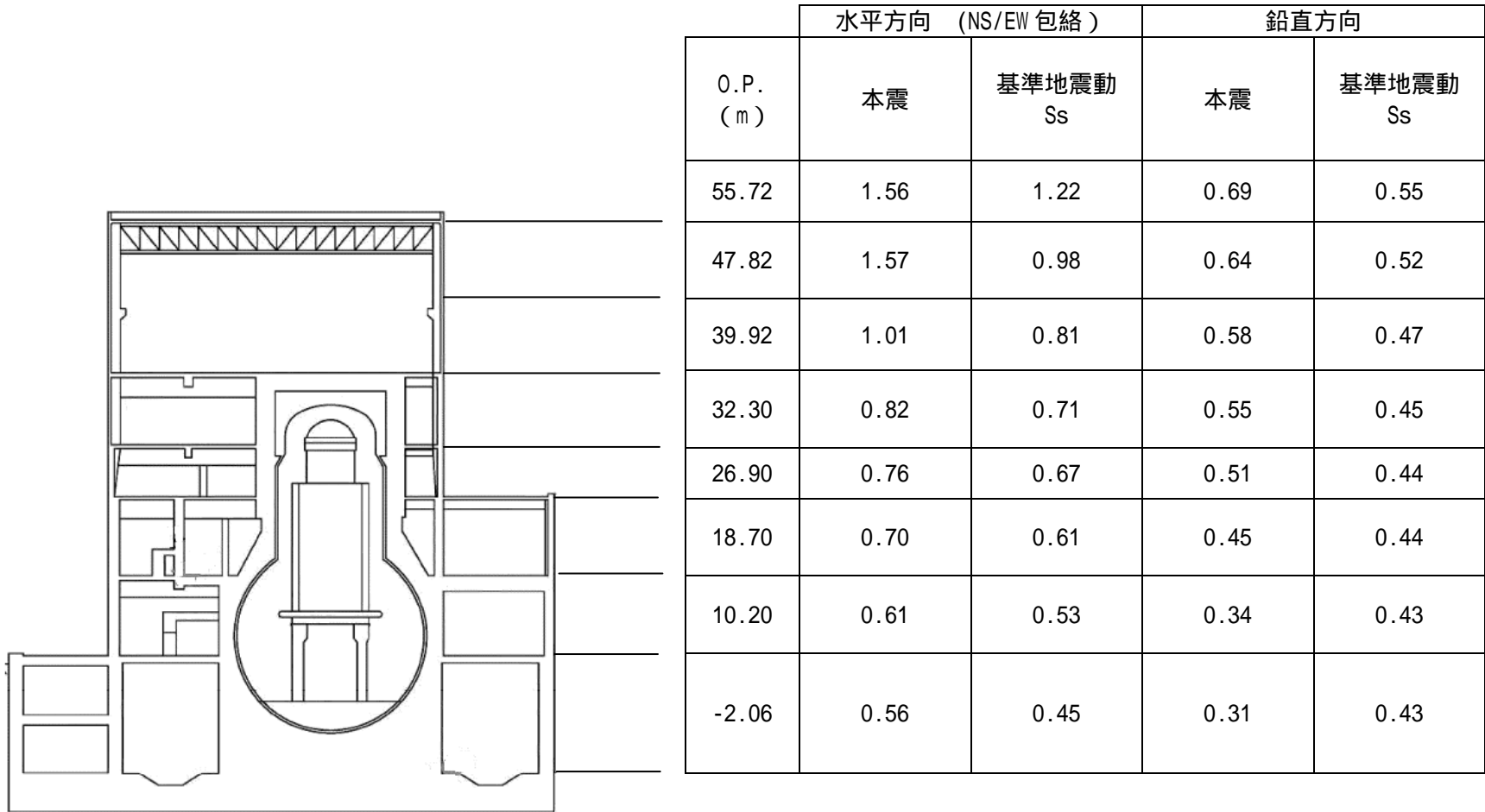
参图-4.1 原子炉建屋の最大応答加速度
