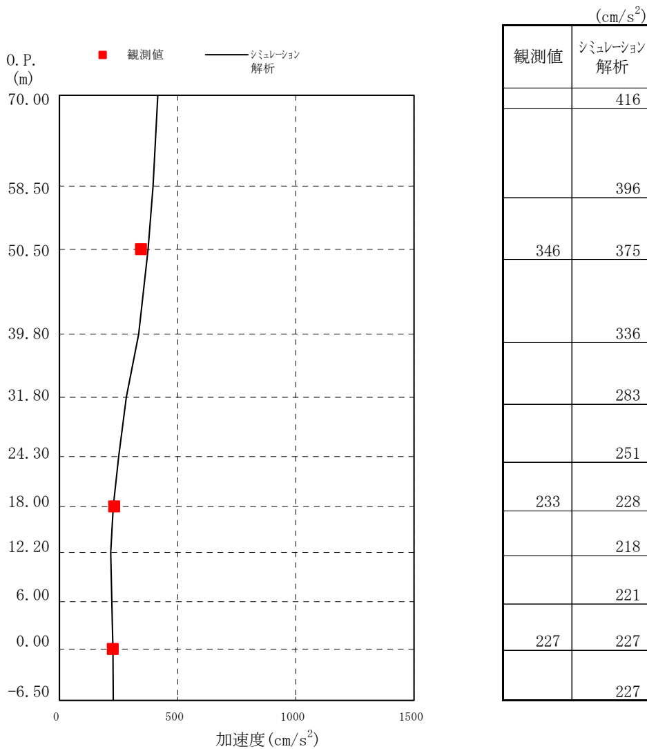
図-3.5.1(3) 最大応答加速度 (鉛直方向)
