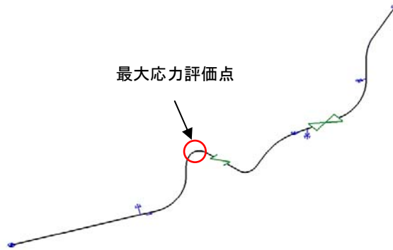
残留熱除去系配管モデル (一部)
