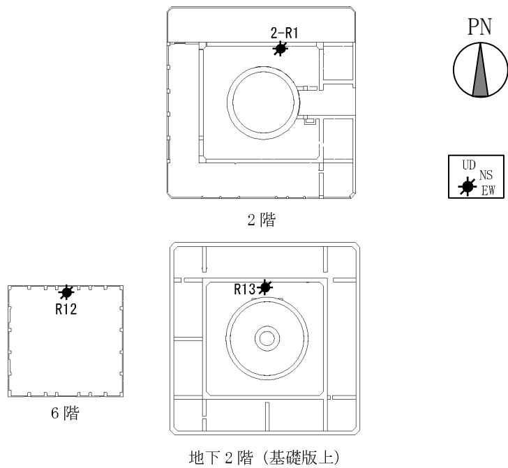
(b) 平面図
