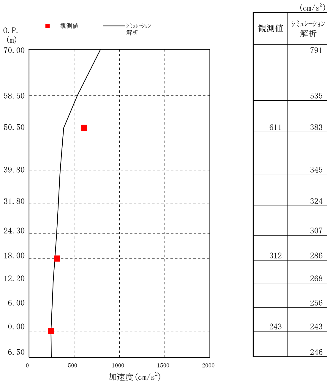
図-3.5.1(1) 最大応答加速度 (南北方向)
