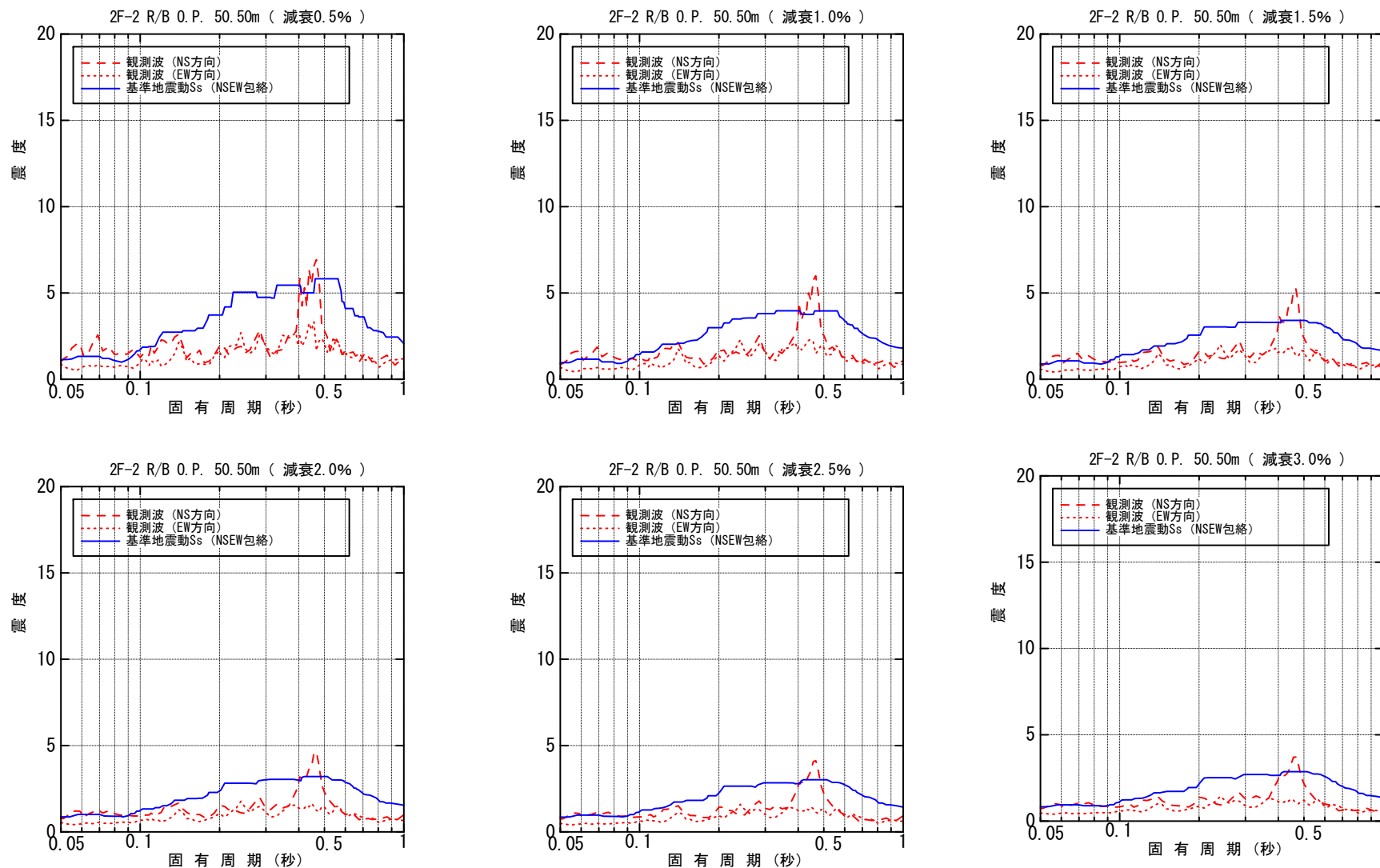
図-4.4.3.1 原子炉建屋 O.P. 50.50m 床応答スペクトル (水平方向)
