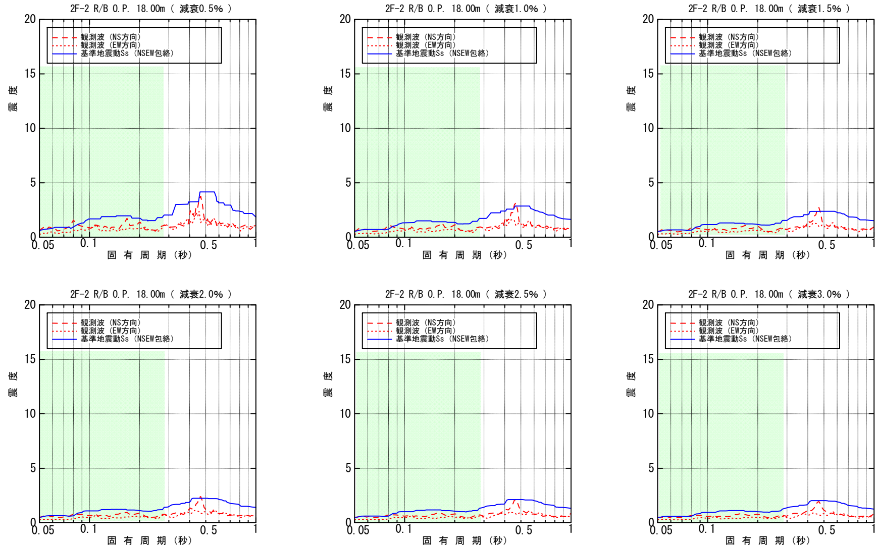
図-4.4.3.2 原子炉建屋 O.P. 18.00m 床応答スペクトル (水平方向)
