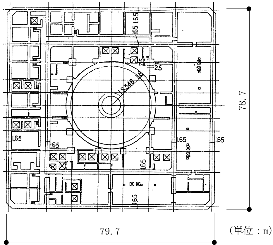
図-3.1.1 原子炉建屋の概略平面図
