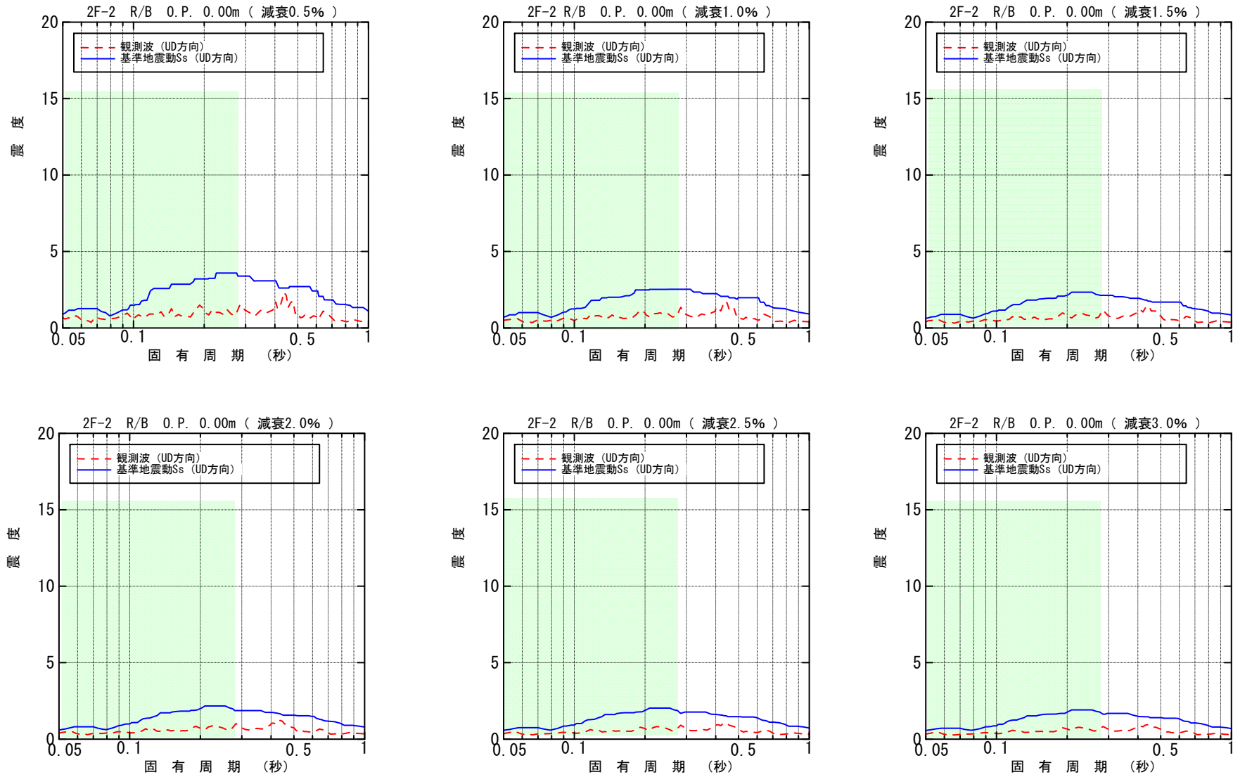
図-4.4.3.6 原子炉建屋 0.P. 0.00m 床応答スペクトル (鉛直方向)
