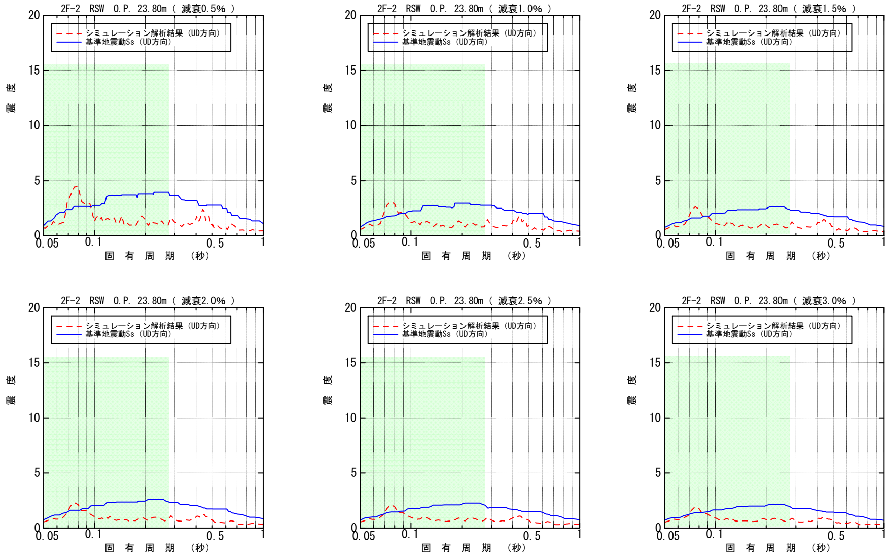
図-4.4.3.12 原子炉遮へい壁 O.P. 23.80m 床応答スペクトル (鉛直方向)
