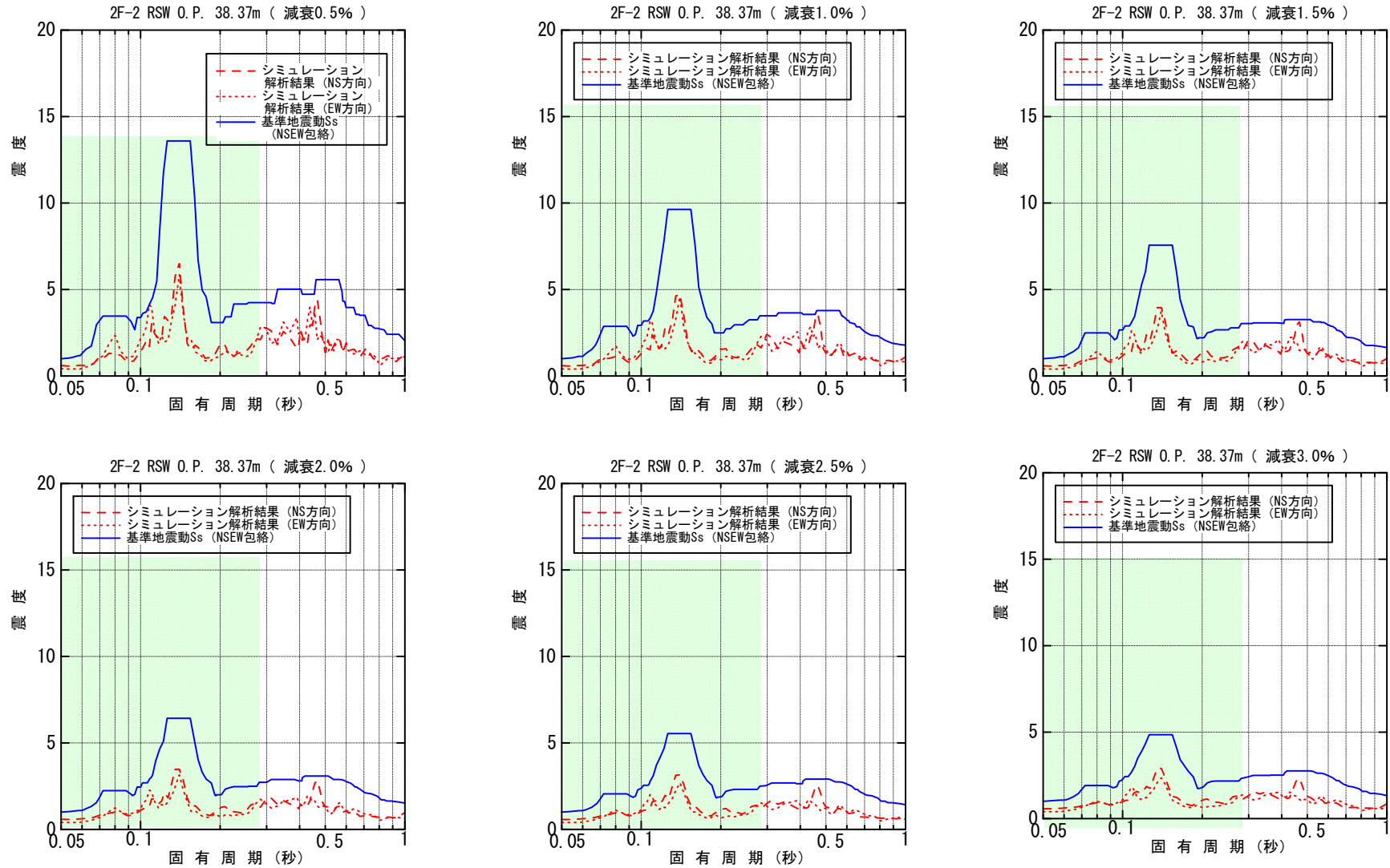
図-4.4.3.7 原子炉遮へい壁 O.P. 38.37m 床応答スペクトル (水平方向)
