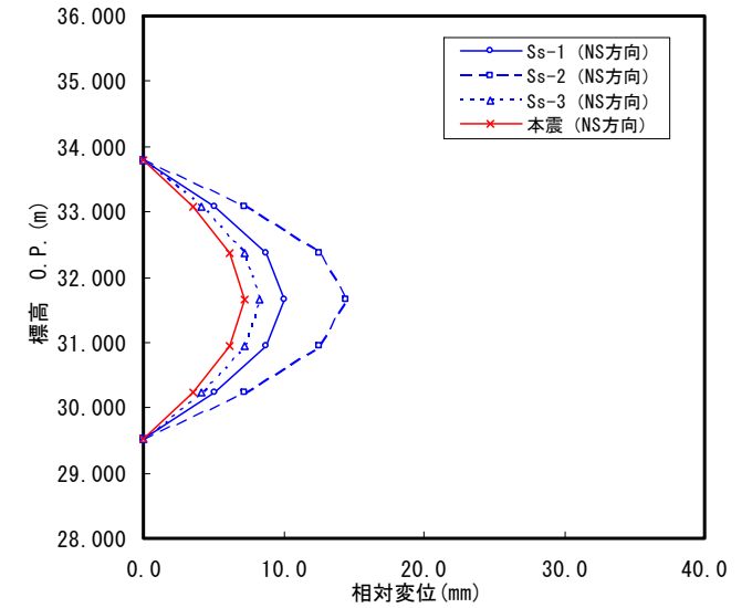
燃料集合体の相対変位 (NS 方向)
