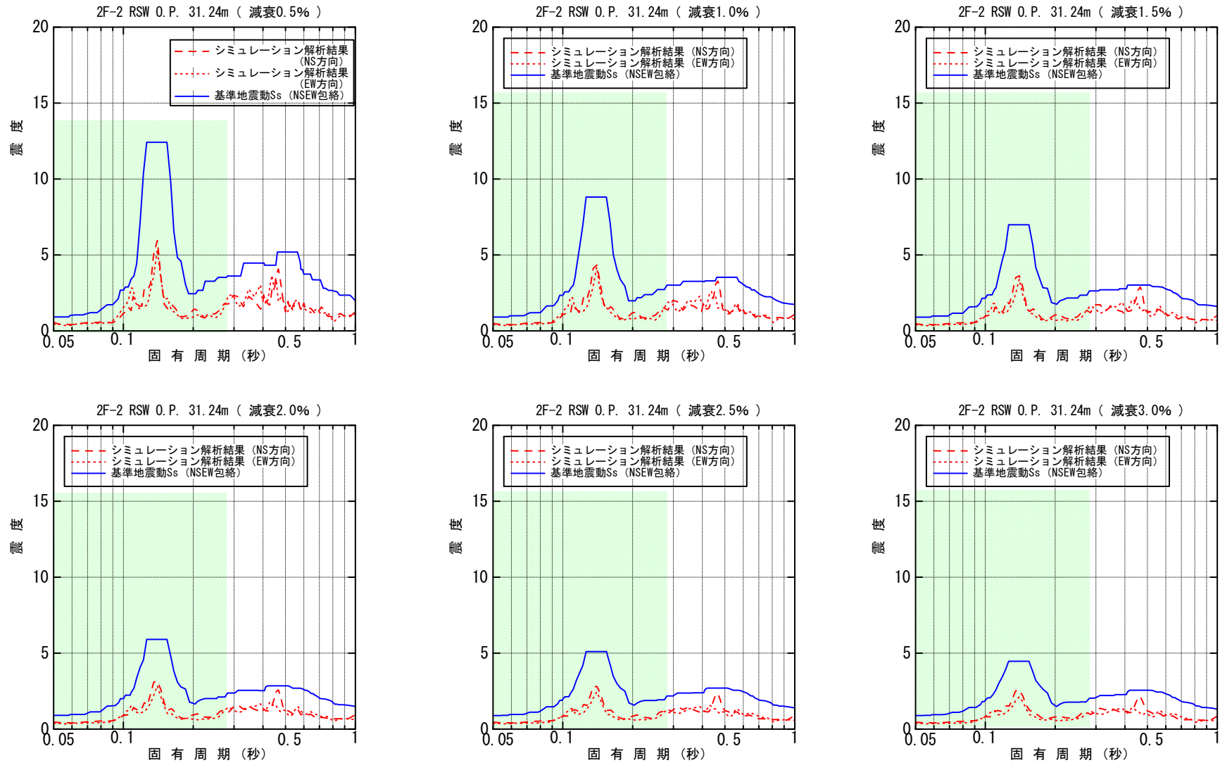
図-4.4.3.8 原子炉遮へい壁 0.P. 31.24m 床応答スペクトル (水平方向)
