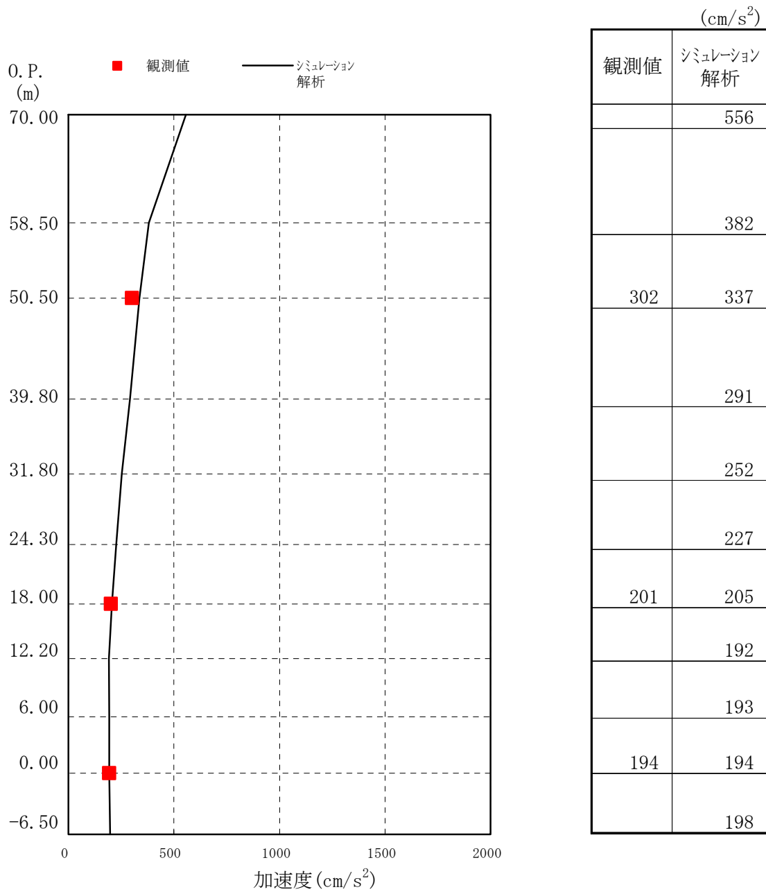
図-3.5.1(2) 最大応答加速度 (東西方向)
