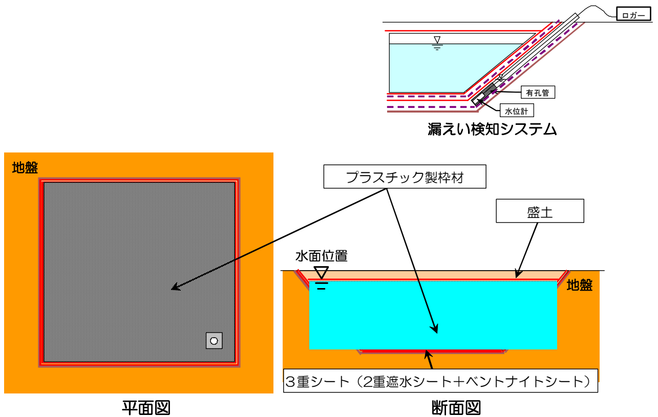
図2 地下貯水槽概要図
