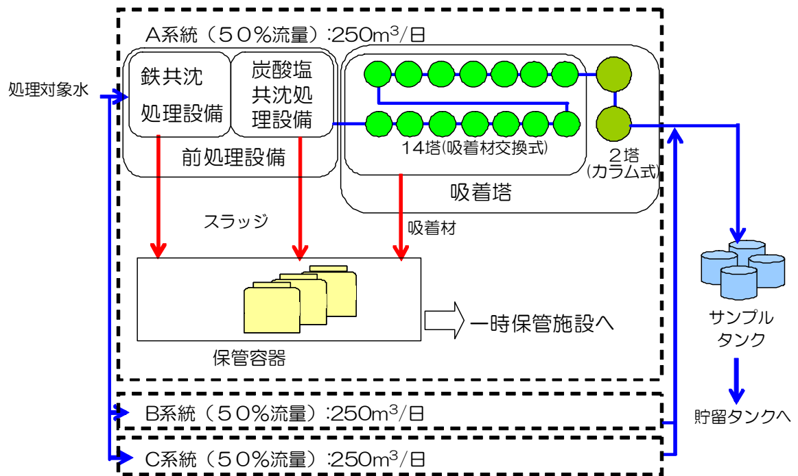
図1 多核種除去設備系統概要
