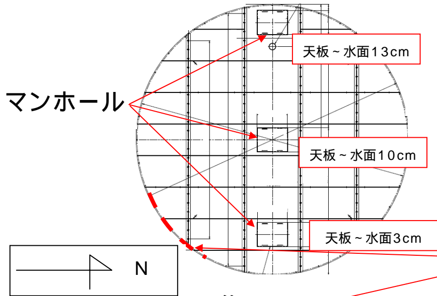
点検用足場底部拡大
