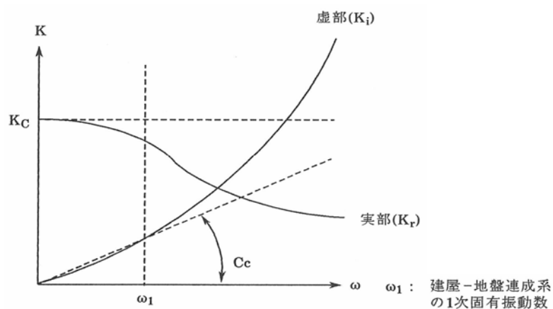
図－２３ 地盤ばねの近似
