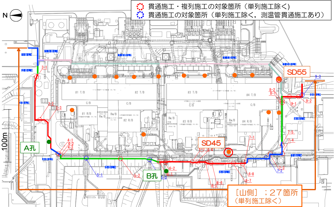
図 1 4 - 2 8 凍土壁ライン近傍のサブドレン・地下水位観測孔 配置図
