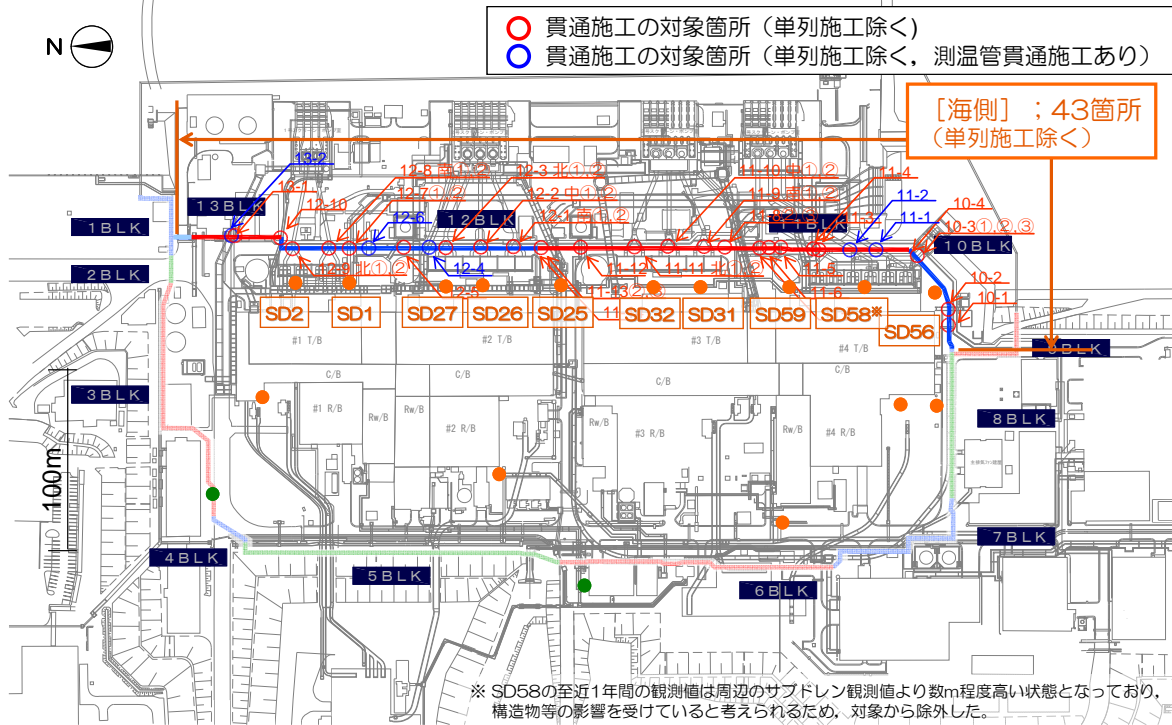
図 5 - 3 1 凍土壁ライン近傍のサブドレン・地下水位観測孔 配置図
