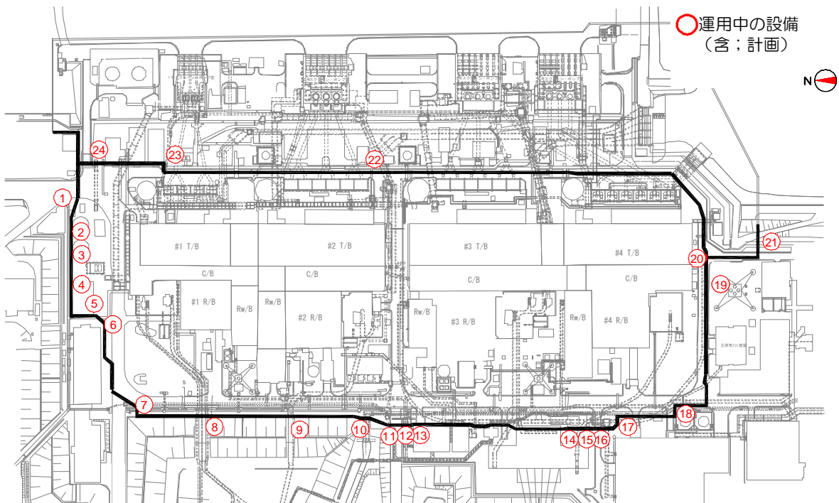
図7 主な運用中の設備と凍土遮水壁の横断箇所
