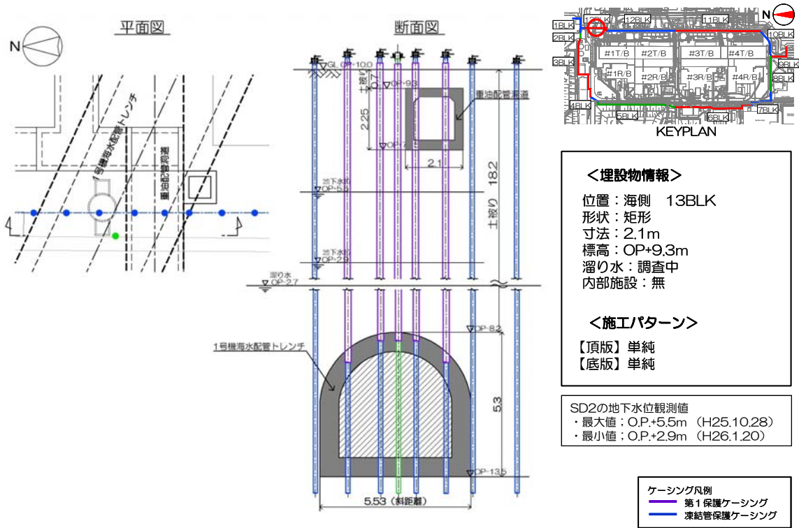
図5-29 【13-1】重油配管トレンチ 施工方法（貫通施工）
