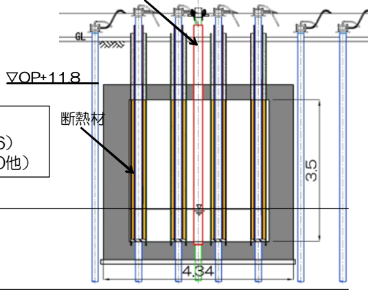
測温管 横断面図
