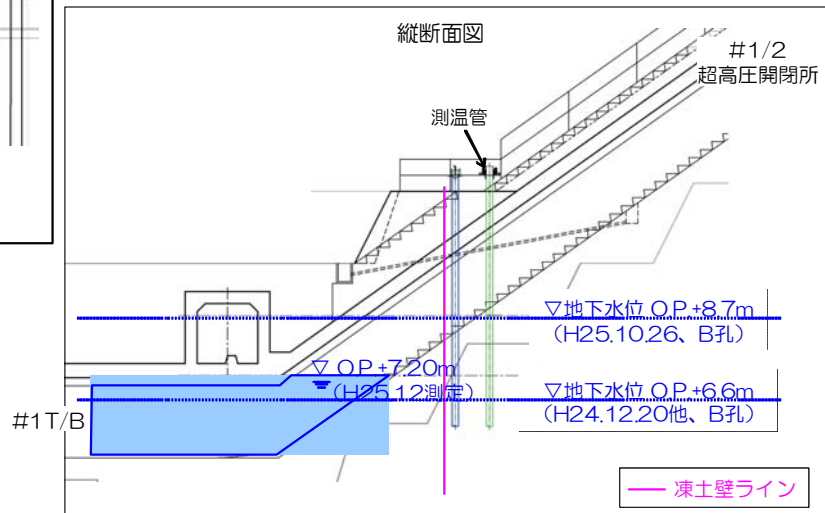
図14-7 【5-1】1号機電気ケーブルダクト 施工方法（貫通施工）
