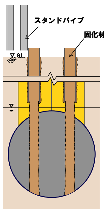
図3 頂版マルチステップ・底版内部充填工法（鉄管）の施工手順（2）
