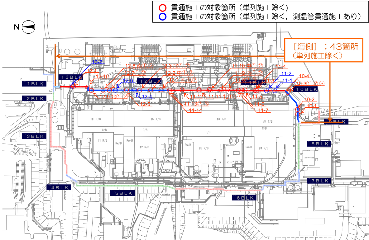
図4 貫通施工の対象箇所
