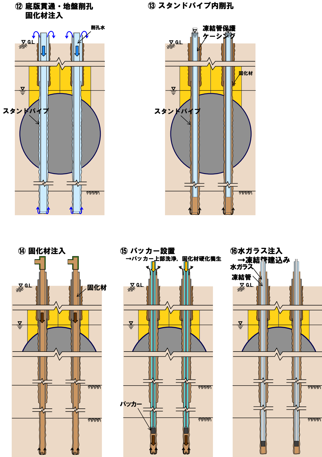
図3 頂版マルチステップ・底版内部充填工法の施工手順 (3)
