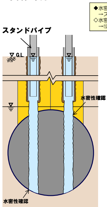
図3 頂版マルチステップ・底版内部充填工法（鉄管）の施工手順（2）
