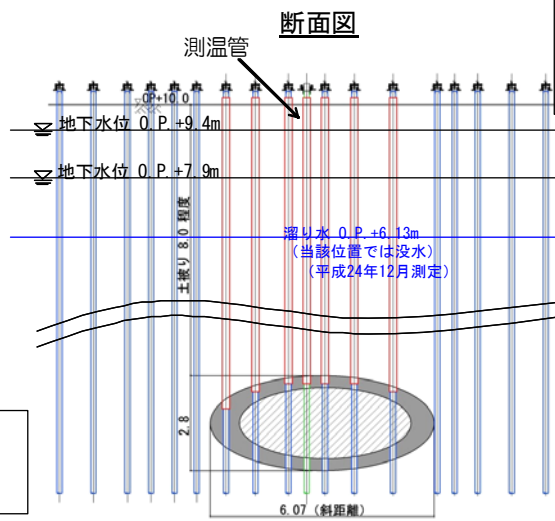
図14-19 【7-2】2~4号機DG連絡ダクト③ 施工方法（貫通施工）
