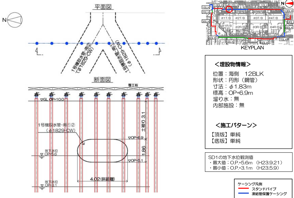
図5-26 【12-8】1号機取水管-南①② 施工方法（貫通施工）
