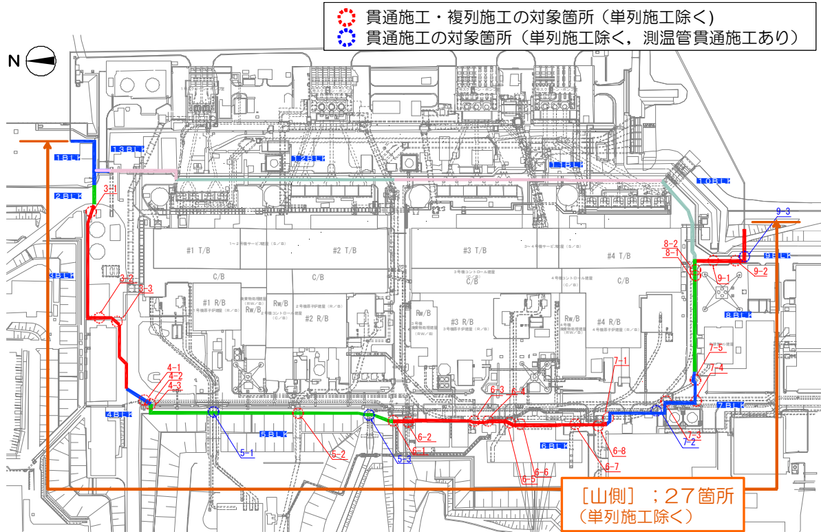
図13 貫通施工・複列施工の対象箇所
