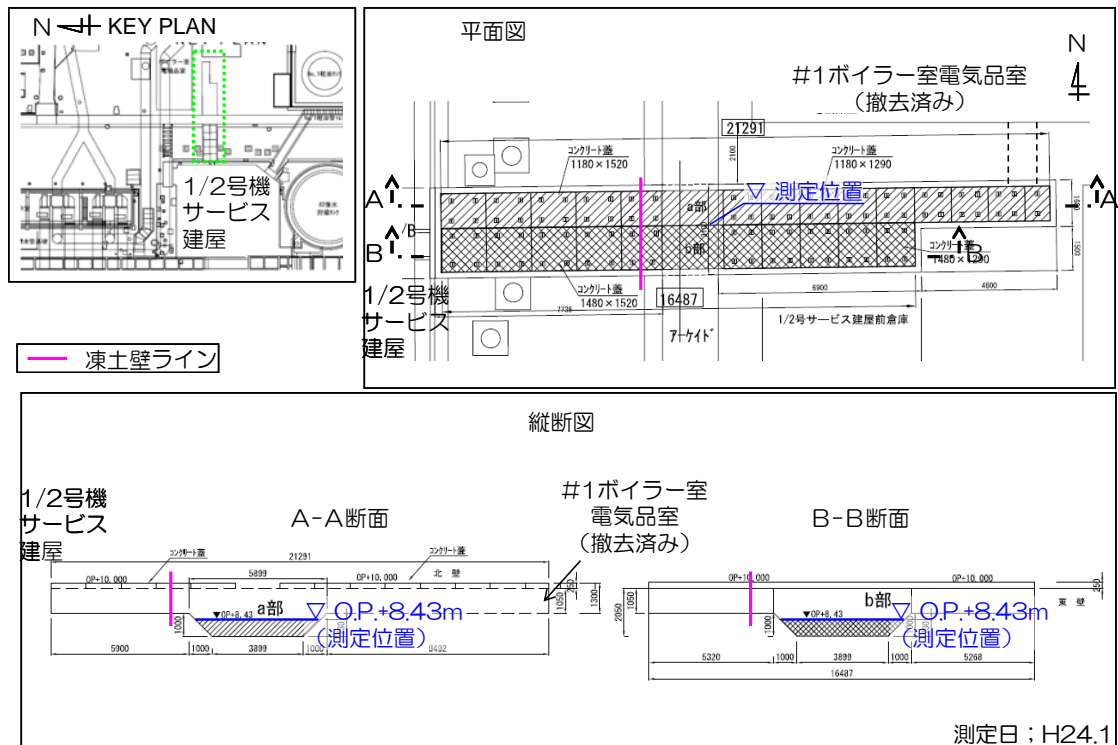
図5-24 【12-6】1号機ボイラー室電気品室連絡トレンチ 施工方法（貫通施工）
