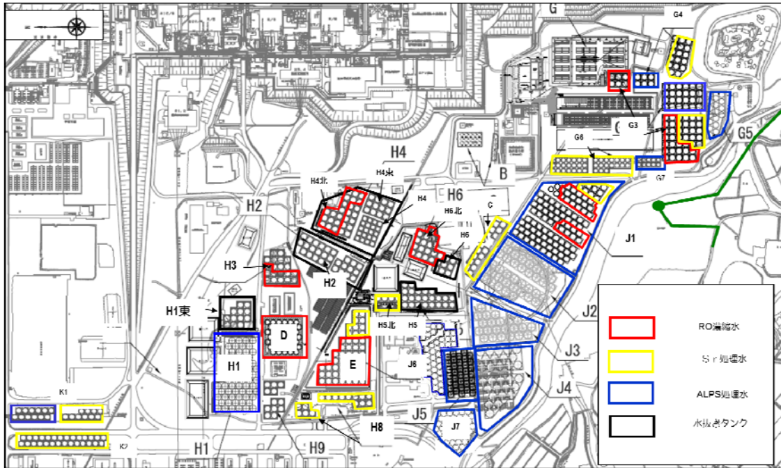
図1 タンクエリアの配置図
