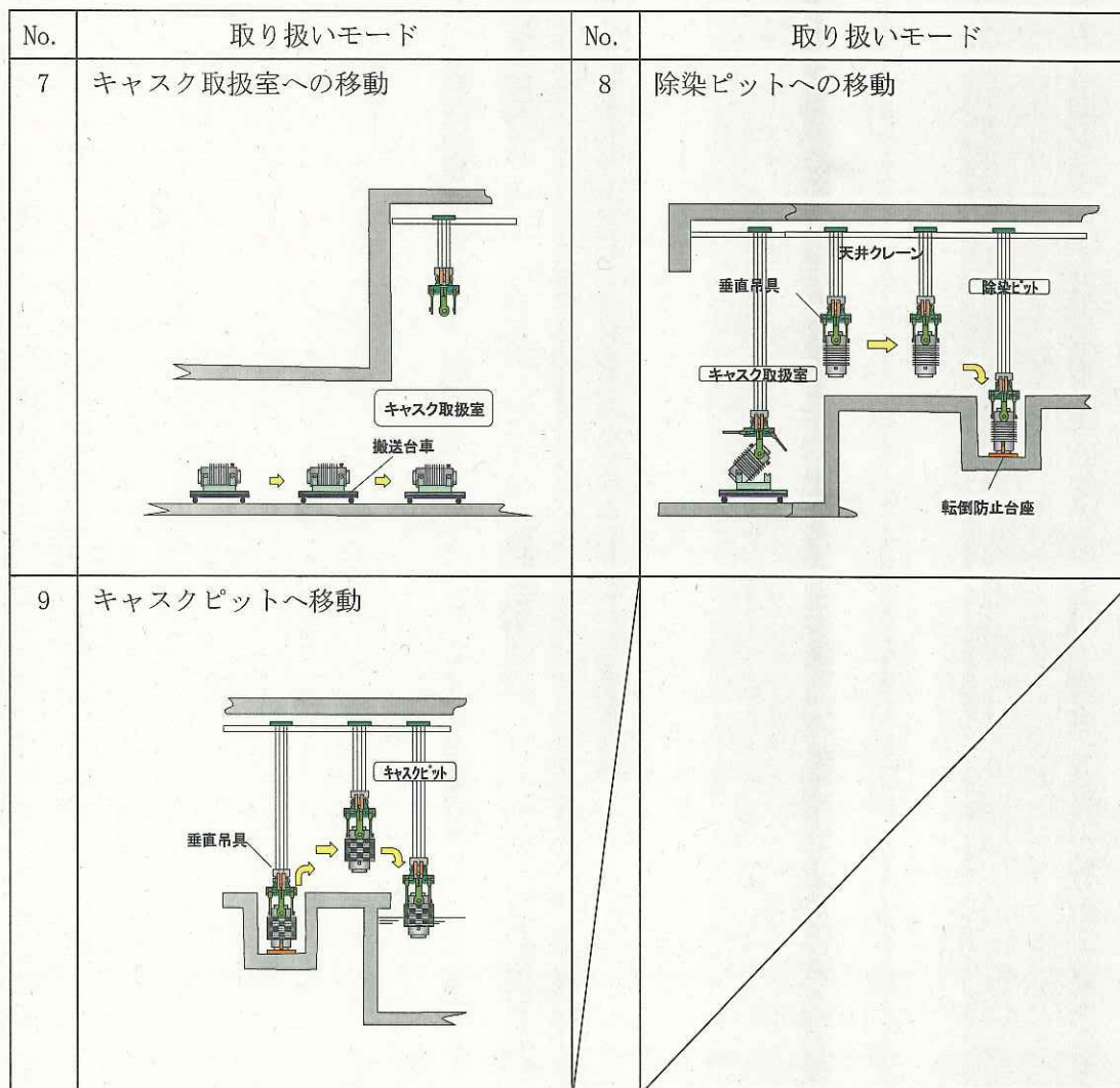
図ー２ 構内用輸送容器のハンドリングフロー (2/2)
