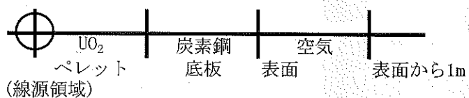
図一 1 8 漏えい燃料棒 2 本分のペレットに対する遮へい解析モデル
