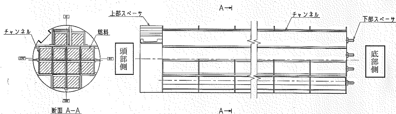
図－４ バスケットの応力評価箇所
