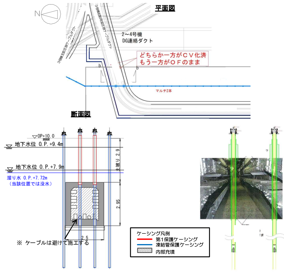
図 1 4 - 1 5 【 6 - 6 】 3号機起動用変圧器ケーブルダクト 施工方法（貫通施工）
