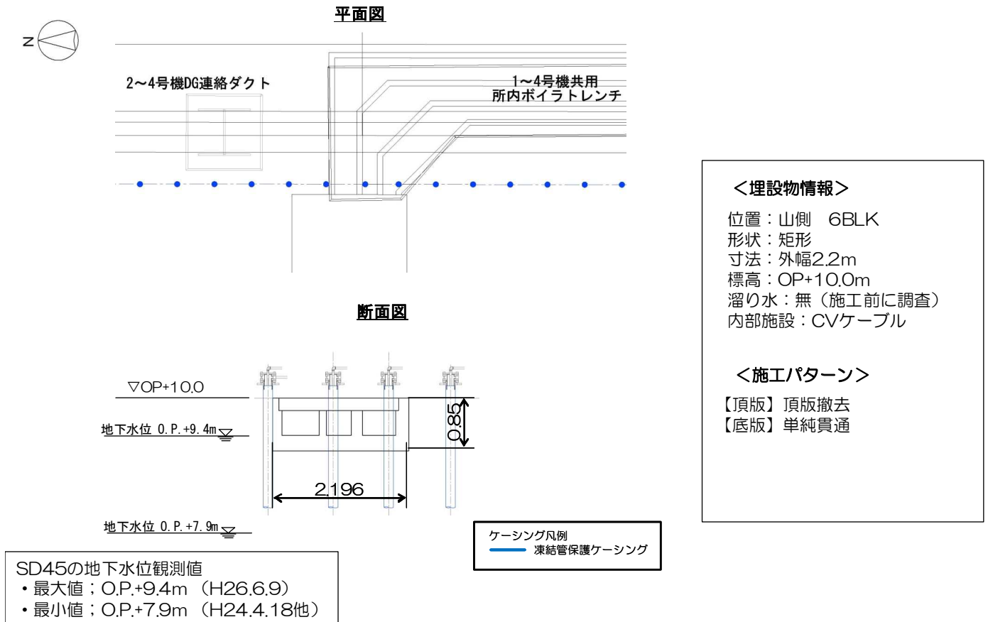
図 1 4 - 1 3 【 6 - 4 】 1 ~ 4 号機共用所内ボイラトレンチ 施工方法（貫通施工）
