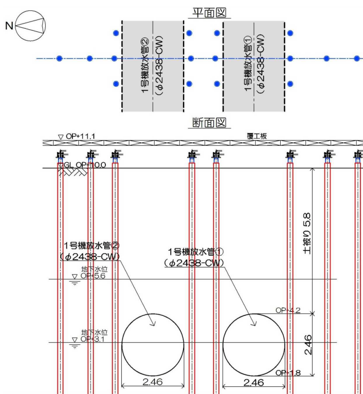
図 3 - 2 5 【 1 2 - 7 】 1号機放水管①② 施工方法（複列施工）
