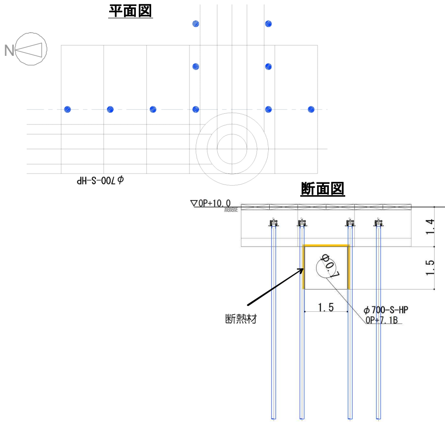
図 1 4 - 2 5 【 9 - 1 】 排水ヒューム管③ 施工方法 (複列施工)
