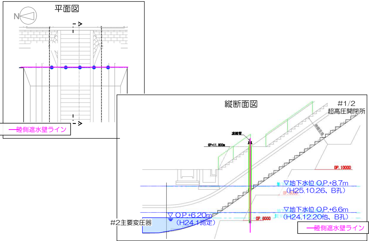
図14-8 【5-2】2号機主変圧器ケーブルダクト 施工方法（貫通施工）
