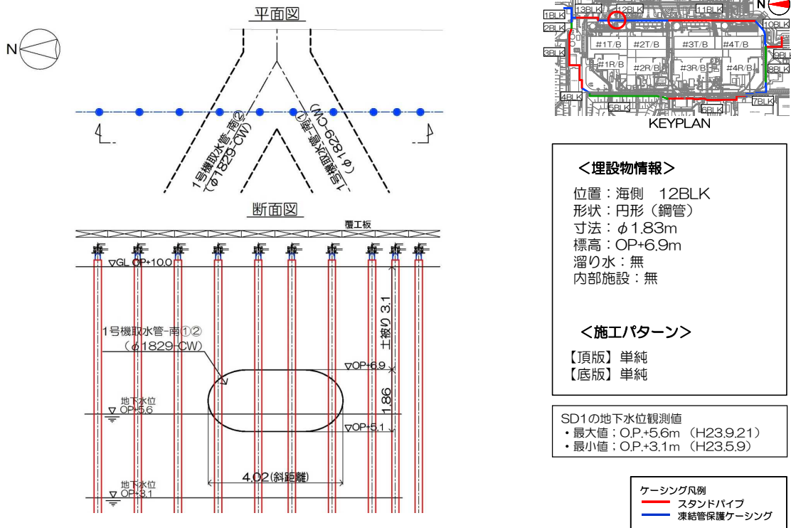
図 3-26 【12-8】1号機取水-南①② 施工方法（貫通施工）
