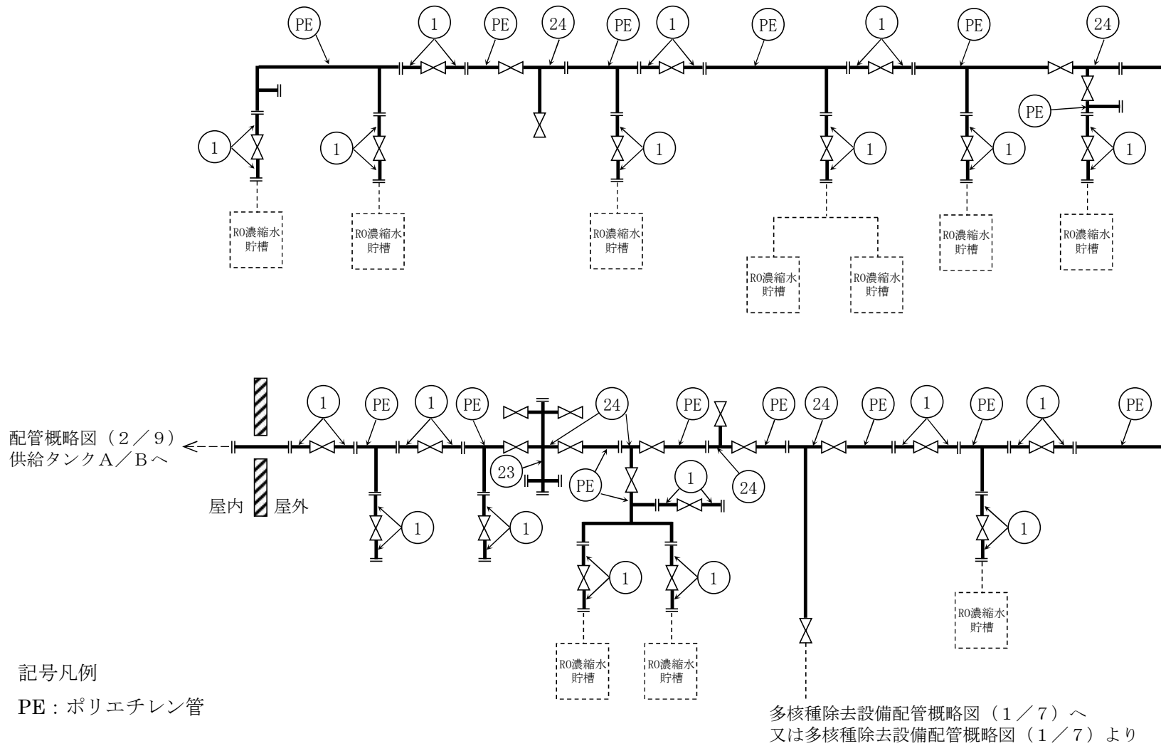
図-4 配管概略図 (1/9)
