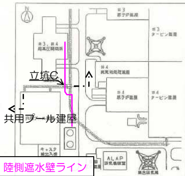
平面図 KEY PLAN
