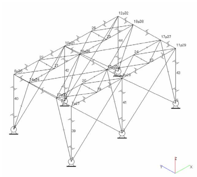
図-5 ディスクフィルタ解析モデル
