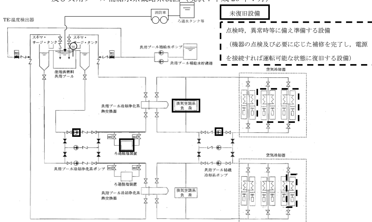
図 1-1 共用プール冷却浄化系，共用プール補機冷却系 及び共用プール補給水系概略系統図（現状：平成 26 年 7 月）
