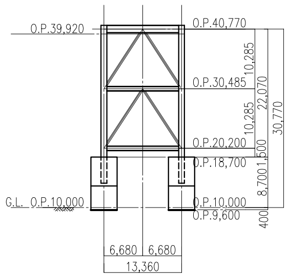
(b) 立面図
