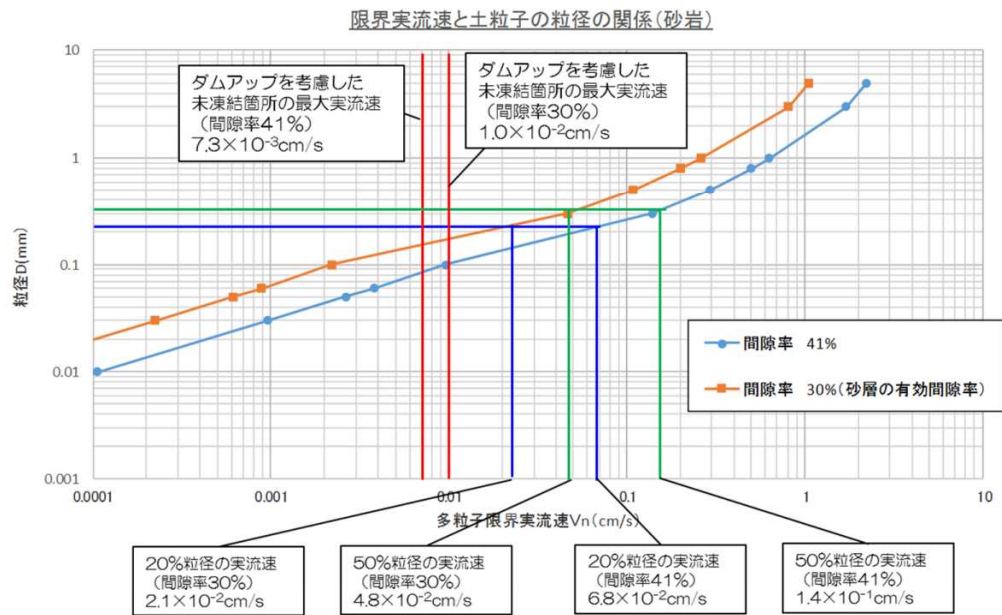
図-10 限界実流速と土粒子の粒径の関係と想定最大実流速
