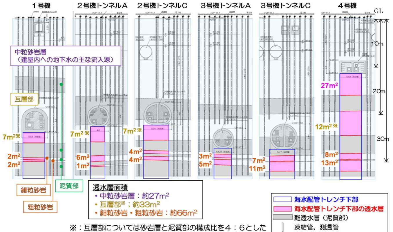
図一 2 海水配管トレンチ下部の非凍結範囲（詳細）
