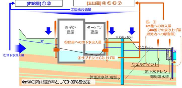
図-3 陸側遮水壁 (海側) のみ閉合した場合の地下水収支想定
