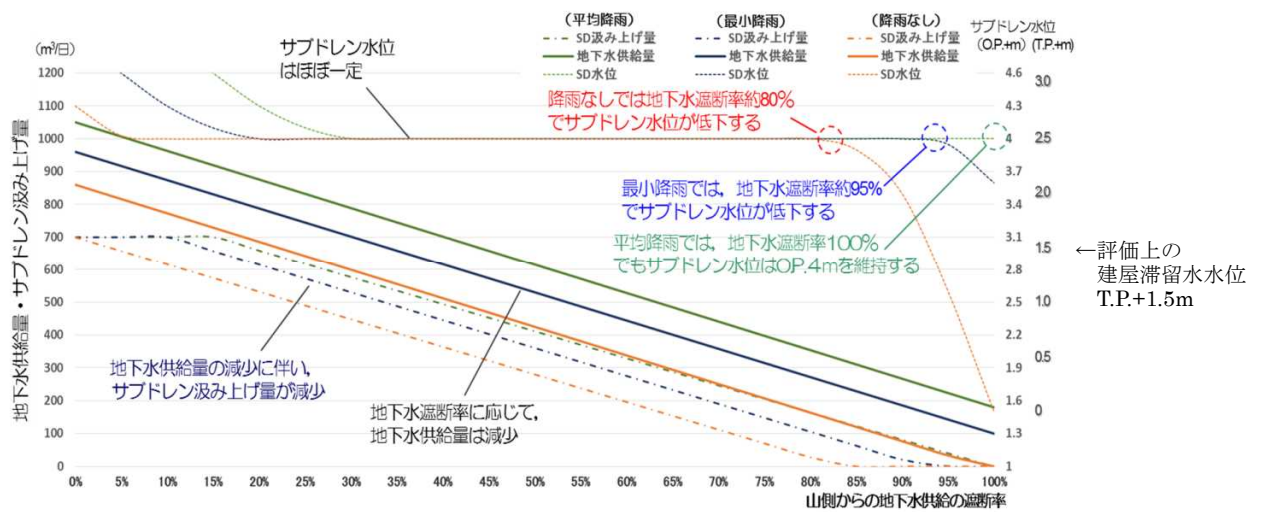
図－2 地下水遮断率 ※2 とサブドレン汲み上げ量 建屋周辺地下水位（サブドレン水位）の関係
