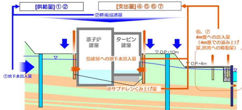
図－3 山側からの地下水流入の遮断率に応じた地下水収支イメージ
