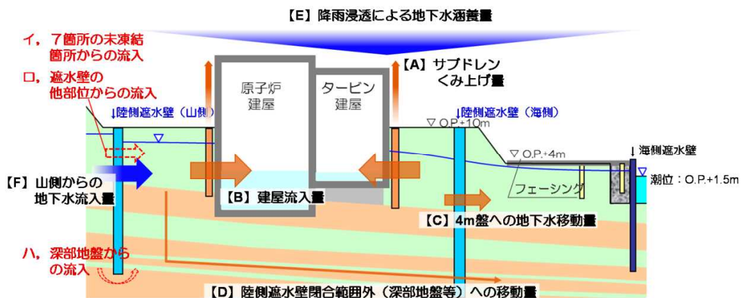
図-1 陸側遮水壁閉合範囲の地下水収支
