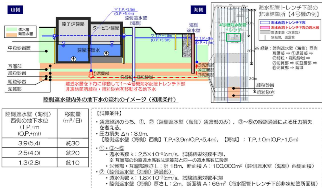
図-5 海水配管トレンチ下部非凍結箇所を通じた地下水移動量の想定 (細粒・粗粒砂岩)
