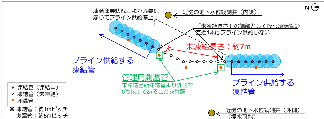
図-15 未凍結長さの管理図（例：西側③）
