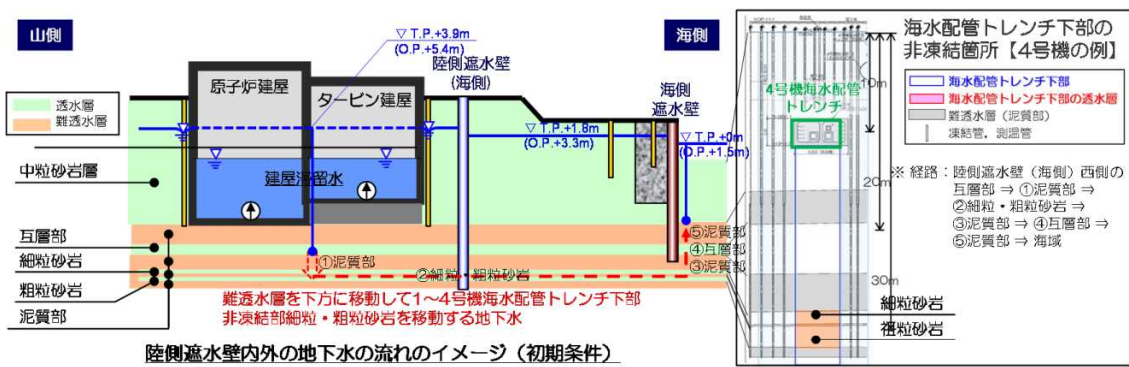
図-4 海水配管トレンチ下部の非凍結箇所を通じた地下水移動量の想定 (第一段階フェーズ1 中粒砂岩層)
