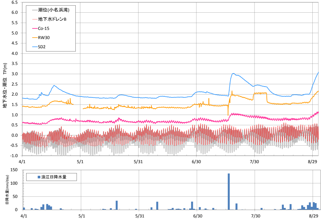
図ー 7 地下水ドレンBライン上の地下水位の経時変化
