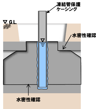
図9 頂版撤去・底版内部充填工法の施工手順
