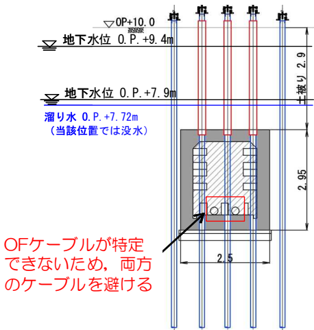
図16-15 【6-6】3号機起動用変圧器ケーブルダクト 施工方法（貫通施工）
