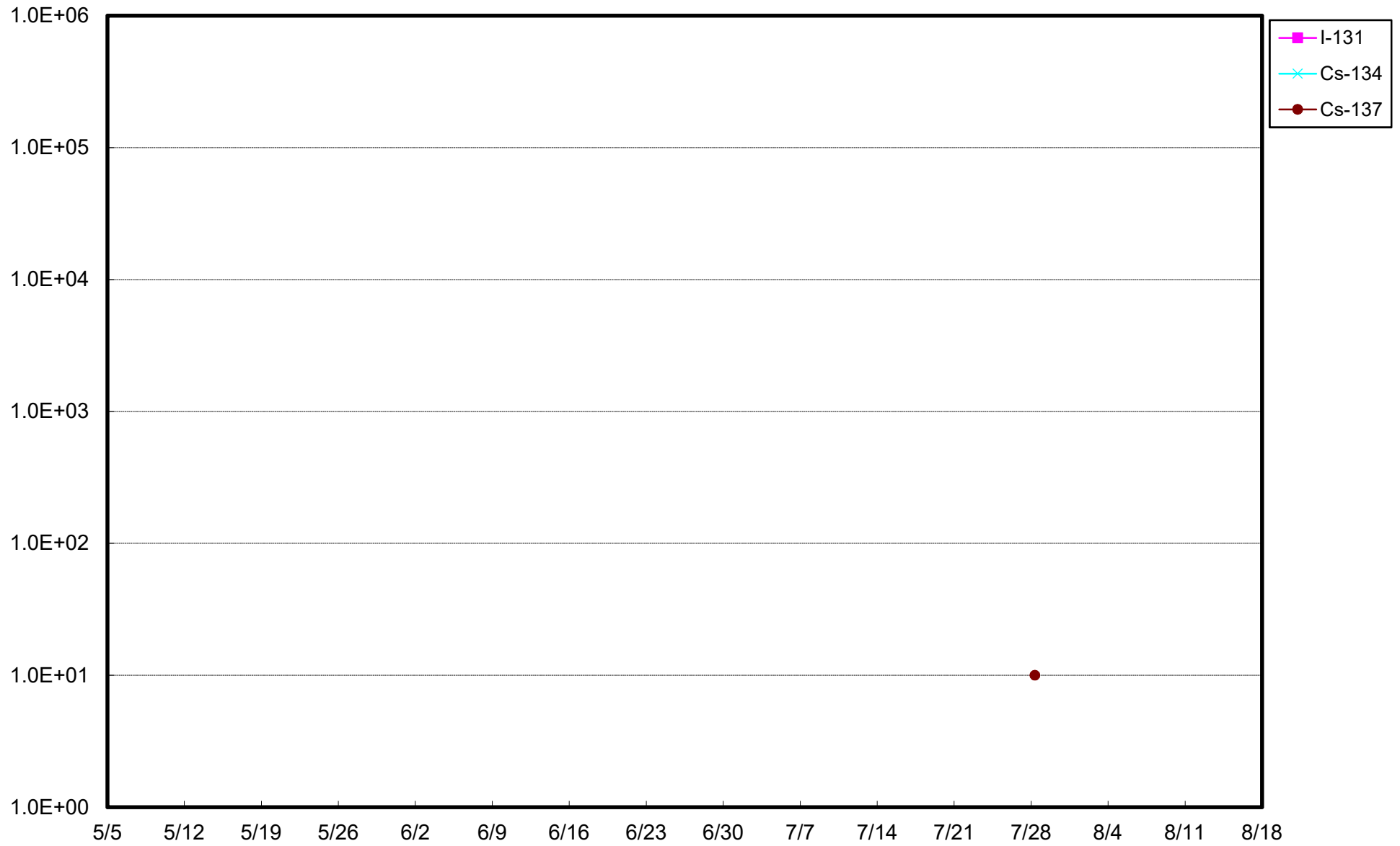
福島第一 4号機サブドレン放射能濃度 (Bq/L)
