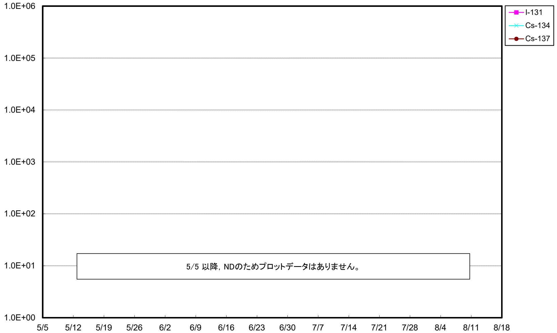
福島第一 3号機サブドレン放射能濃度(Bq/L)
