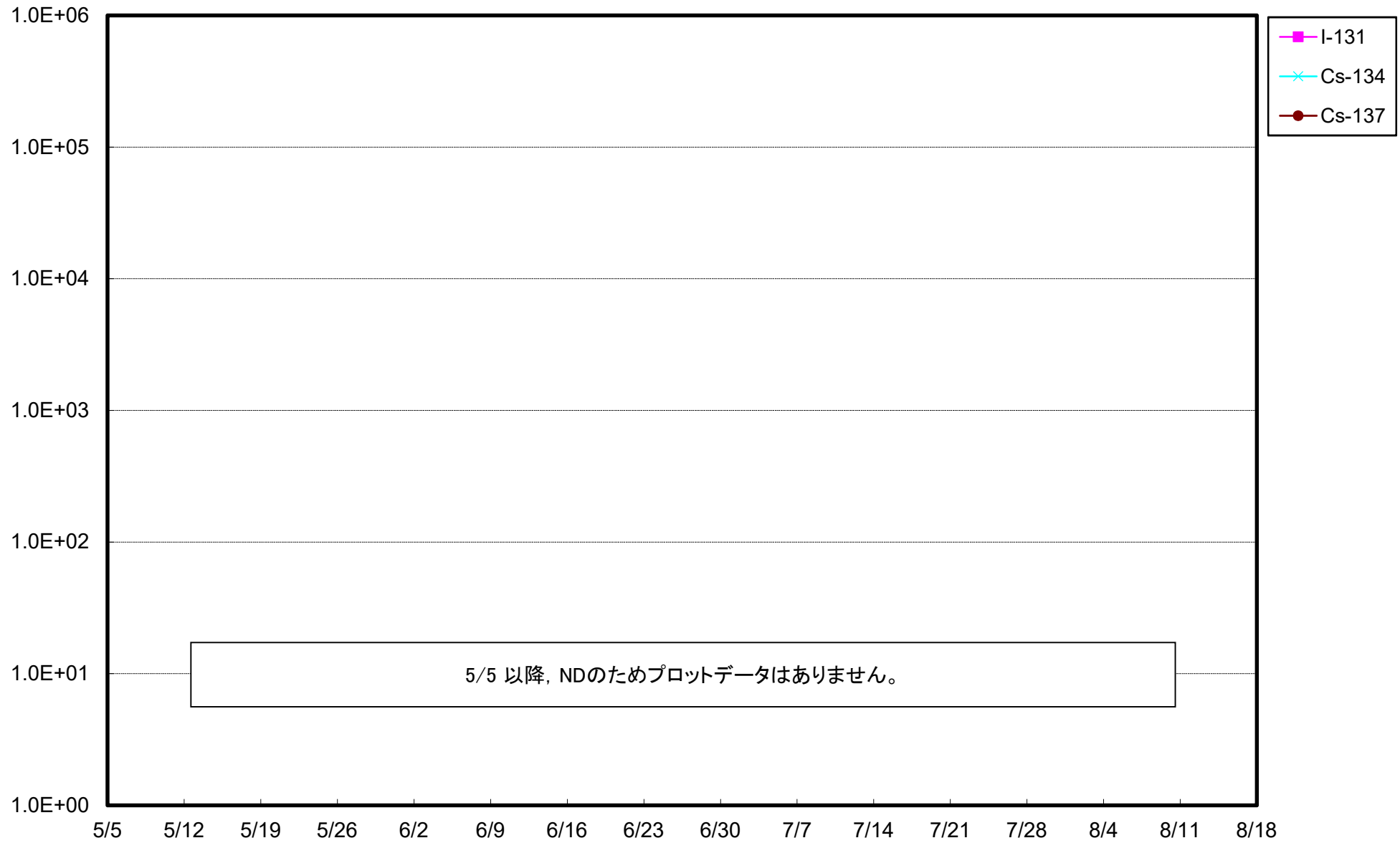
福島第一 5号機サブドレン放射能濃度(Bq/L)
