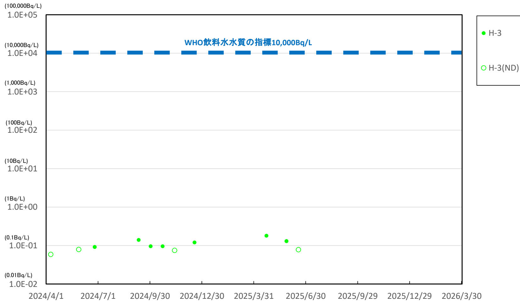
小高区沖合15km付近(T-B1) 表層 海水放射能濃度
