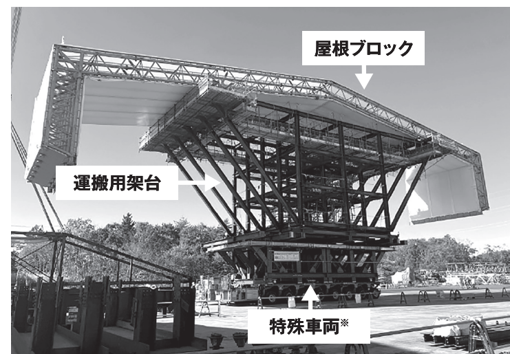
可動屋根を特殊車両に積載している様子
