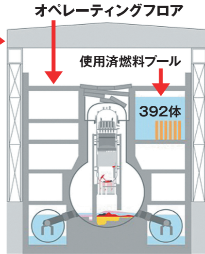
1号機原子炉建屋 縦断面図
