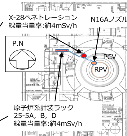
2号機R/B2階
