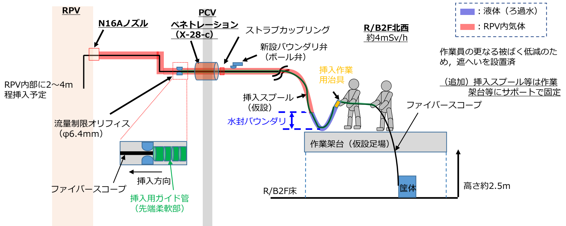
RPV内部調査方法のイメージ
