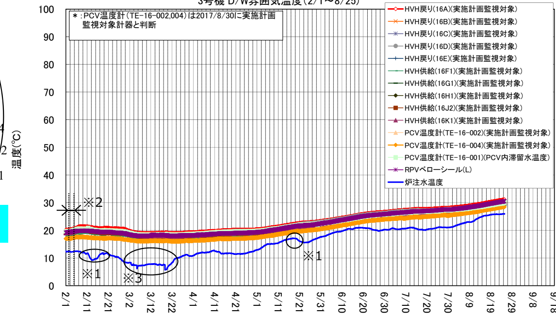
3号機 D/W雰囲気温度 (2/1~8/25)
