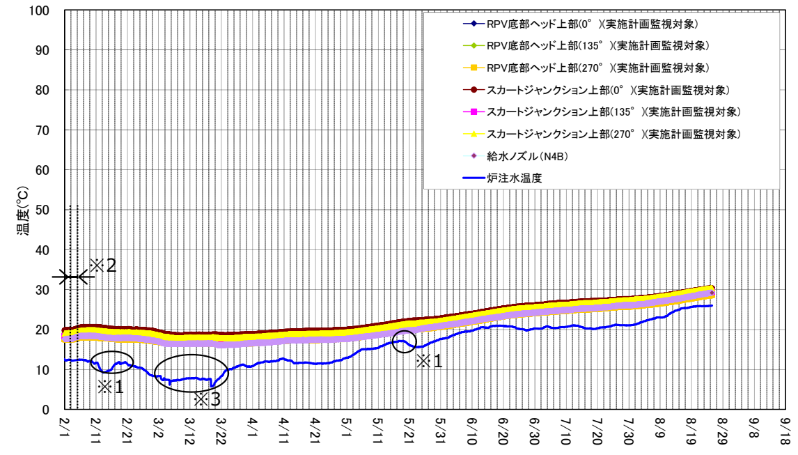
3号機 原子炉压力容器まわり温度 (2/1~8/25)
